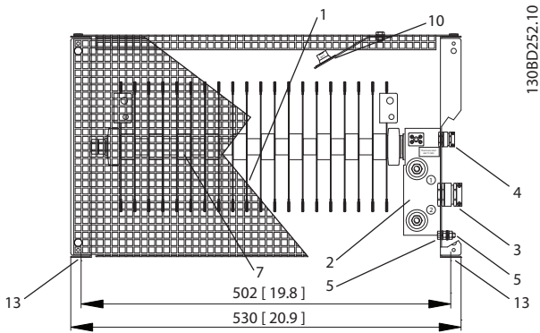
Abbildung 9.45 IP20, Vorderansicht
