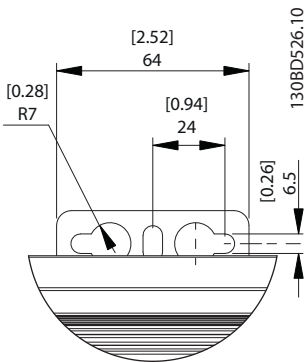
Abbildung 9.9 Bohrung
