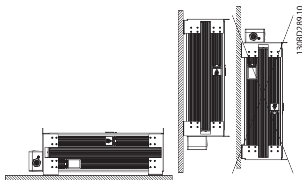
Abbildung 9.90 Aufstellung
