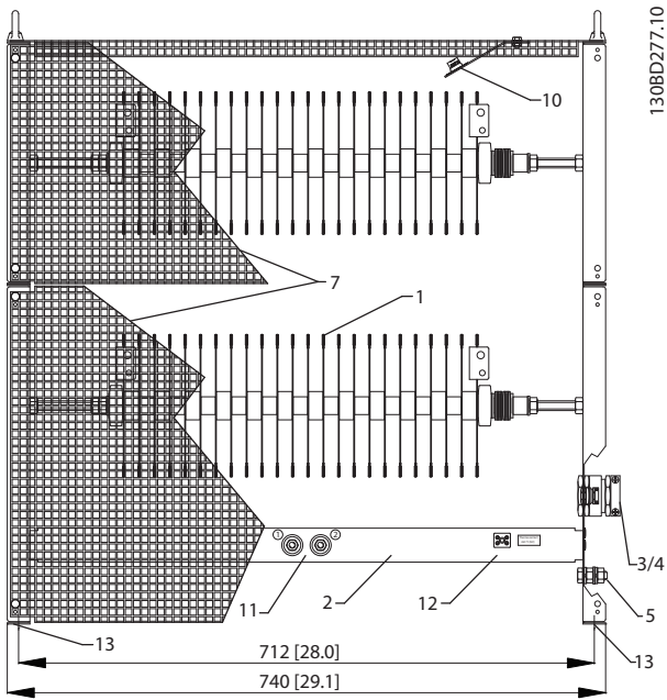
Abbildung 9.70 IP20, Vorderansicht
