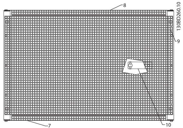
Abbildung 9.53 IP20, Ansicht von oben
