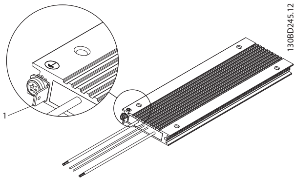
Abbildung 2.3 Flatpack IP54
