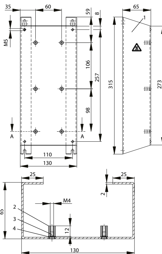
Abbildung 9.116 Auflagehalterung 175U0086
