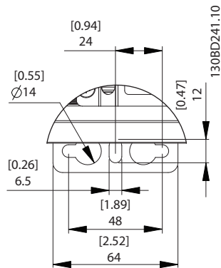
Abbildung 9.3 Bohrung
