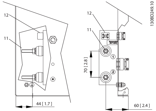
Abbildung 9.57 Anschlüsse
