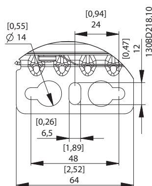
Abbildung 9.31 Bohrung
