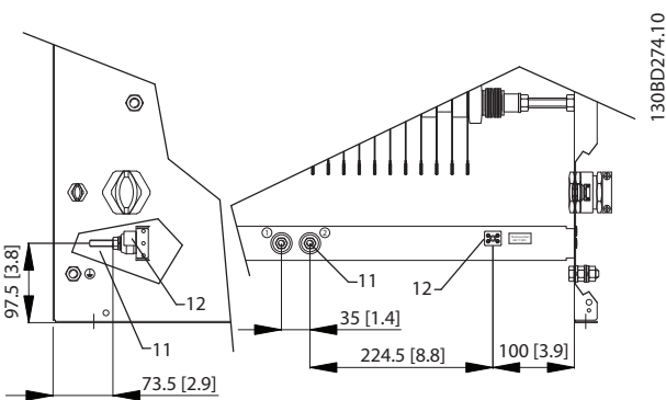
Abbildung 9.72 Anschlüsse
