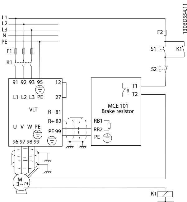
Abbildung 3.19 Der Temperaturschalter in Motor und Bremswiderstand schaltet die Netzversorgung durch einen Eingangsschütz ab
