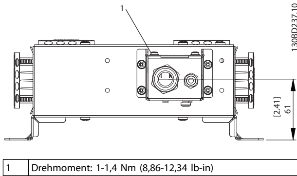
Abbildung 9.2 IP21, Ansicht von unten, Verteilerbox
