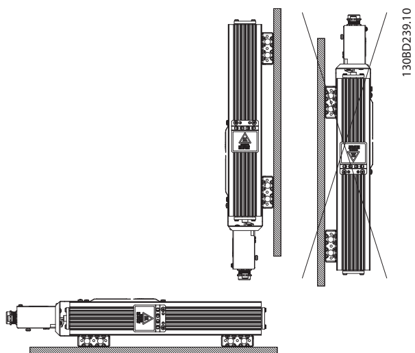
Abbildung 9.6 Aufstellung
