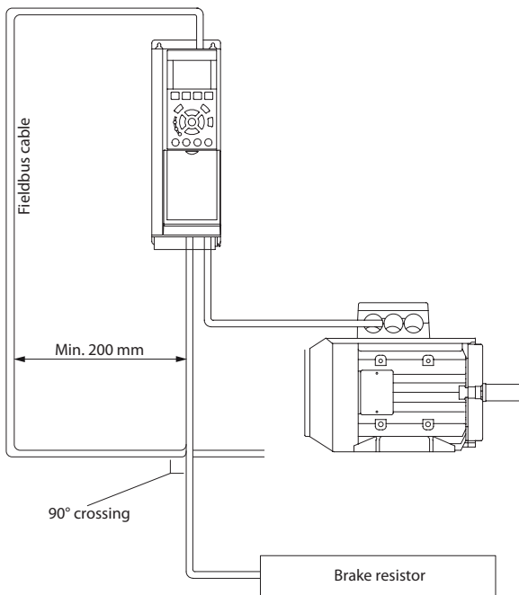
Abbildung 3.15 Kabelführung
