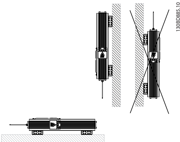
Abbildung 9.11 Aufstellung
