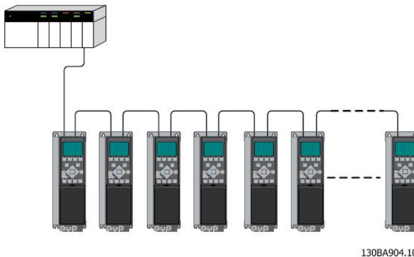
Ilustración 3.3: Topología en línea
