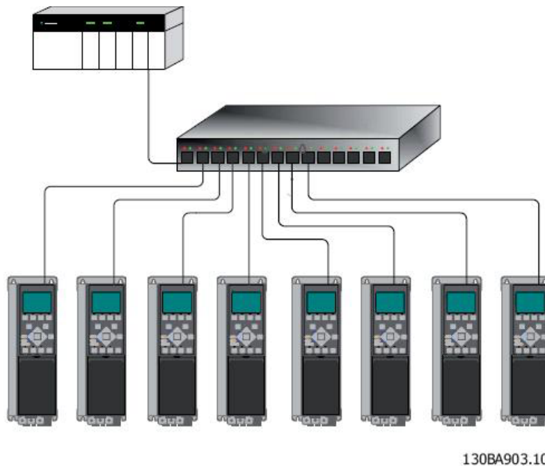
Ilustración 3.2: Topología en estrella
