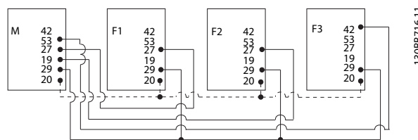
Illustration 6.4 Connexion des fils de commande des unités esclaves F1-F3 au maître M
