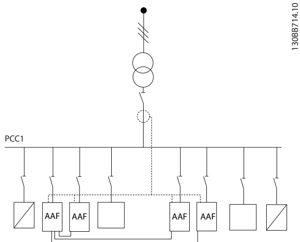
Illustration 6.2 4 AAF en maître/esclave
