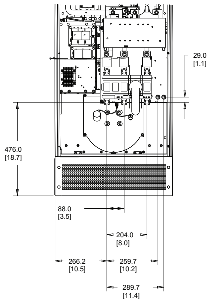
Illustration 3.6 Emplacement des bornes sur le D14 avec sectionneur
