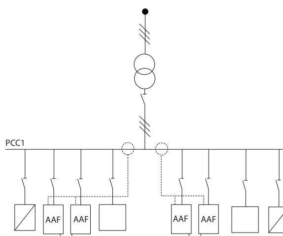
Illustration 6.1 Deux ensembles d'AAF en maître/esclave
