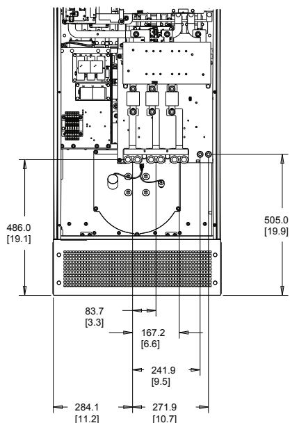
Рисунок 3.7 Расположение клемм в корпусе D14 без разъединителя
