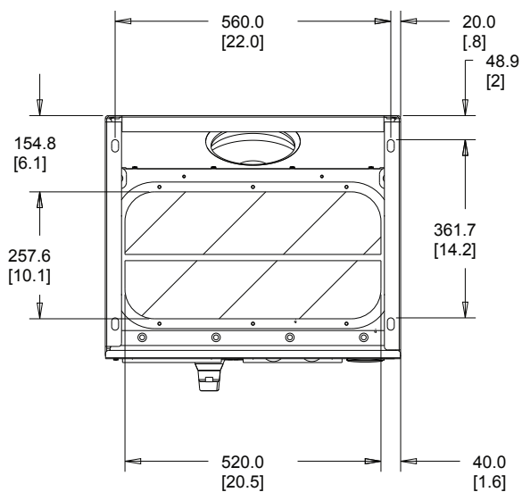
Рисунок 3.13 Корпус E1, вид снизу
