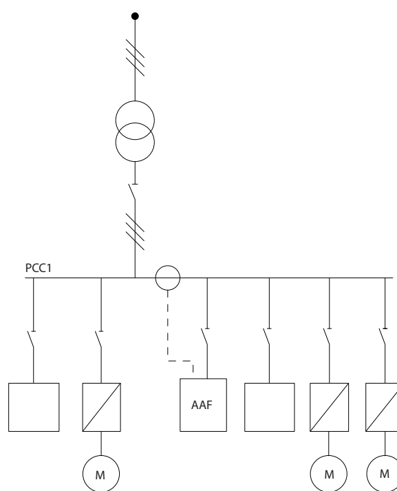
Рисунок 4.9 Трансформаторы тока, установленные со стороны источника (PCC), для групповой компенсации.
