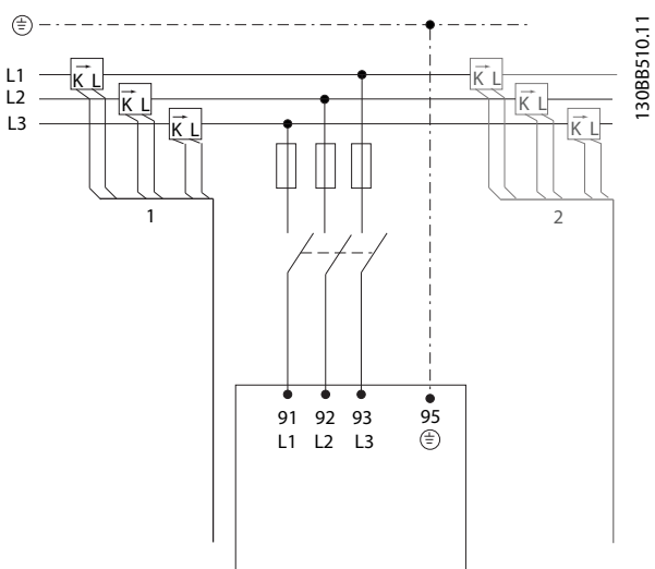
图 2.4 外部 CT 的接线
