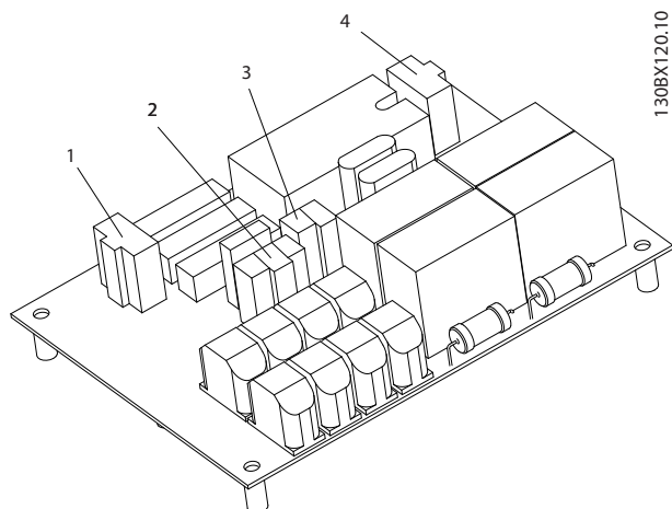
图 6.4 软充电卡连接器
