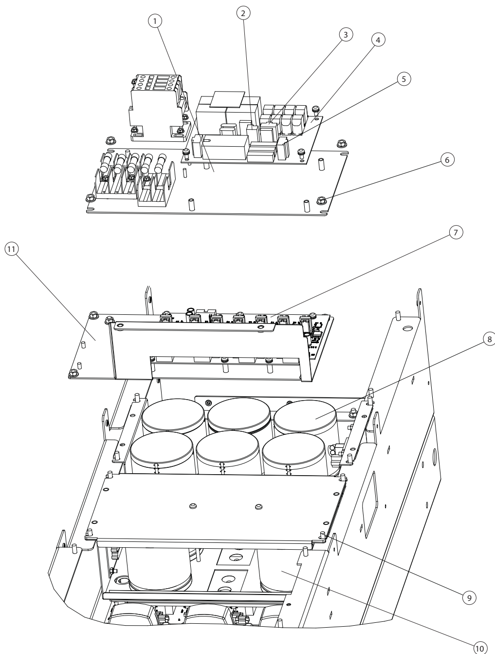
图 8.3 软充电卡、门驱动器卡、电容器组
