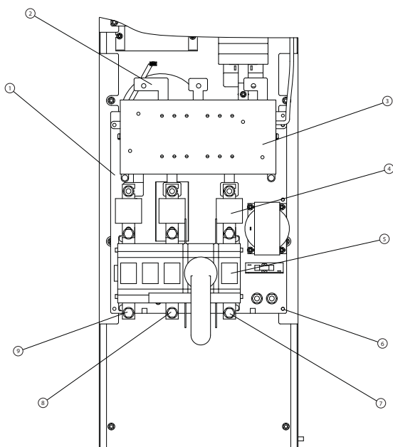
图 7.5 输入端子固定板
