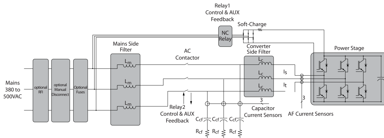
图 3.1 AAF 内部电路
