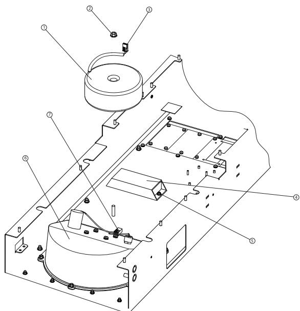
图 7.7 软充电电阻器、风扇变压器和散热片风扇单元
