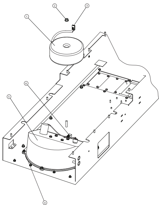
图 8.8 风扇变压器和散热片风扇单元
