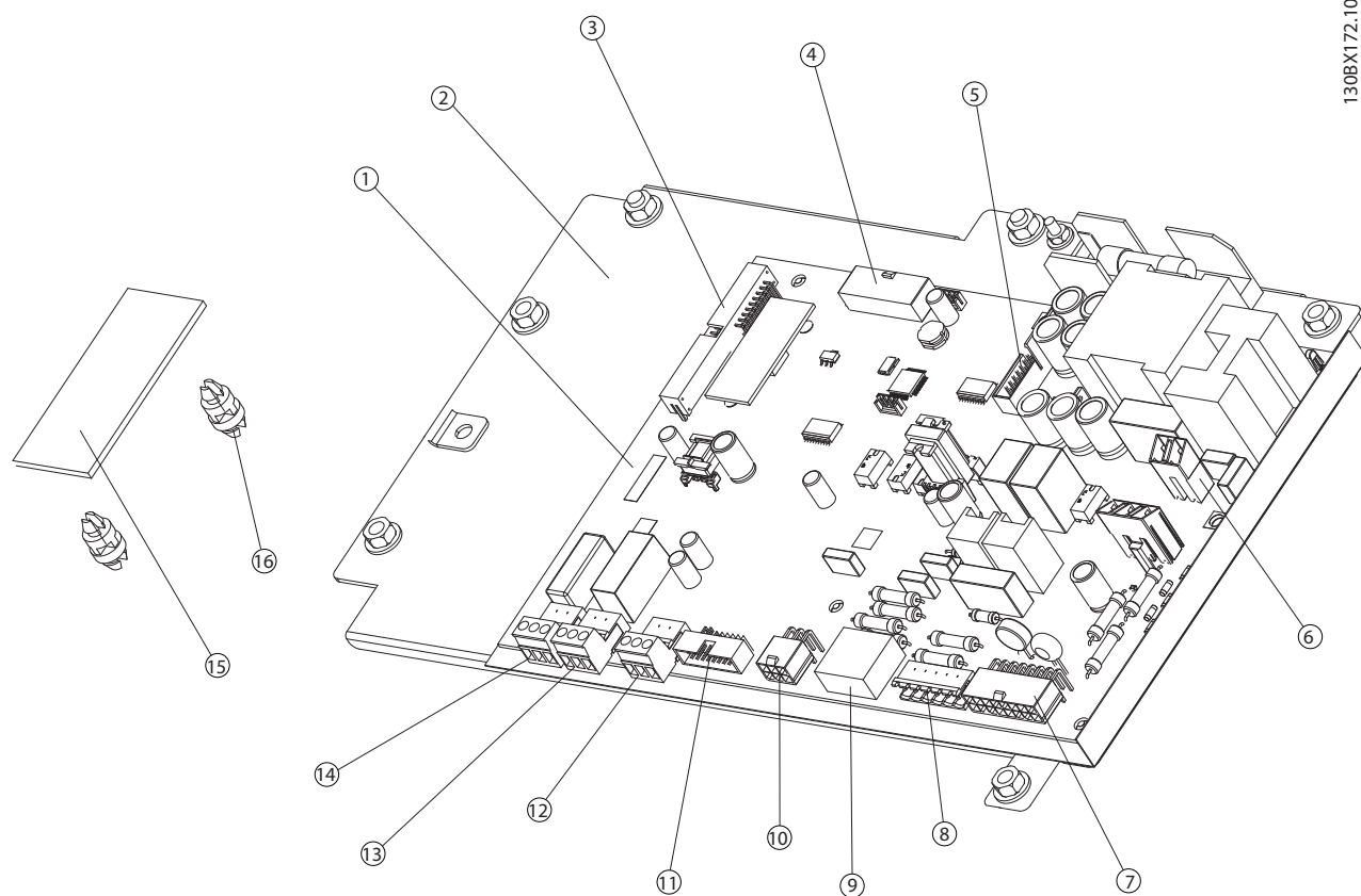
图 7.2 功率卡端子和标定卡
