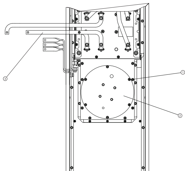
图 8.9 散热片风扇单元
