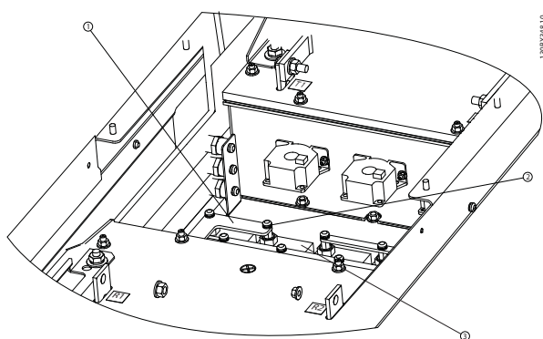
图 8.11 阻尼电阻器
