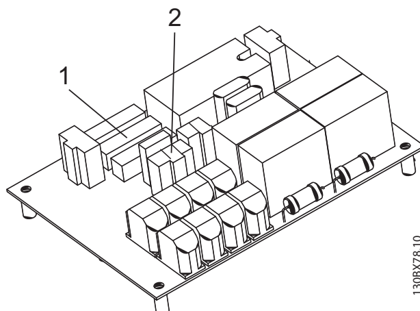
图 6.3 软充电卡的熔断器位置
