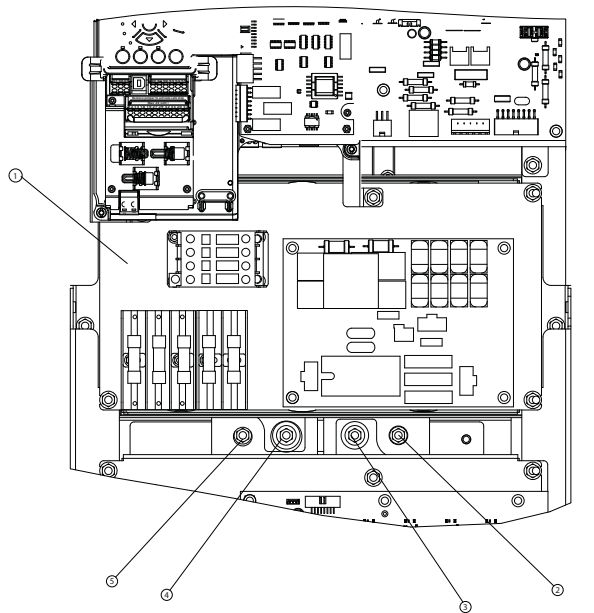
图 8.5 直流电容器组检视
