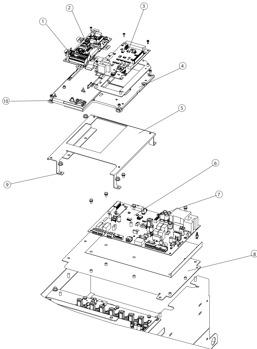
图 8.1 控制卡、有源滤波器卡和功率卡固定
