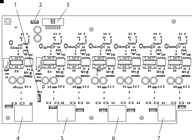
图 8.4 门驱动器卡
