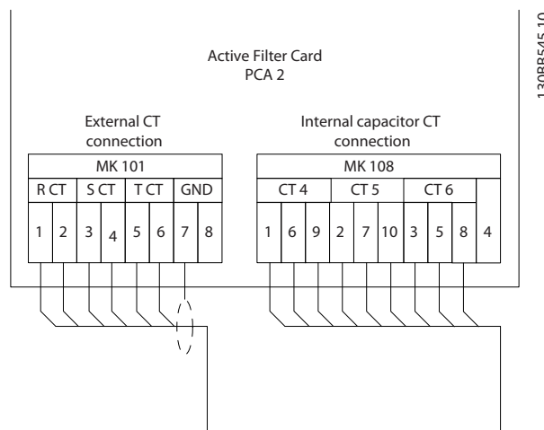
图 2.2 AFC 连接器 MK101 和 MK108
