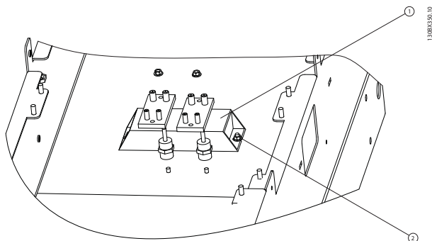
图 8.6 软充电电阻器
