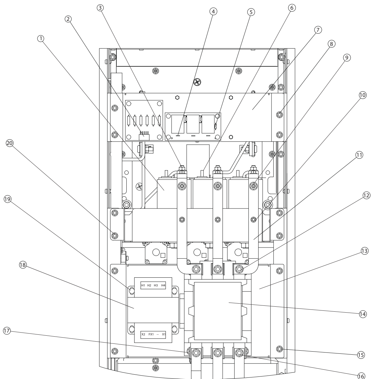
图 8.10 交流输入接触器、变压器、固定板、交流电容器组和射频干扰滤波器板
