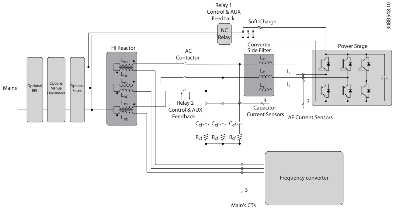
图 3.3 LHD 内部电路
