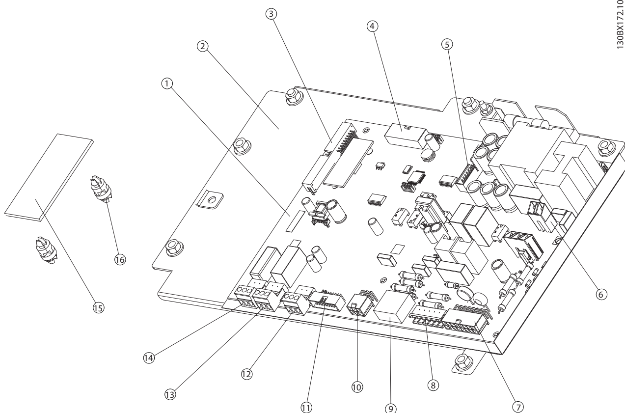
图 8.2 功率卡端子和标定卡
