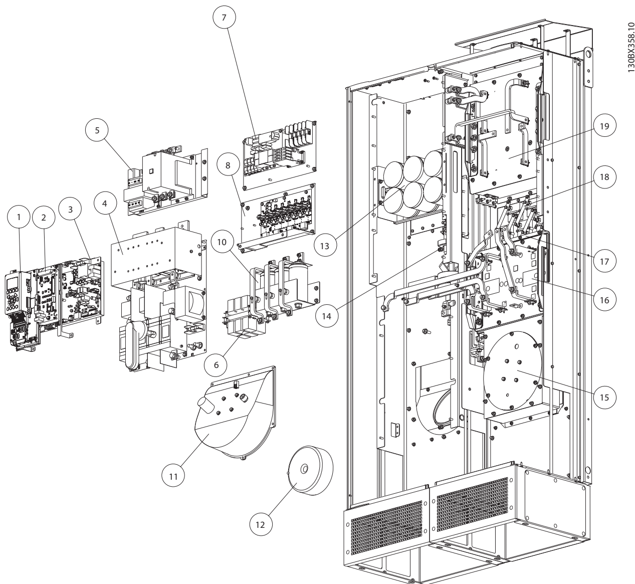
图 1.1 AAF005 分解图 (D 机架)
