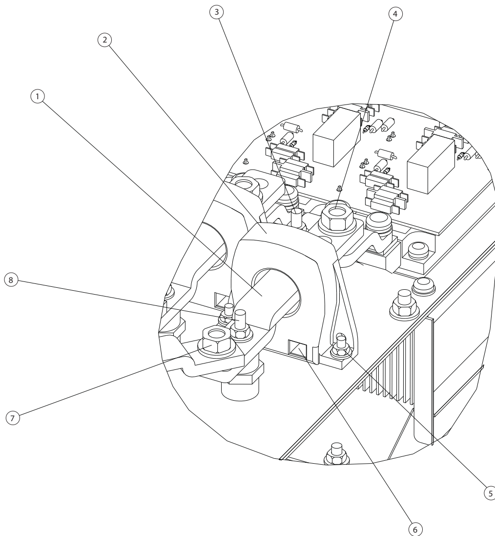
图 7.6 IGBT 电流传感器
