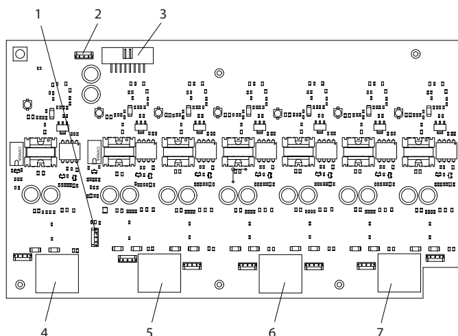
图 7.3 门驱动器卡
