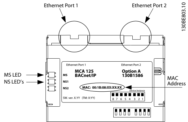
Abbildung 7.1 Übersicht über die BACnet/IP-Schnittstelle
