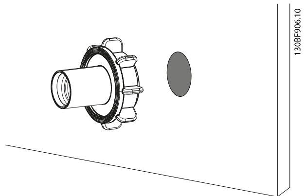
Abbildung 1.5 Die Mutter, gedreht um 180°, für dünne Wände
