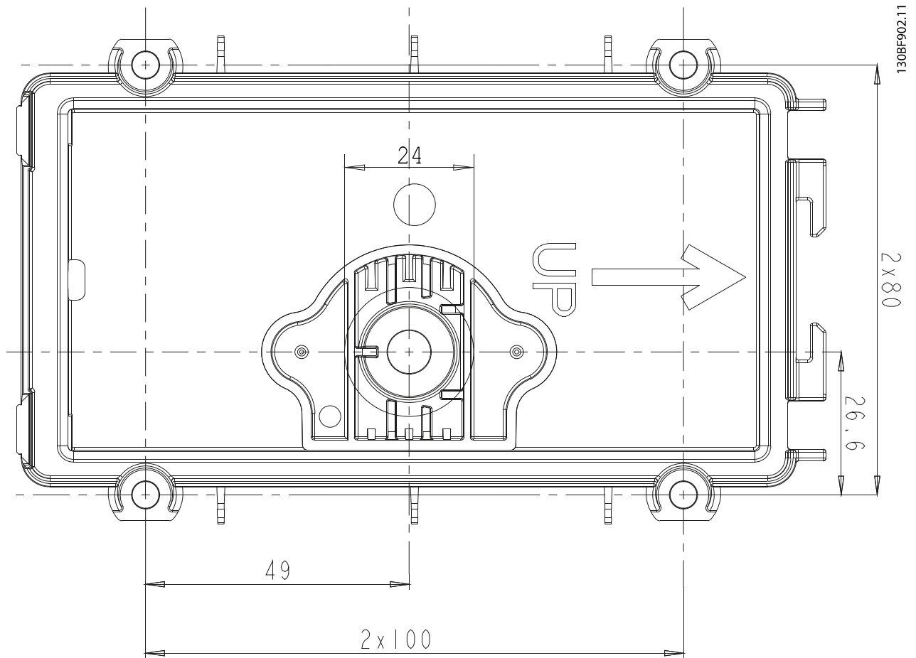
Abbildung 1.16 Bohrschablone, Maßstab 1:1
