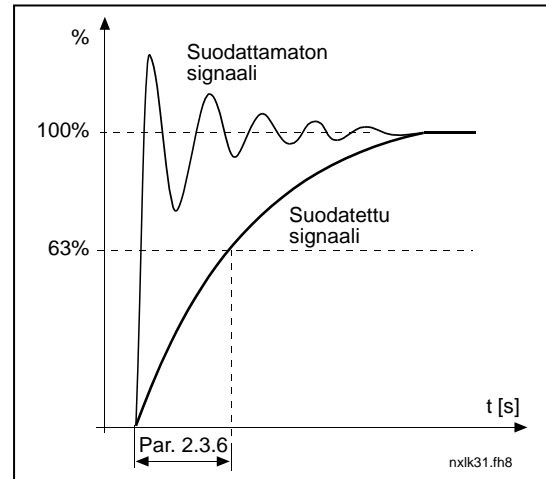
Kuva 1-5. Analogialähdön suodatusaika
