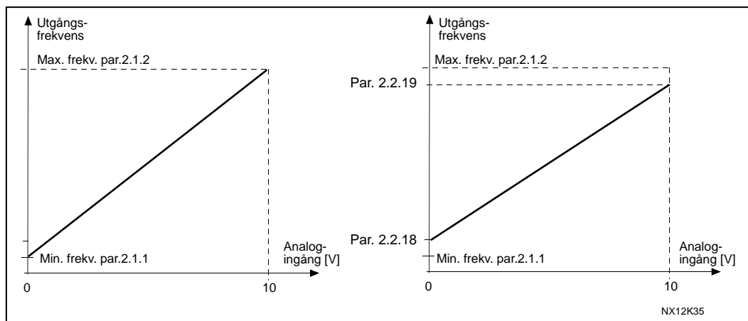
Figur 1- 4. Vänster: Par 2.1.18=0 (Ingen referensskalning) Höger: Referensskalning
