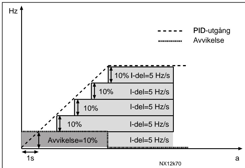
Figur 1- 24. PID-regulatorns funktion som I-regulator.
