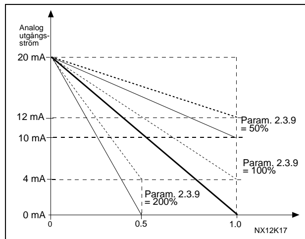
Figur 1- 6. Invertering av analog utgång
