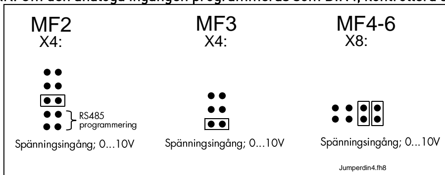
Figur 1- 1. Byglingsalternativ på X4/X8 då AI1 fungerar som DIN4
