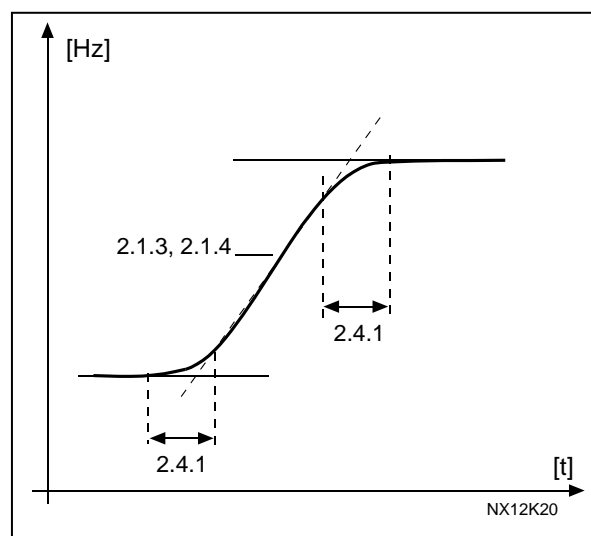
Figuur 1- 10. Acceleratie/Deceleratie (S-curve)
