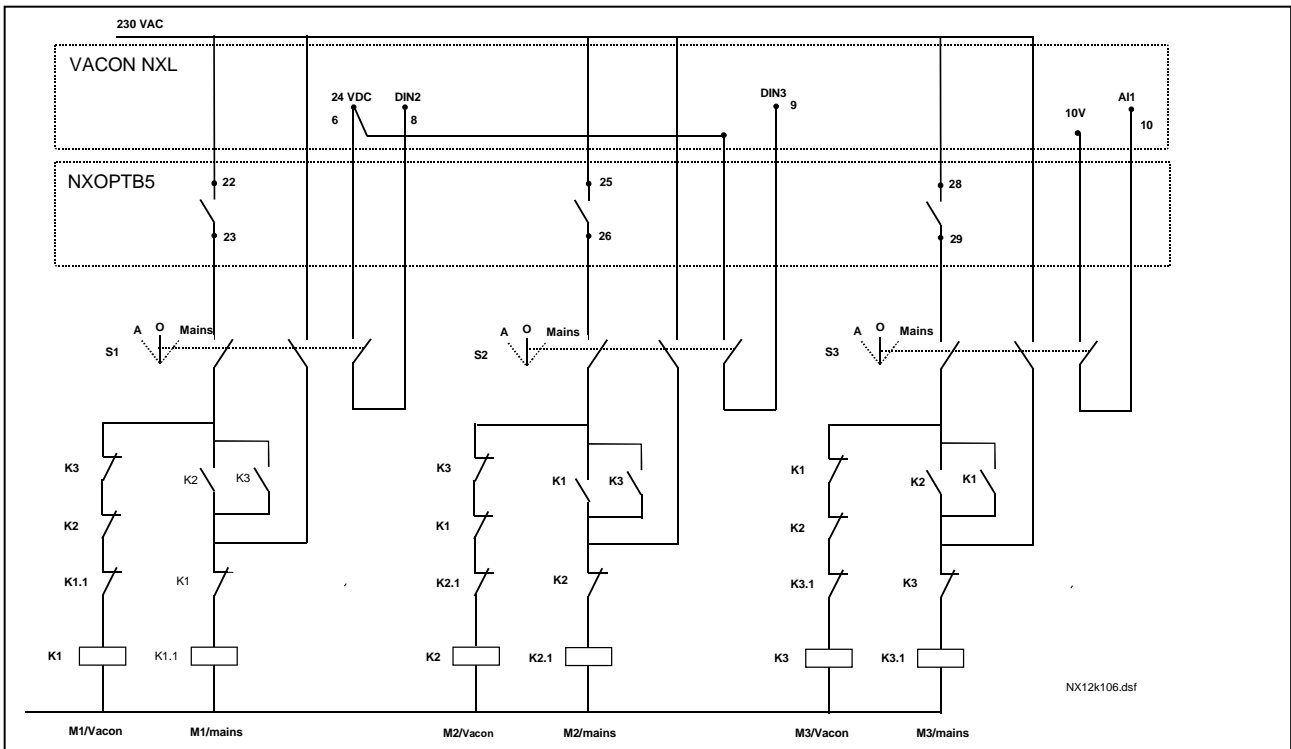
Figuur 1- 31. 3-pomp autowissel systeem, principe stroom diagram
