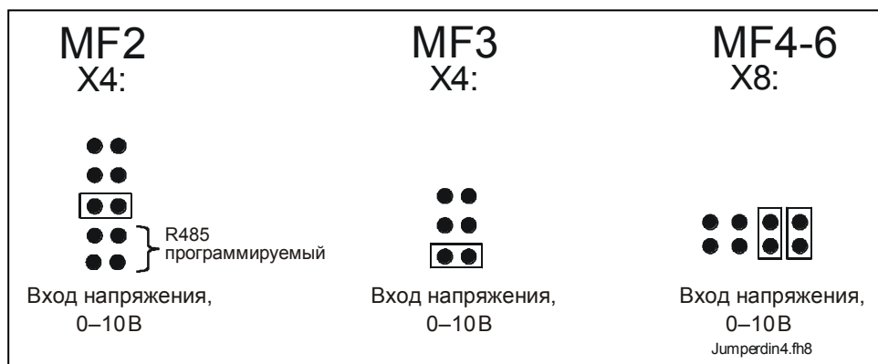
Рис. 1-1. Расположение перемычек X4/X8, когда AI1 функционирует как DIN4
