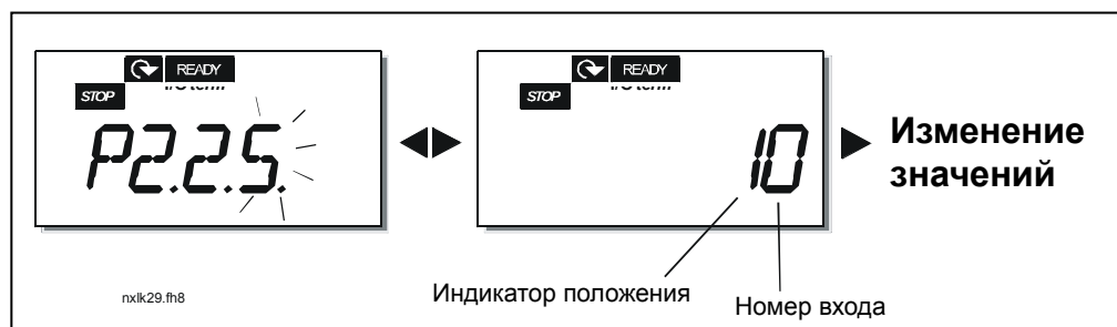
Рис. 1-2. Выбор сигнала AI1
