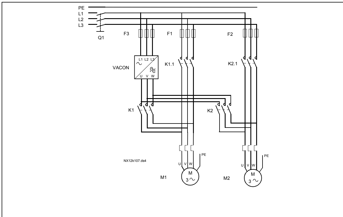
Рис. 1-34. Пример автозамены среди 2 насосов, силовая схема
