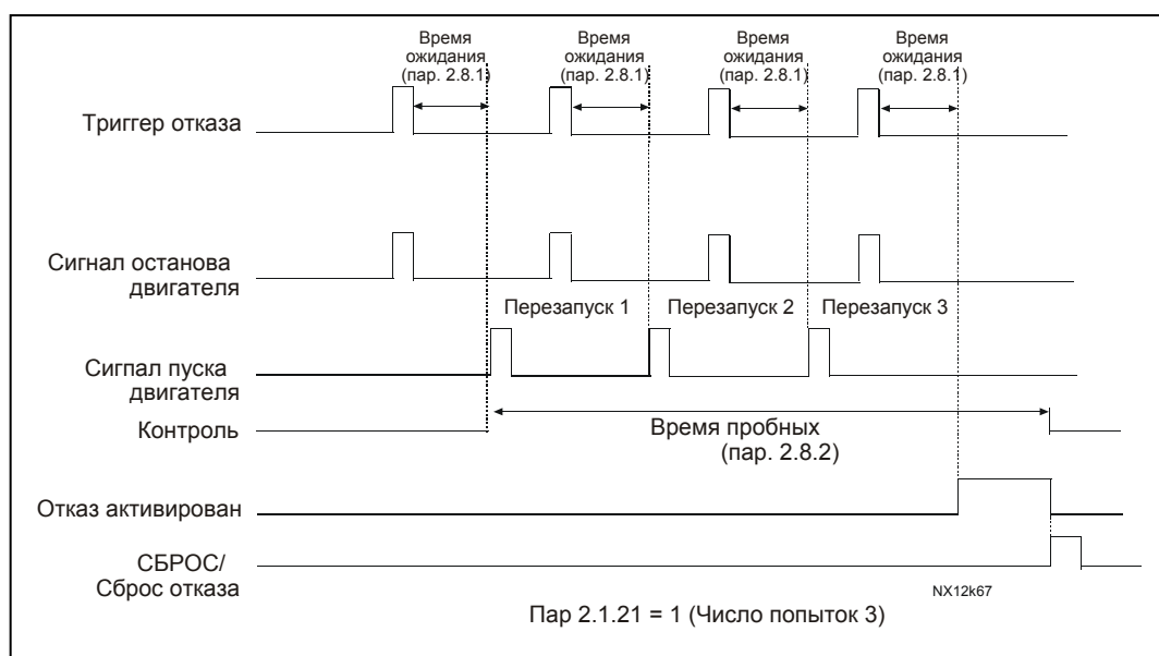
Рис. 1-24. Автоматический перезапуск
