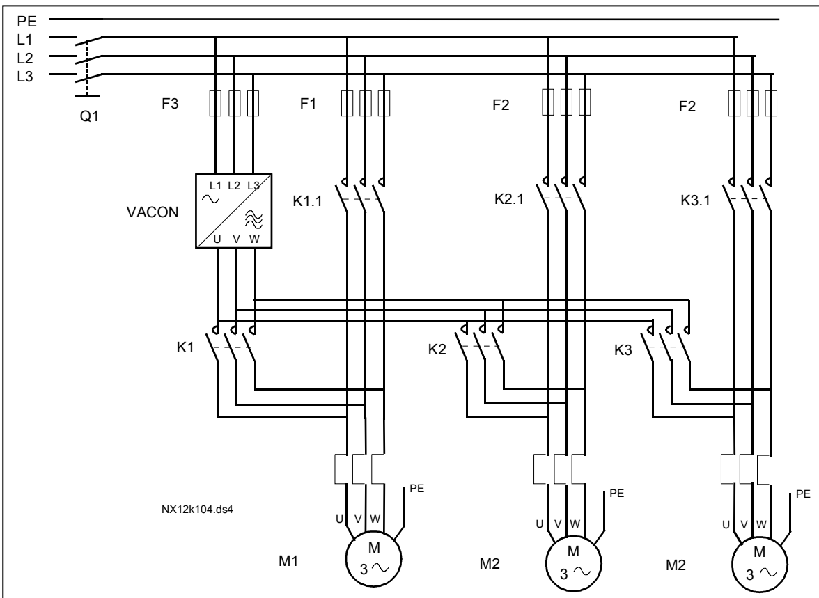
Рис. 1-32. Пример автозамены среди 3 насосов, силовая схема
