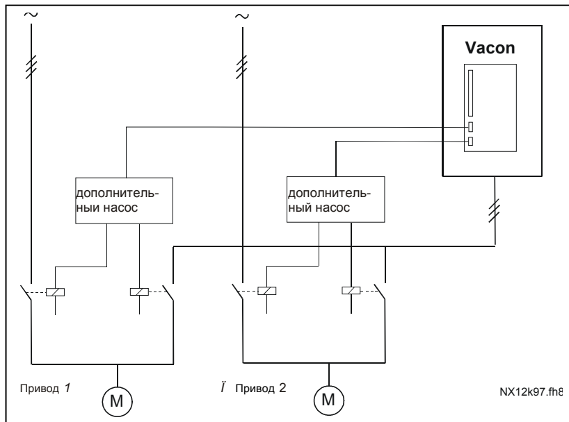
Рис. 1-36. Автозамена всех приводов
