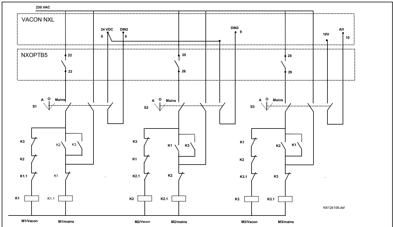
Рис. 1-31. Система из 3 насосов с автозаменой, принципиальная схема управления
