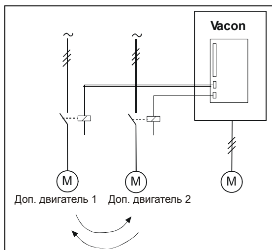
Рис. 1-35. Автозамена относится только к дополнительным приводам.
