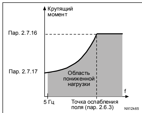
Рис. 1-22. Настройка минимальной нагрузки
