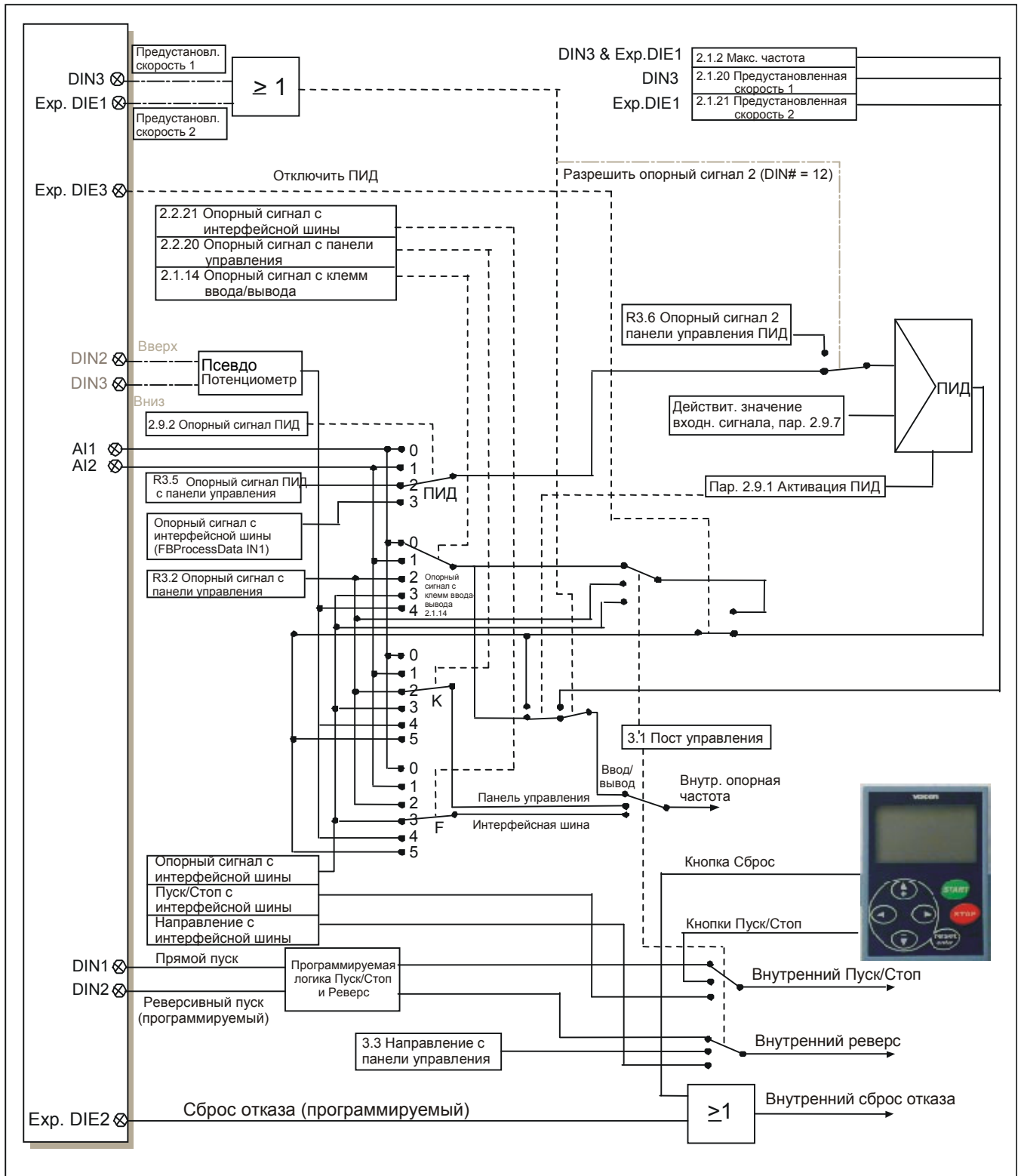
Рис. 1-38. Логика управляющих сигналов программы управления
