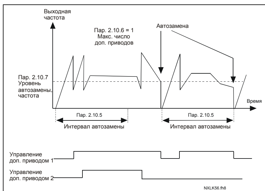
Рис. 1-37. Интервалы и пределы автозамены
