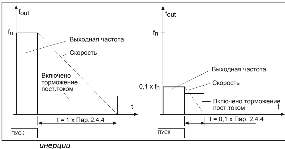
Рис. 1-11. Время торможения постоянным током в режиме останова = по инерции
