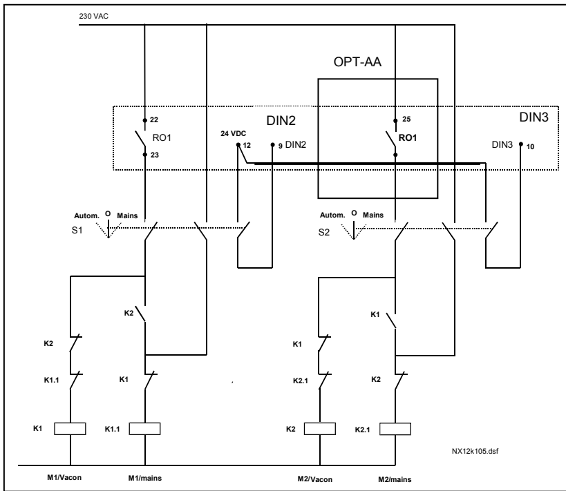
Рис. 1-33. Система из 2 насосов с автозаменой, принципиальная диаграмма управления
