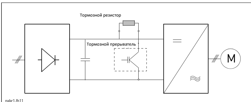
Рис. 1. Компоненты тормозов и стандартная схема подключения
