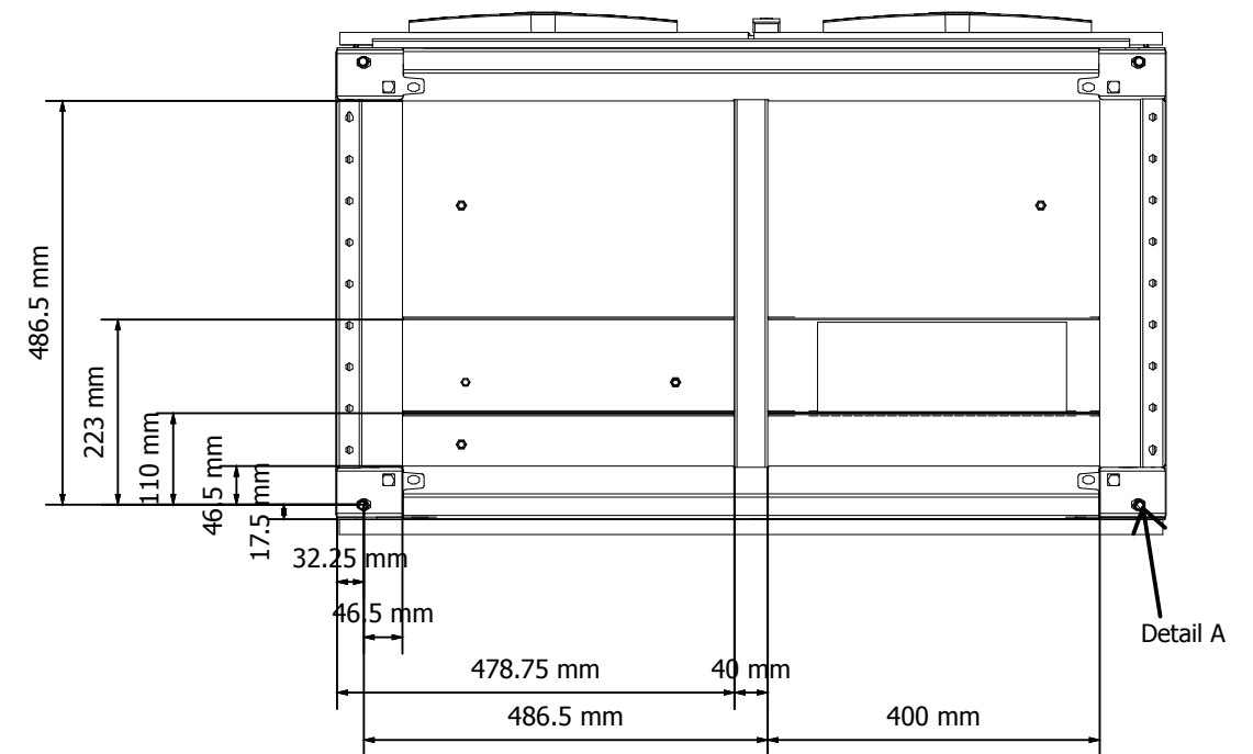
Bottom view Ansicht von unten
