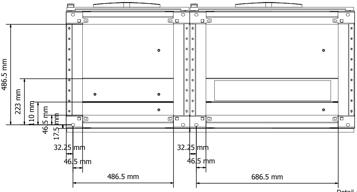
Bottom view Ansicht von unten
