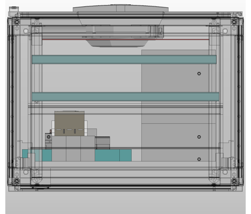
Bottom view Ansicht von unten
