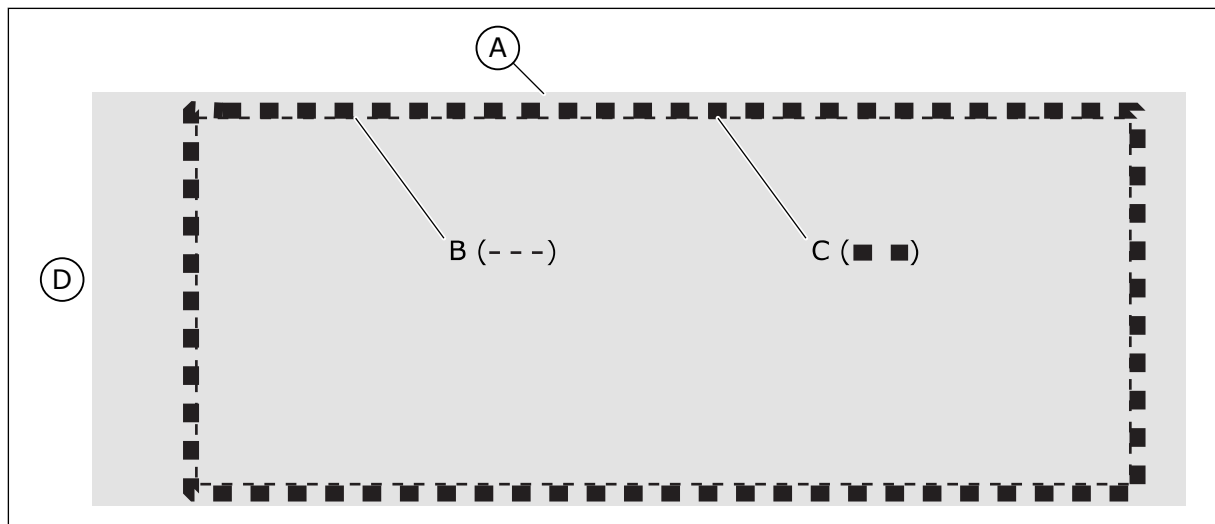
Abb. 20: Dichtung für die Öffnung für MR8, MR9 und MR10
