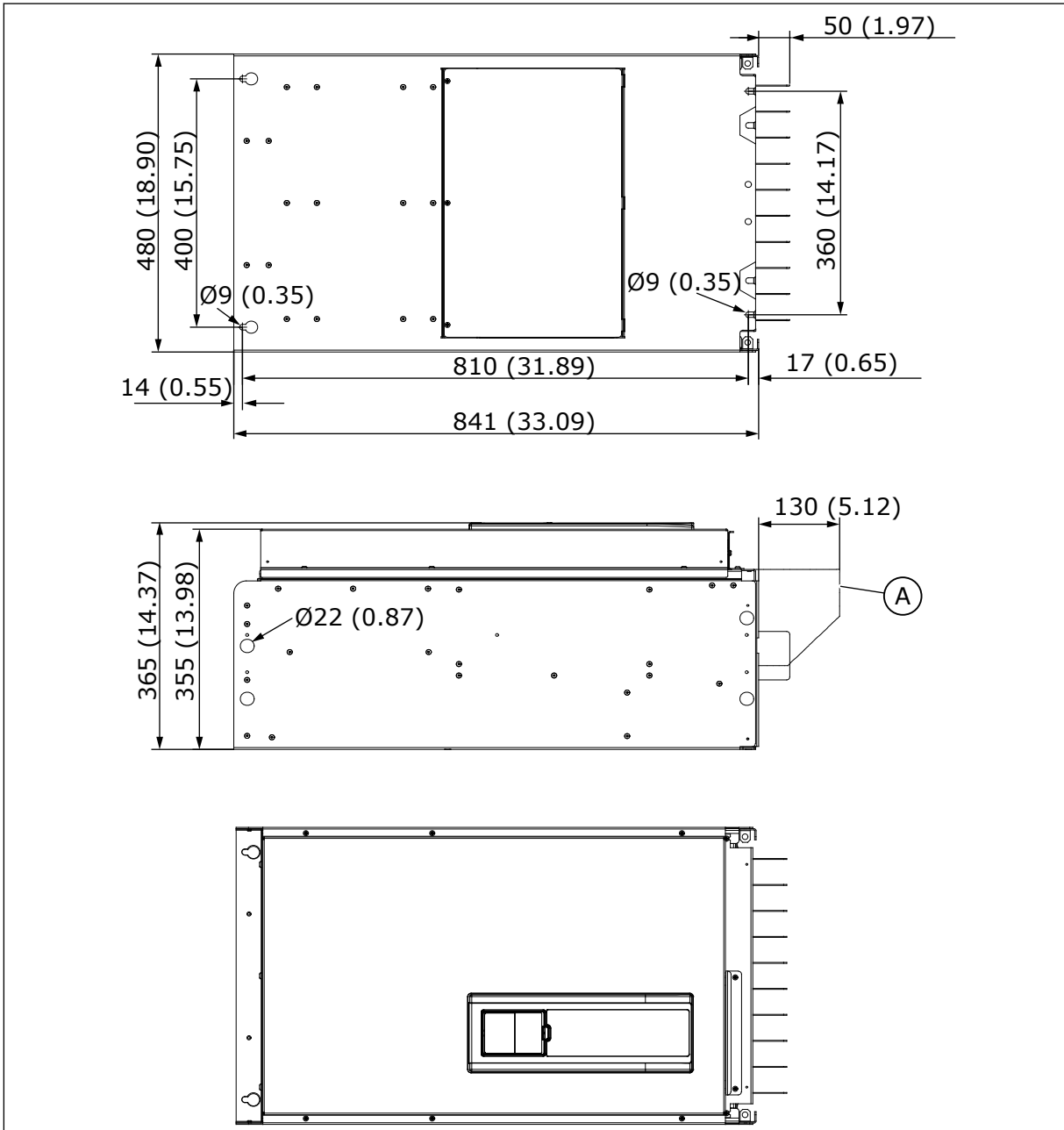
Abb. 4: Abmessungen des Frequenzumrichters MR9 [mm (in)]
