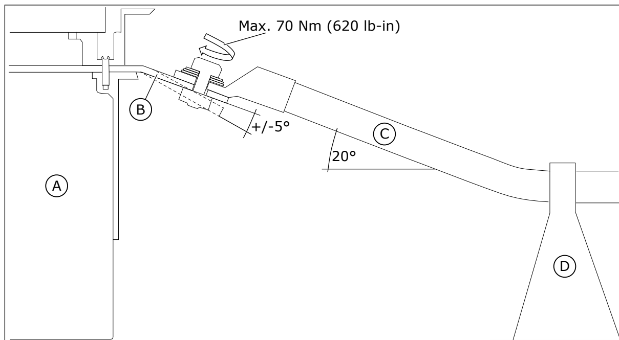
Abb. 24: Mechanische Stütze für die Kabel, wenn der Umrichter kein Optionsmodul aufweist
