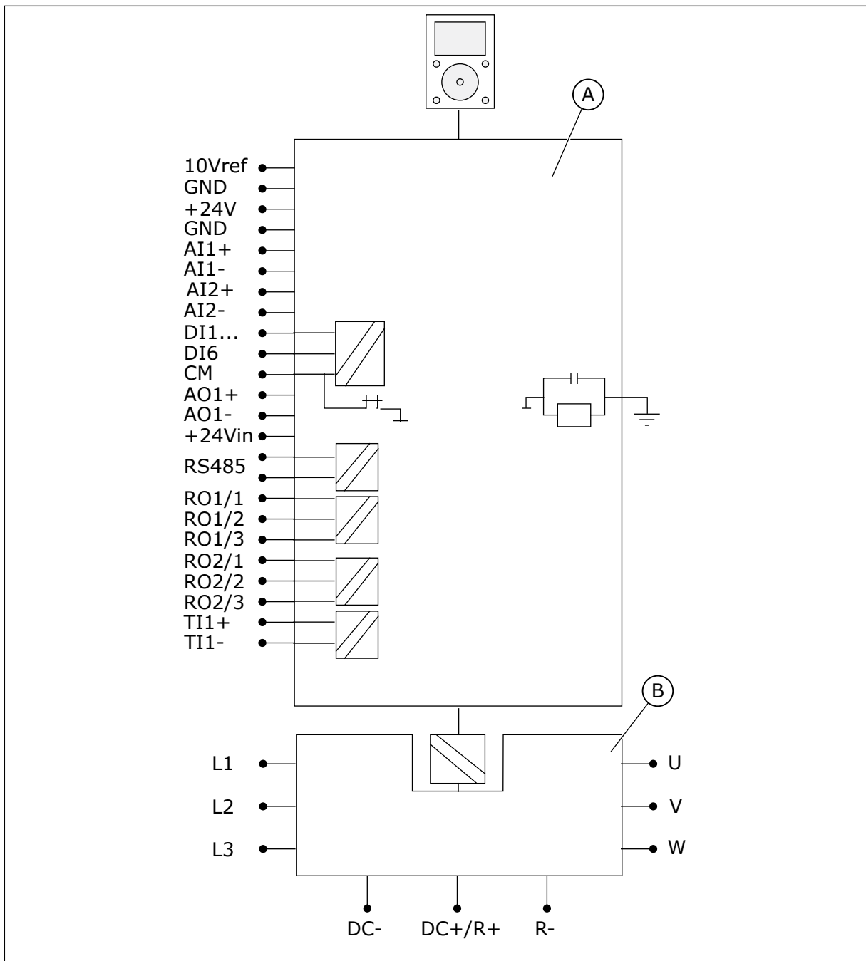
Abb. 32: Galvanische Trennung
