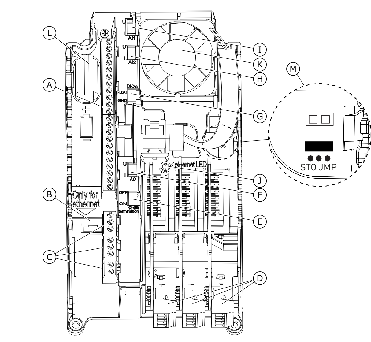
Abb. 25: Komponenten der Steuereinheit
