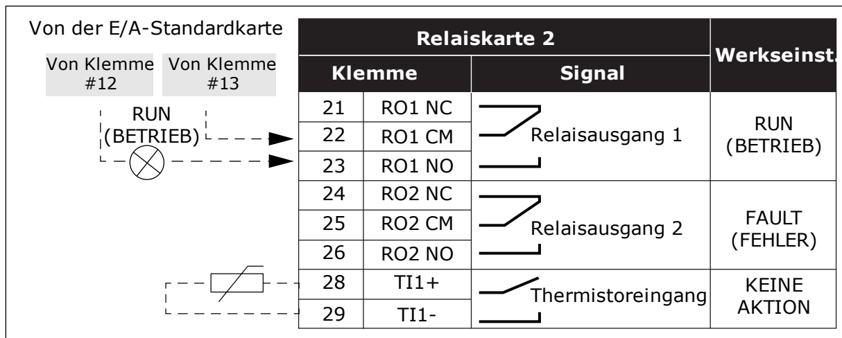
Abb. 28: Optionale Relaiskarte (+SBF4)
