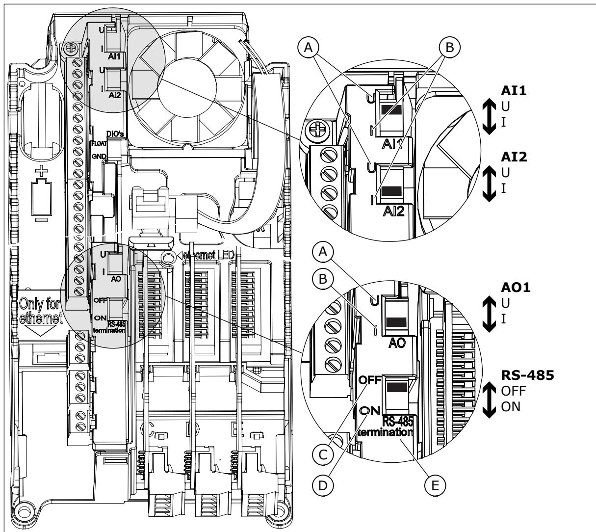
Abb. 29: Auswahlmöglichkeiten mit den DIP-Schaltern
