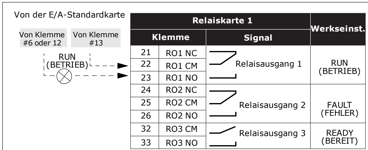
Abb. 27: Standardrelaiskarte (+SBF3)
