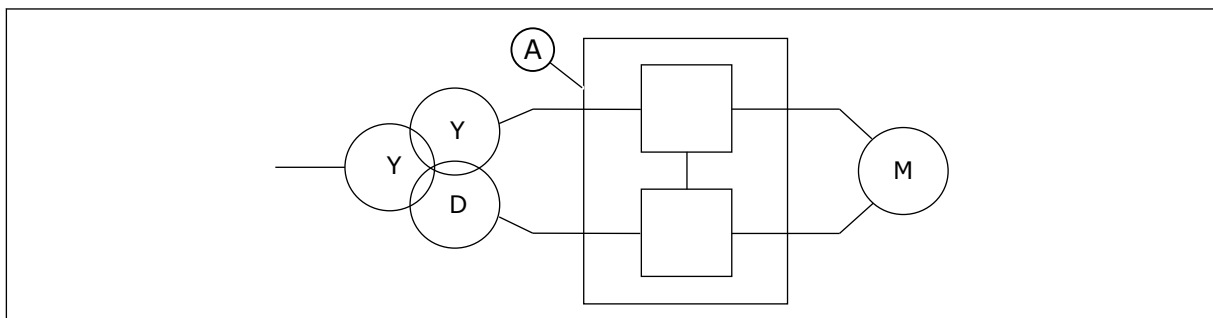
Abb. 17: Der 12-Puls-Betrieb des MR12
