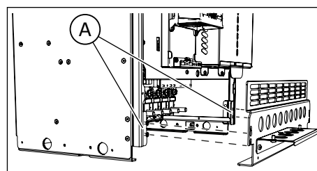
A. Die Schrauben
