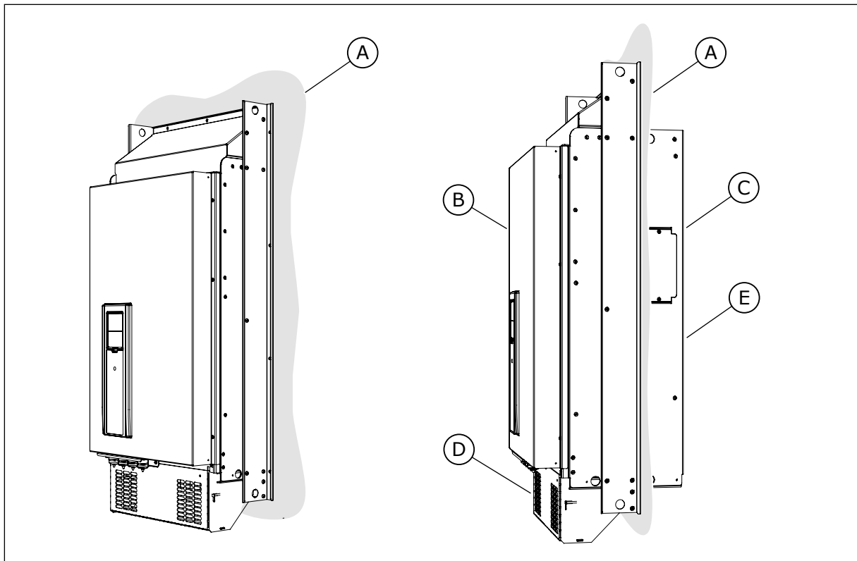
Abb. 18: Beispiel für eine Flanschbefestigung (Gehäusegröße MR9)
