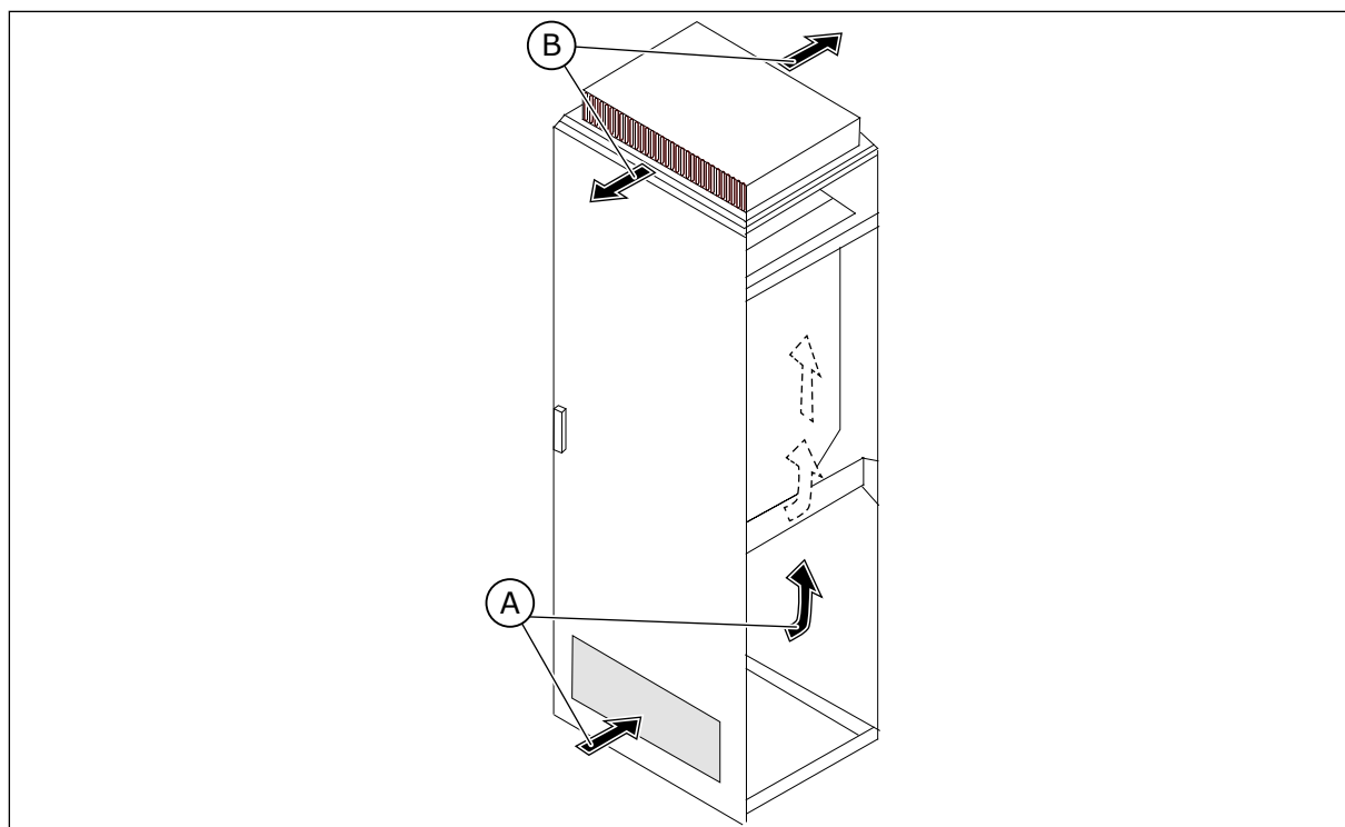
Abb. 22: Die Kühlluft muss sich im Schaltschrank frei bewegen
