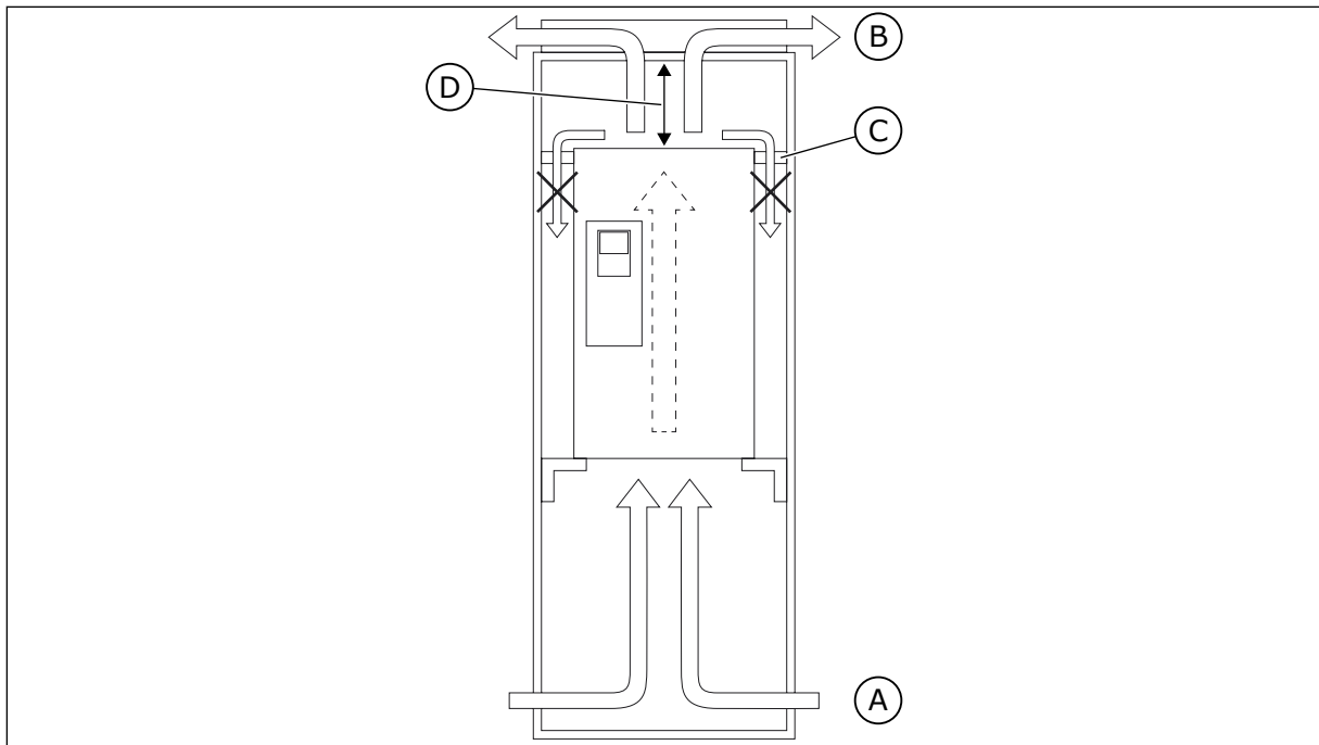
Abb. 21: Ordnungsgemäße Zirkulation der Kühlluft im Schaltschrank
