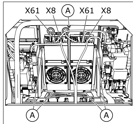
A. Die 5 Schrauben
