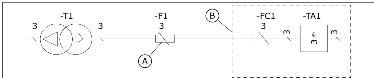
Abb. 23: Die Position der Sicherungen
