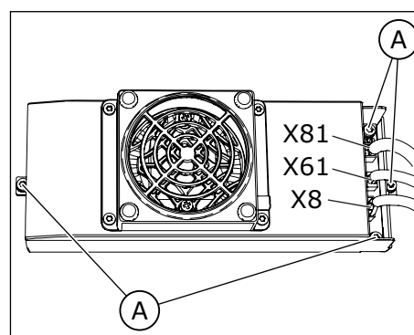
A. Die 4 Schrauben
