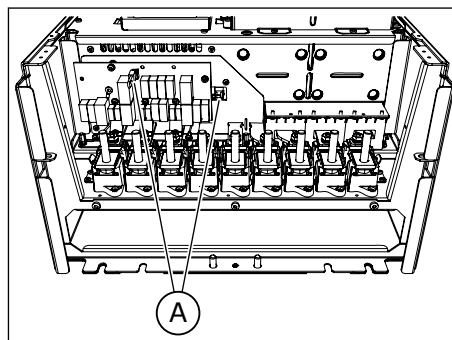
A. Die EMV-Steckbrücken
