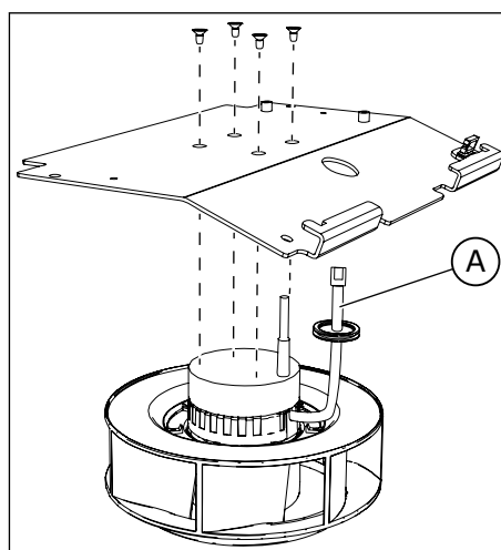
A. Das Lüfterkabel
