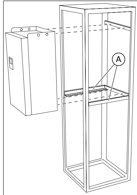
A. Die Schienen im Schaltschrank
