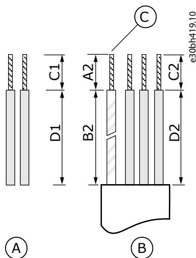
Ilustración 44: Pelado de los cables de suministro de CC y del motor
