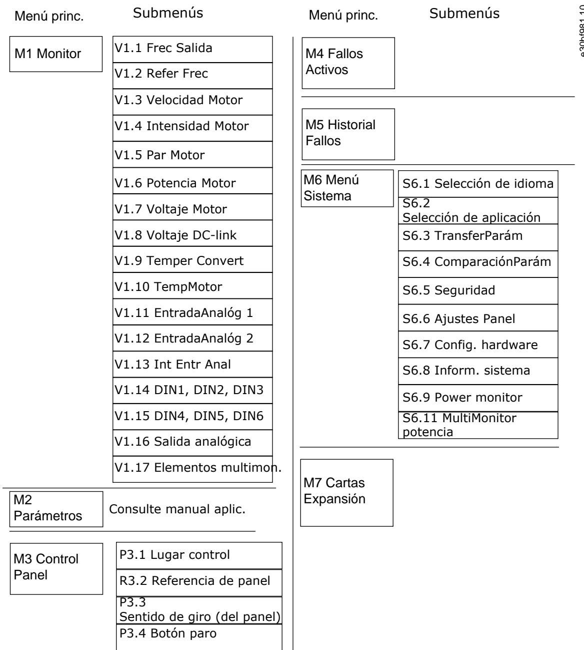
Ilustración 5: Estructura básica de menús del convertidor de frecuencia
