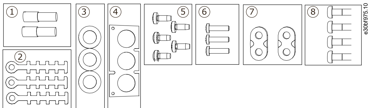
Ilustración 6: Contenido de la bolsa de accesorios para los modelos FR4-FR6/FI4-FI6
