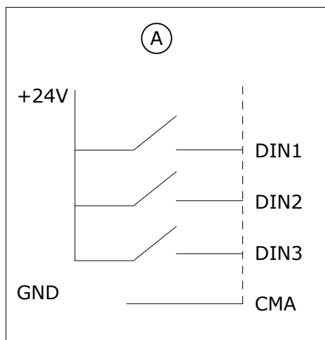
Ilustración 27: Lógica positiva o negativa
