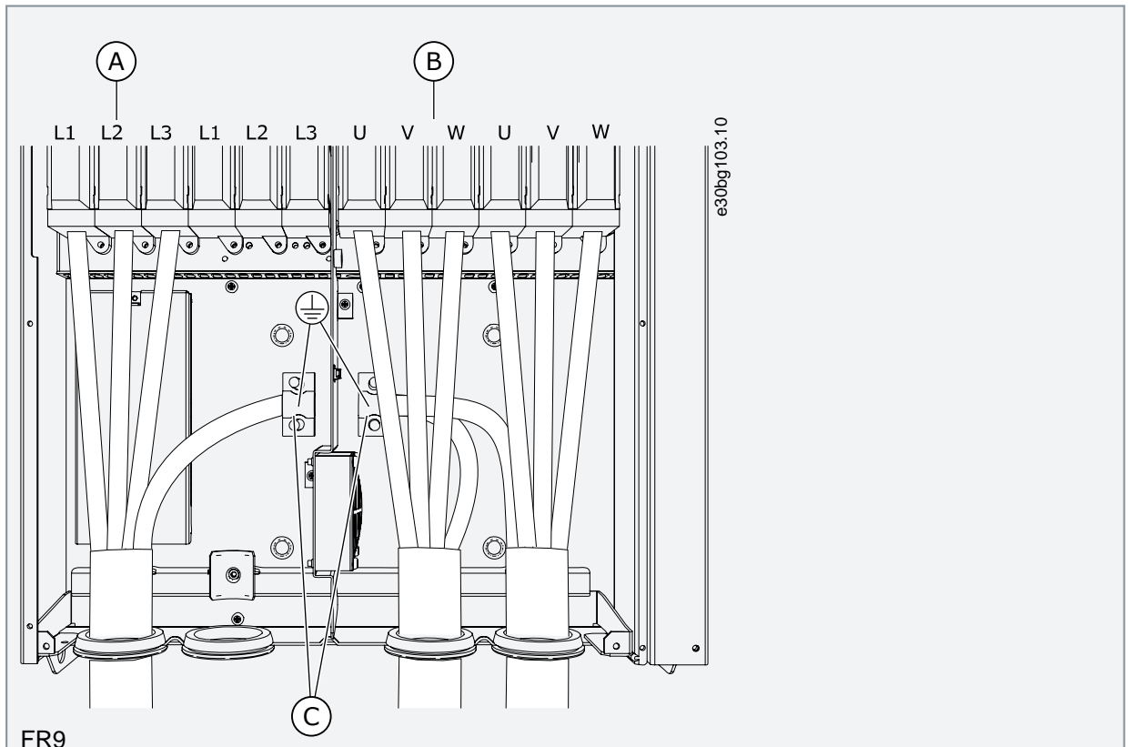
Afbeelding 21: FR9-klemmen
