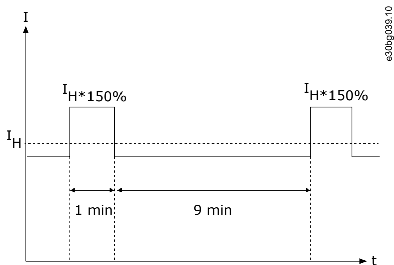
Afbeelding 75: Hoge overbelasting
