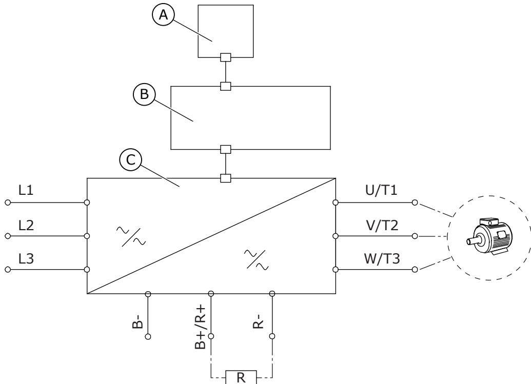
Afbeelding 13: Principeschema aansluitingen
