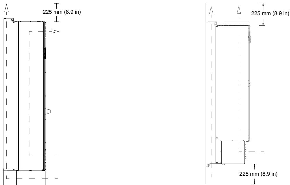
Illustrazione 69: Flusso d'aria per E1h/E2h (sinistra) ed E3h/E4h (destra)
