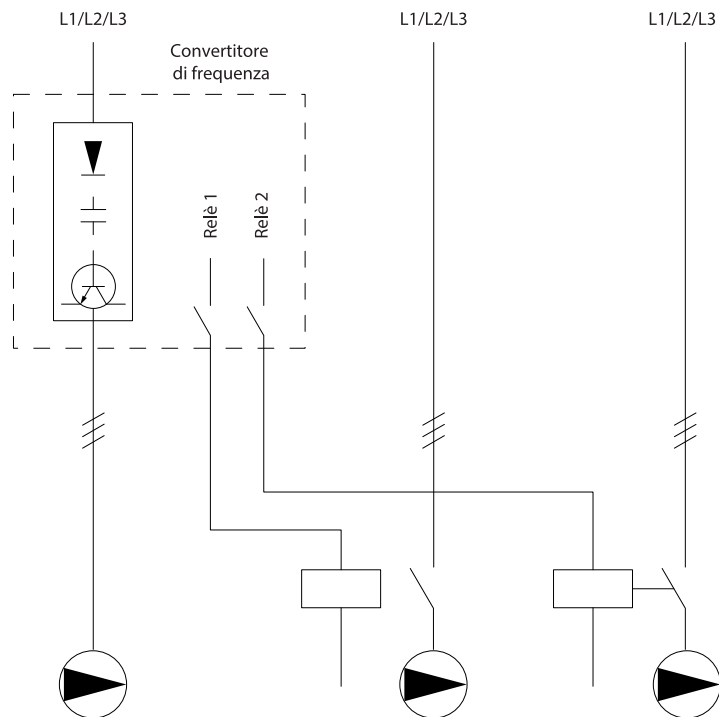
Illustrazione 46: Schema di cablaggio pompa a velocità variabile fissa
