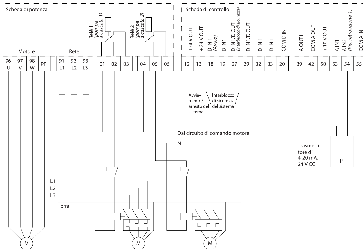
Illustrazione 45: Schema di cablaggio del Controllore in cascata
