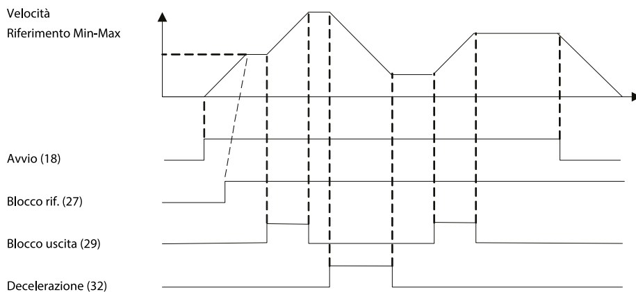
Illustrazione 40: Accelerazione/decelerazione
