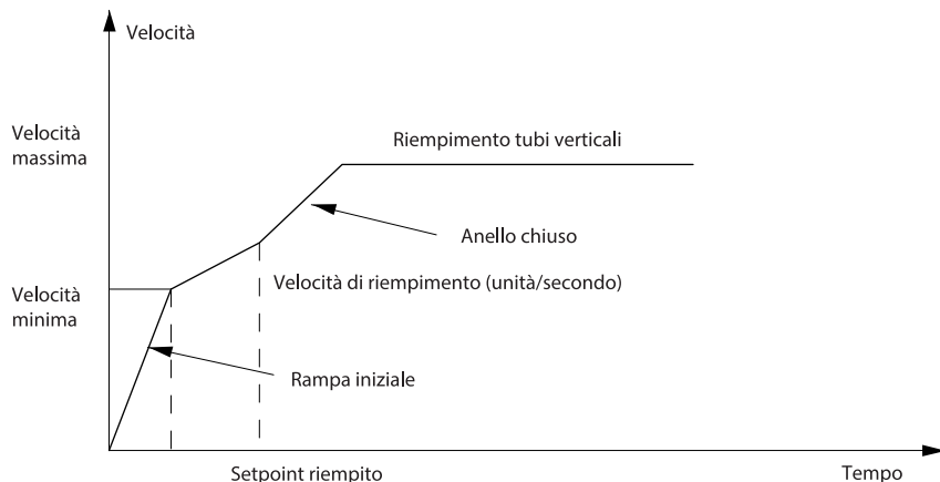
Illustrazione 44: Curva di prestazione per modo riempimento condutture
