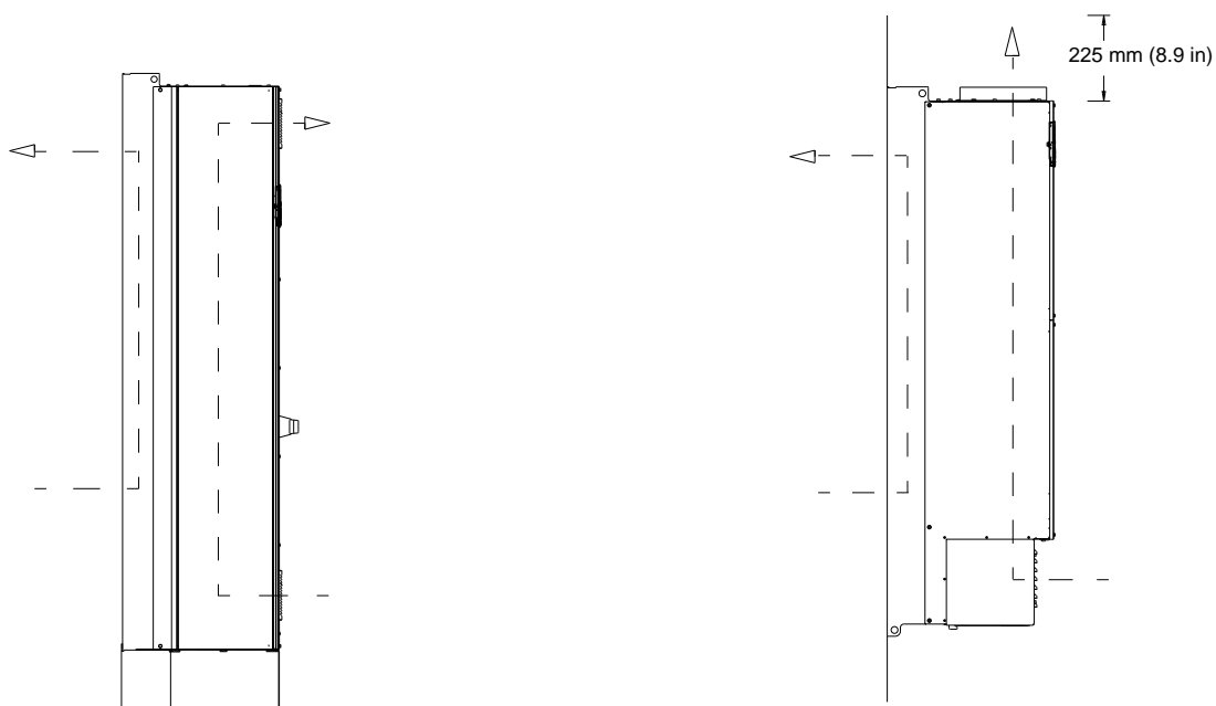
Illustrazione 70: Flusso d'aria con kit di raffreddamento della parete posteriore su E1h/E2h (sinistra) ed E3h/E4h (destra)
