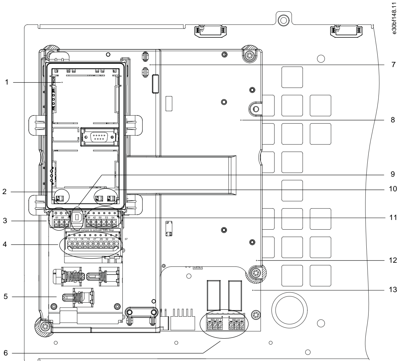
Illustrazione 4: Vista del rack di controllo
