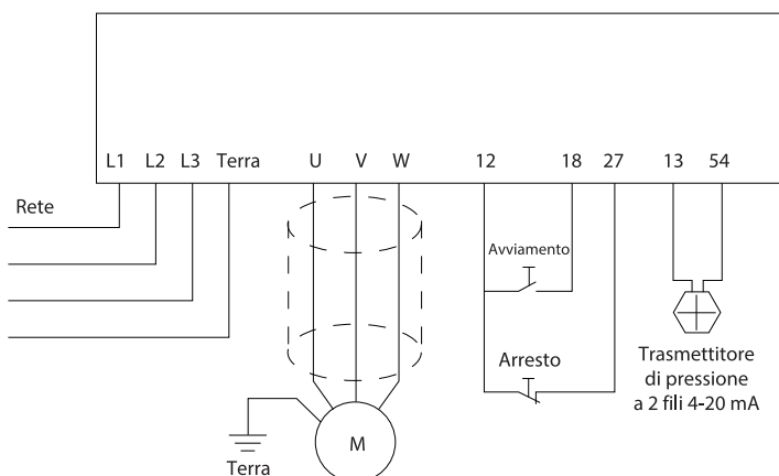
Illustrazione 43: Cablaggio per applicazione pompa sommersa
