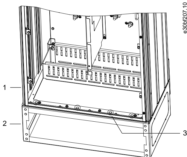
Illustrazione 12: Punti di montaggio tra piedistallo e contenitore
