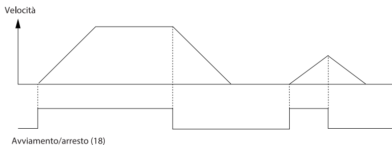
Illustrazione 41: Comando di avviamento/arresto con Safe Torque Off
