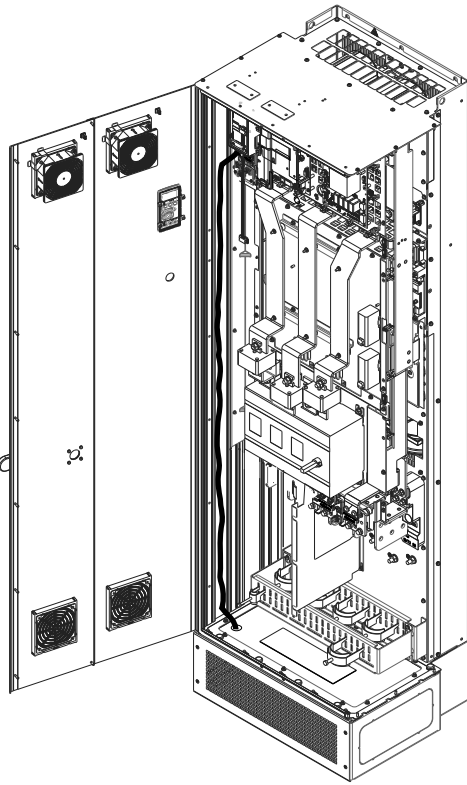
Illustrazione 32: Intradamento del cavo della scheda di controllo
