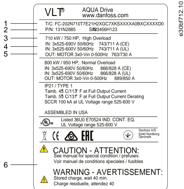
Illustrazione 8: Targa del prodotto per il contenitore E2h (esempio)
