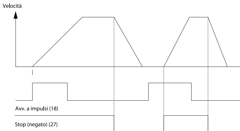
Illustrazione 42: Avviamento su impulso/arresto negativo
