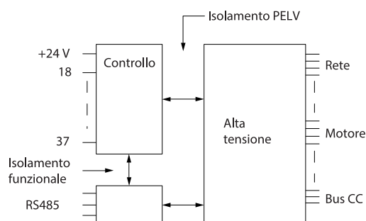
Illustrazione 52: Isolamento PELV
