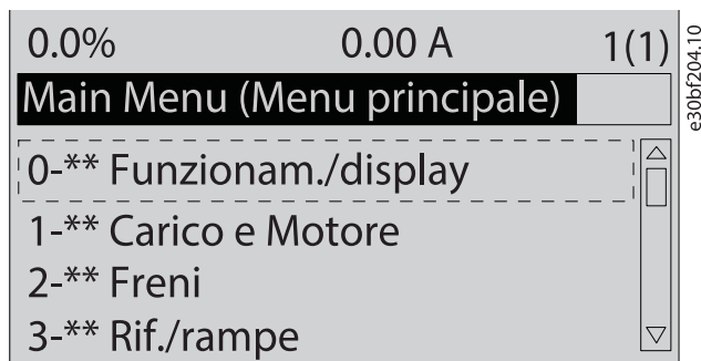
Illustrazione 7: Vista del menu principale
