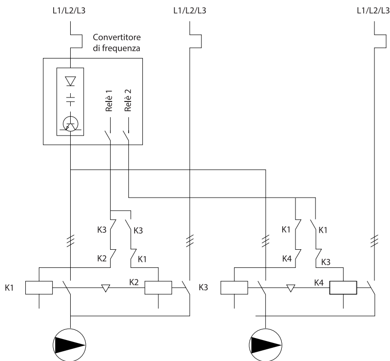
Illustrazione 47: Schema di cablaggio dell'alternanza della pompa primaria
