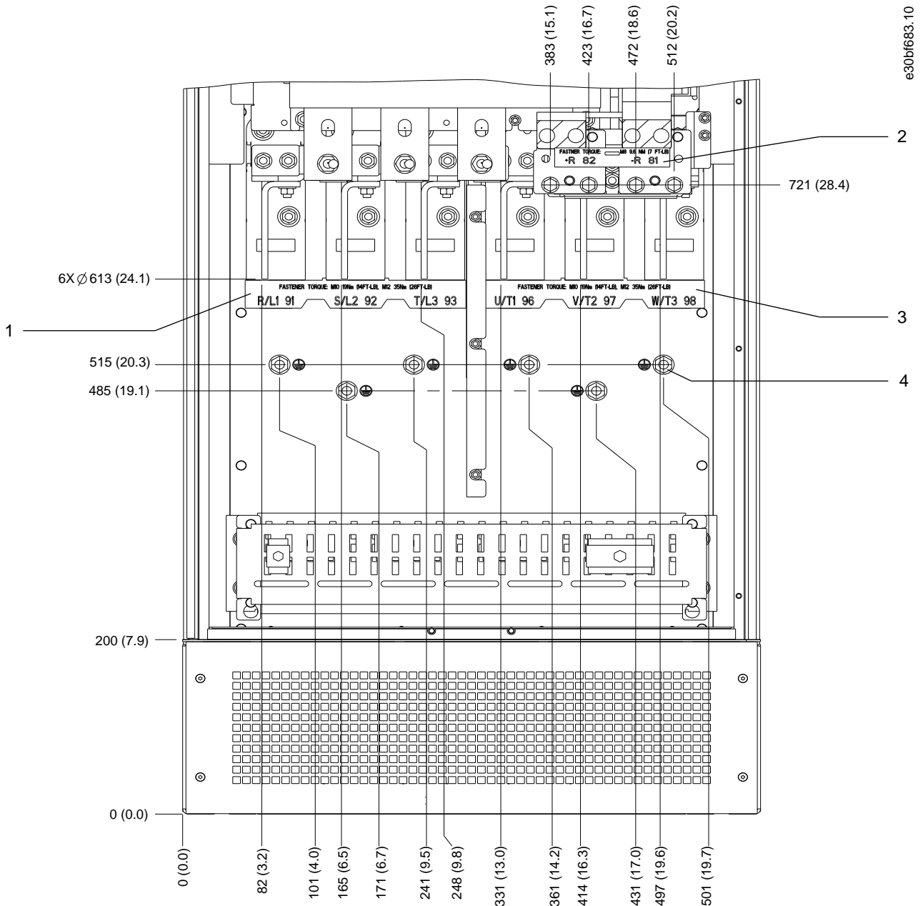
Ilustração 22: Dimensões dos terminais do E1h (vista frontal)
