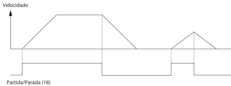
Ilustração 42: Comando de partida/parada com Safe Torque Off
