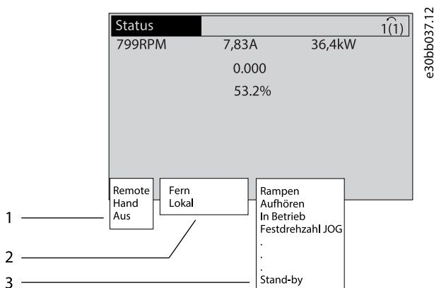
Abbildung 26: Statusanzeige
