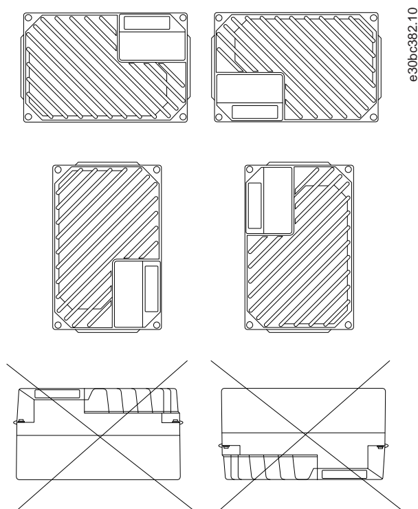
Abbildung 5: Zulässige Montagepositionen – Standardanwendungen
