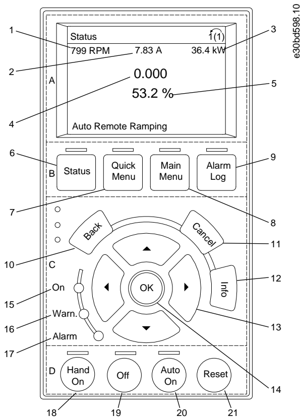
Abbildung 22: Bedieneinheit (LCP)
