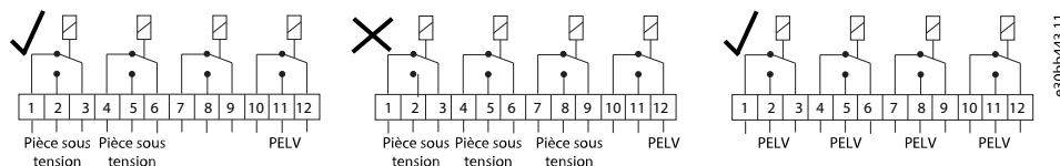
Illustration 3: Branchements valides pour isolation galvanique
