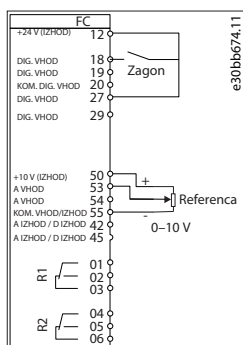
Ilustracija 27: Ožičenje frekvenčnega pretvornika
