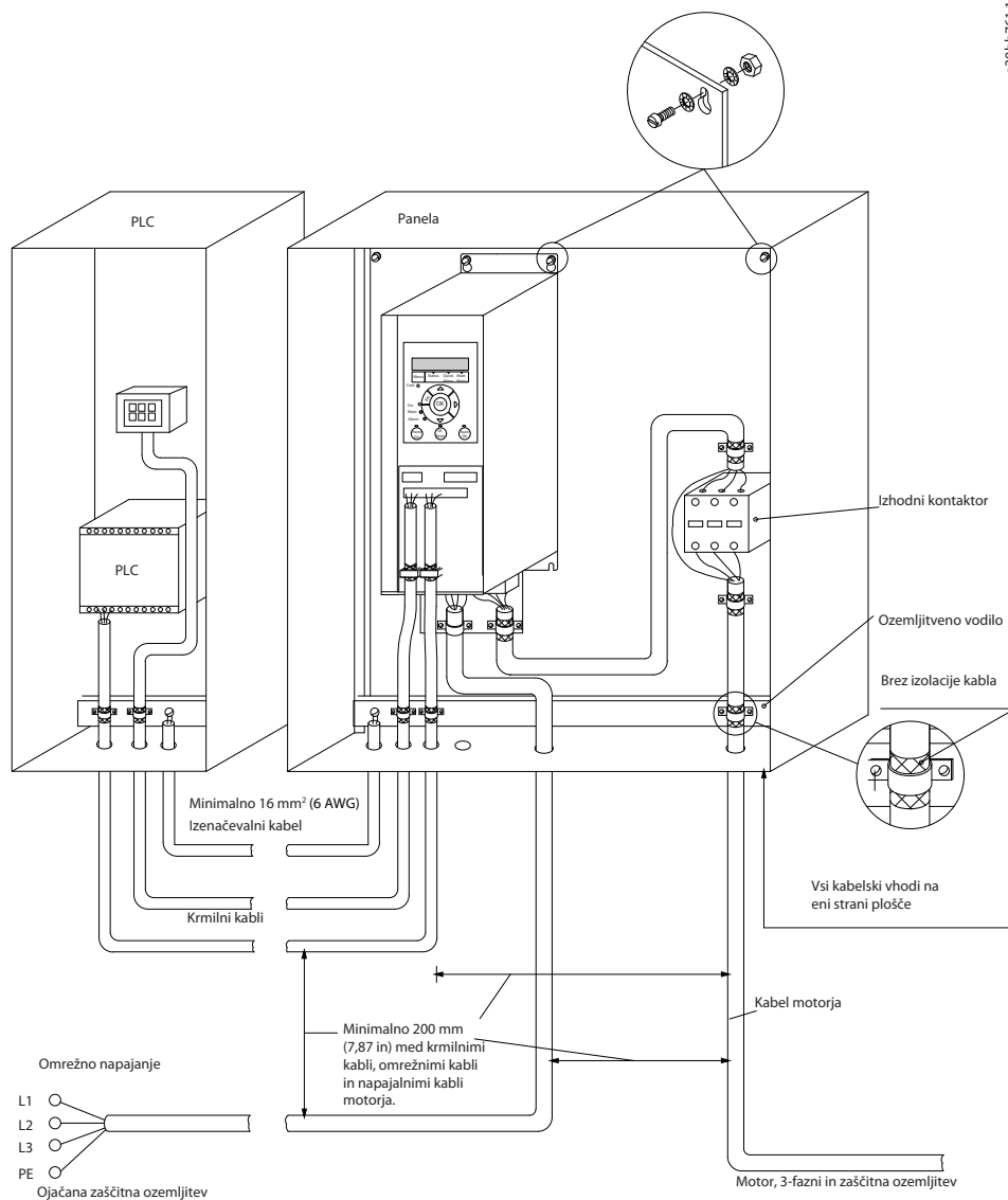
Ilustracija 22: EMC-ustrezne električne napeljave
