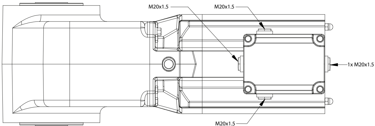
Afbeelding 8: Schroeven aansluitkast
