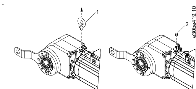
Afbeelding 6: De oogbout na installatie vervangen door de kunststof dop
