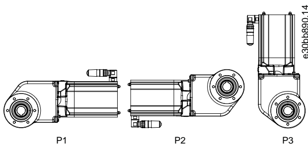
Afbeelding 12: Montageposities
