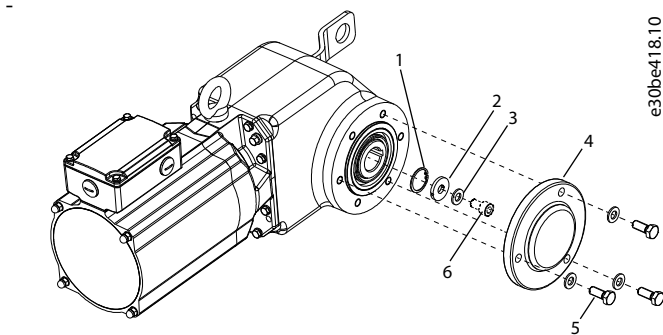
Afbeelding 5: De montage-inrichting en de afdekking van de holle as monteren
