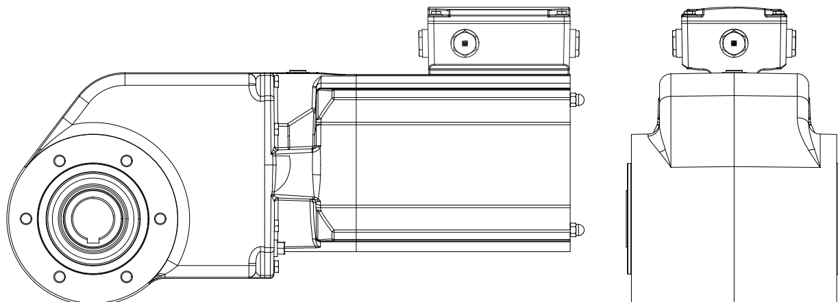
Ilustração 7: Caixa de terminais
