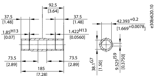
Ilustração 28: Eixo I1 de aço/aço inoxidável
