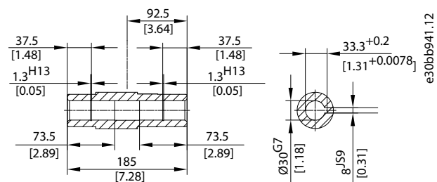
Ilustração 23: Eixo de 30 mm de aço/aço inoxidável
