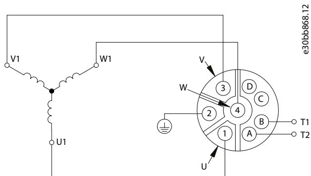
Ilustração 10: Diagrama da Conexão CleanConnect® OneGearDrive
