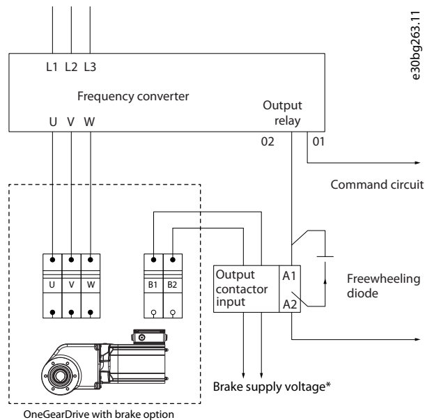
Ilustração 33: Exemplo de conexão do freio mecânico ao conversor
