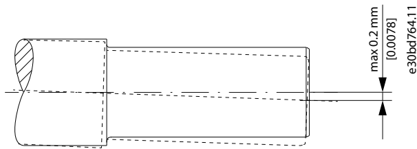
Ilustração 3: Excentricidade máxima do eixo do transportador
