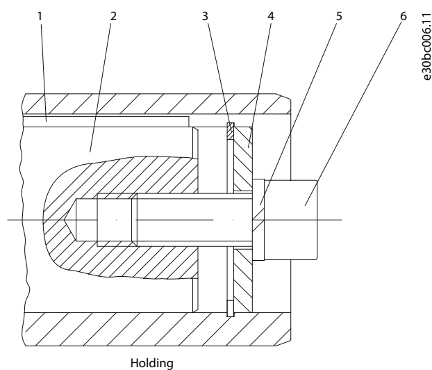
Ilustração 1: Kit de montagem
