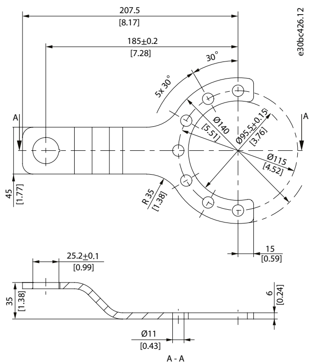
Ilustração 29: Braço de torque
