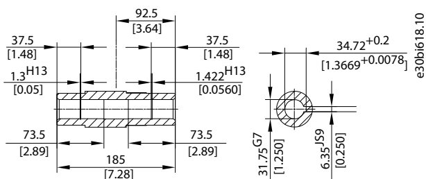
Ilustração 26: Eixo I1 de aço/aço inoxidável
