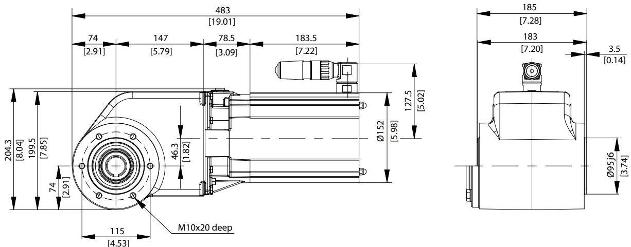
Ilustração 20: VLT® OneGearDrive® Hygienic
