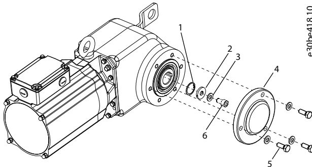
Ilustração 5: Montagem da disposição de montagem e da tampa do eixo oco
