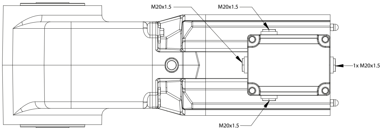
Ilustração 8: Parafusos da caixa de terminais
