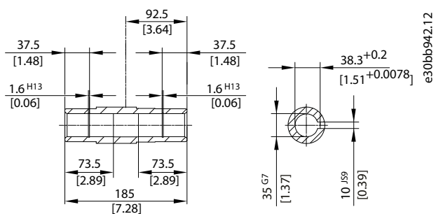
Ilustração 24: Eixo de 35 mm de aço/aço inoxidável
