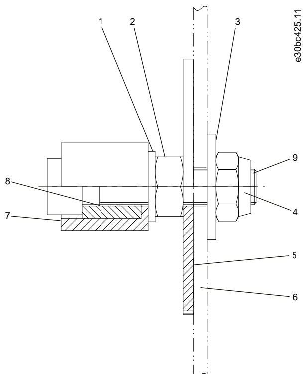
Ilustração 29: Braço de torque
