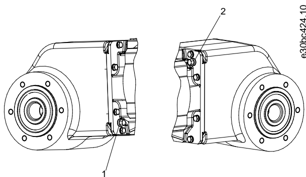
Ilustração 13: Parafusos de óleo do VLT® OneGearDrive® 1 e 2
