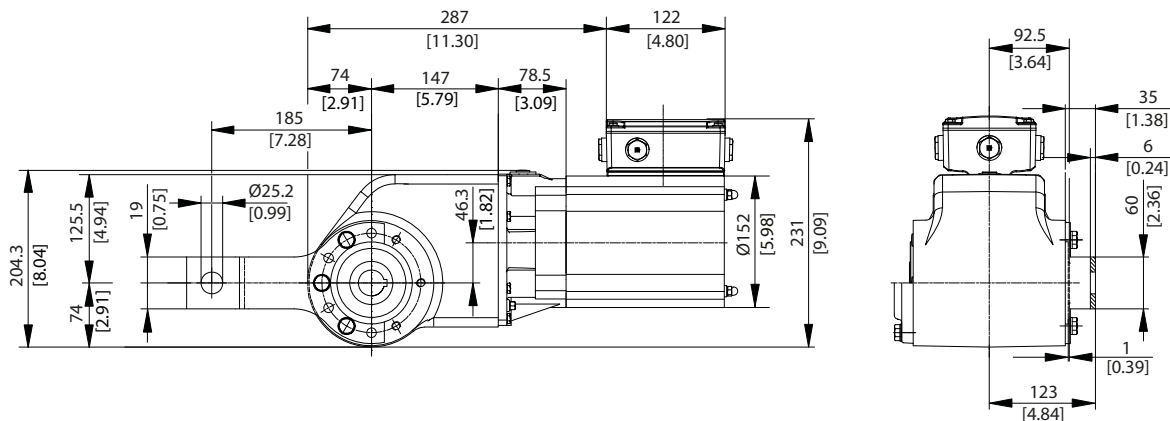
Ilustração 19: VLT® OneGearDrive® Standard com braço de torque na posição frontal (opcional)
