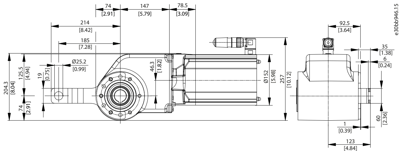
Ilustração 22: VLT® OneGearDrive® Hygienic com braço de torque na posição frontal (opcional)
