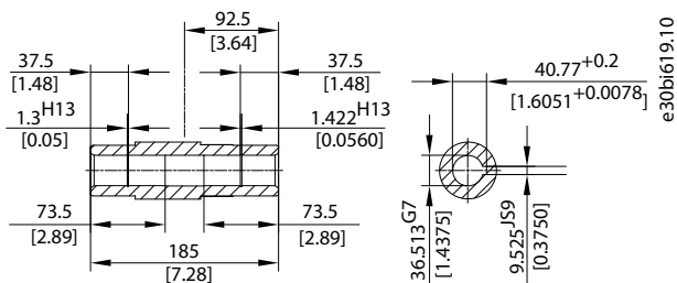
Ilustração 27: Eixo I2 de aço/aço inoxidável
