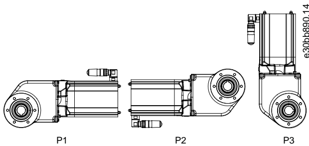
Ilustração 12: Posições de montagem
