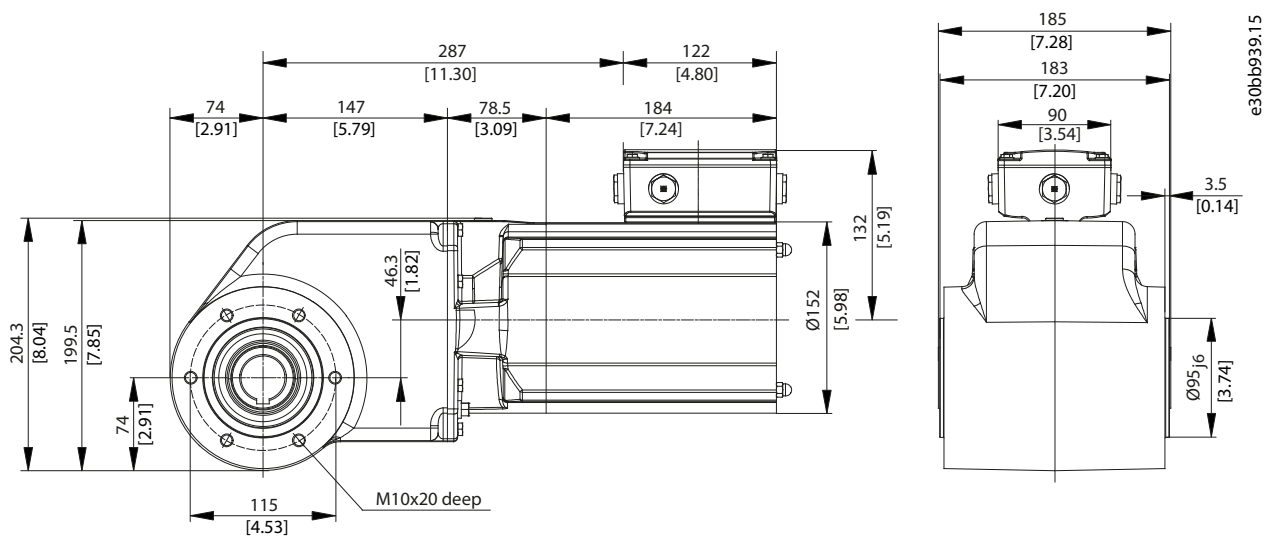
Ilustração 18: VLT® OneGearDrive® Standard
