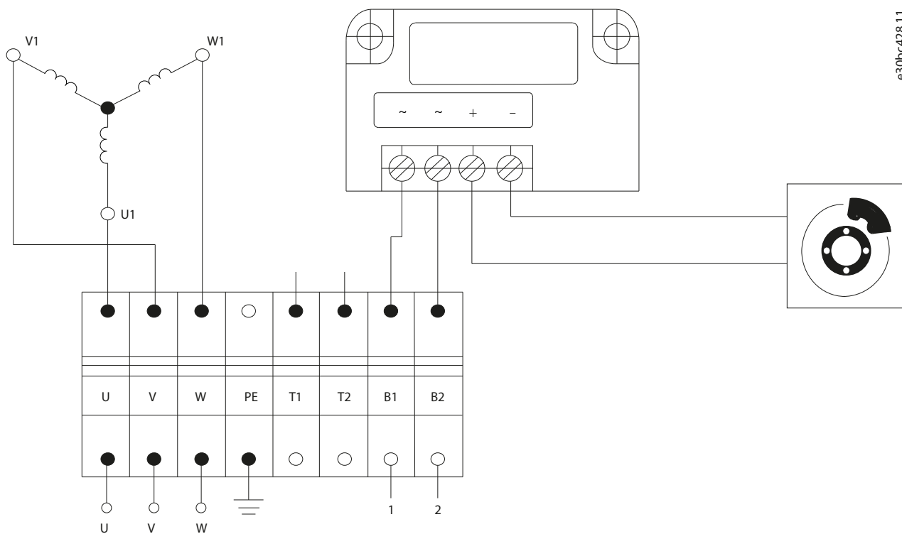
Ilustração 32: Braçadeira de fixação e conexão com o VLT® AutomationDrive FC 302
