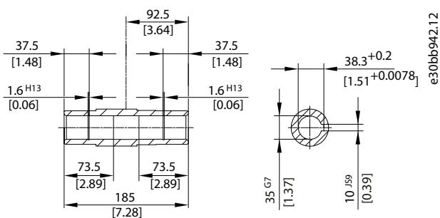
Illustration 24: Arbre en acier/acier inoxydable de 35 mm
