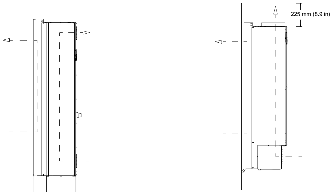
Abbildung 69: Luftzirkulation mit Einbausatz für Rückwand-Kühlung für E1h/E2h (links) und E3h/E4h (rechts)
