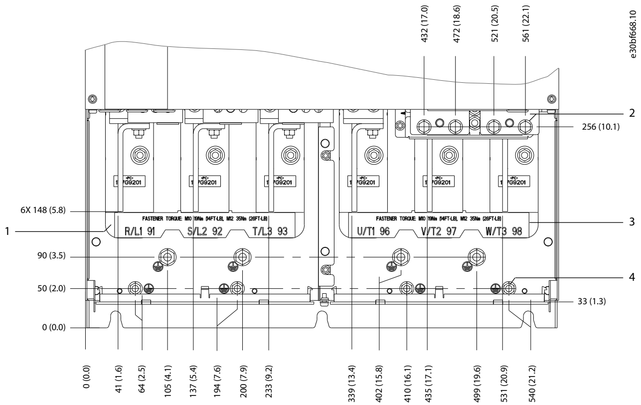
Abbildung 28: E4h-Klemmenabmessungen (Frontansicht)
