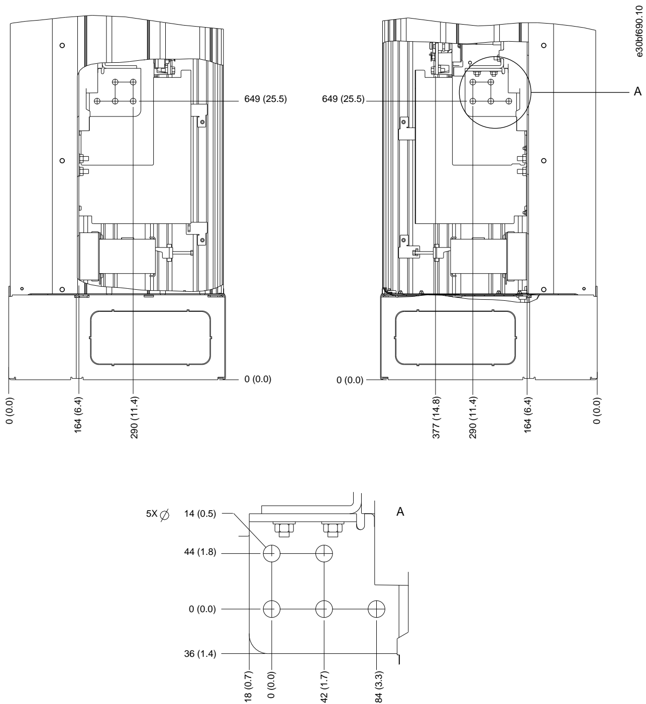
Abbildung 24: E2h-Klemmenabmessungen (Seitenansichten)
