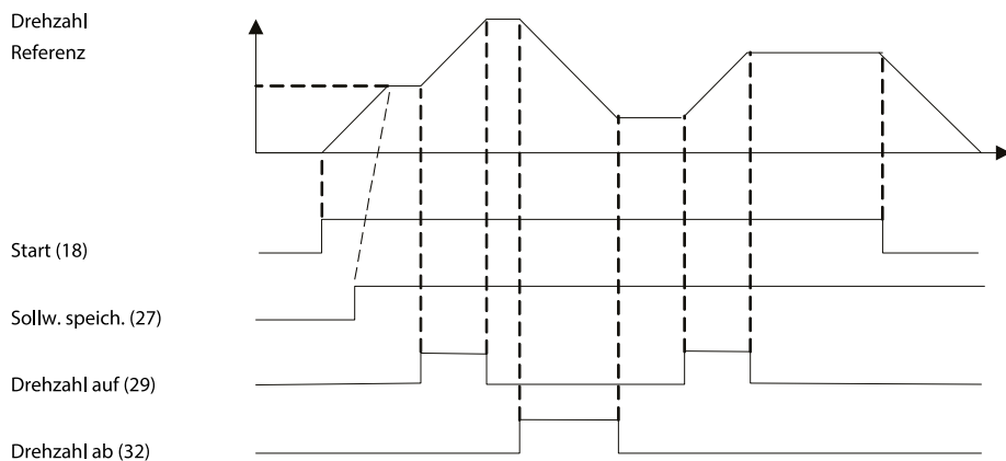
Abbildung 39: Drehzahlkorrektur auf/ab
