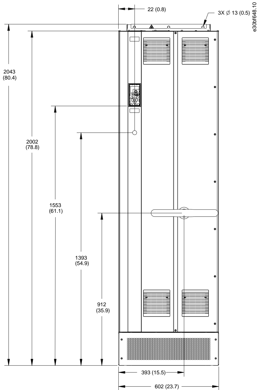
Abbildung 52: Frontansicht E1h
