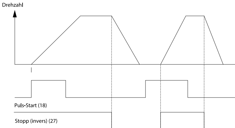
Abbildung 41: Puls-Start/Stop invers
