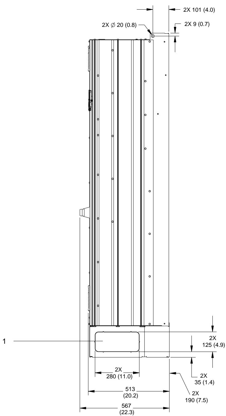
Abbildung 57: Seitenansicht E2h
