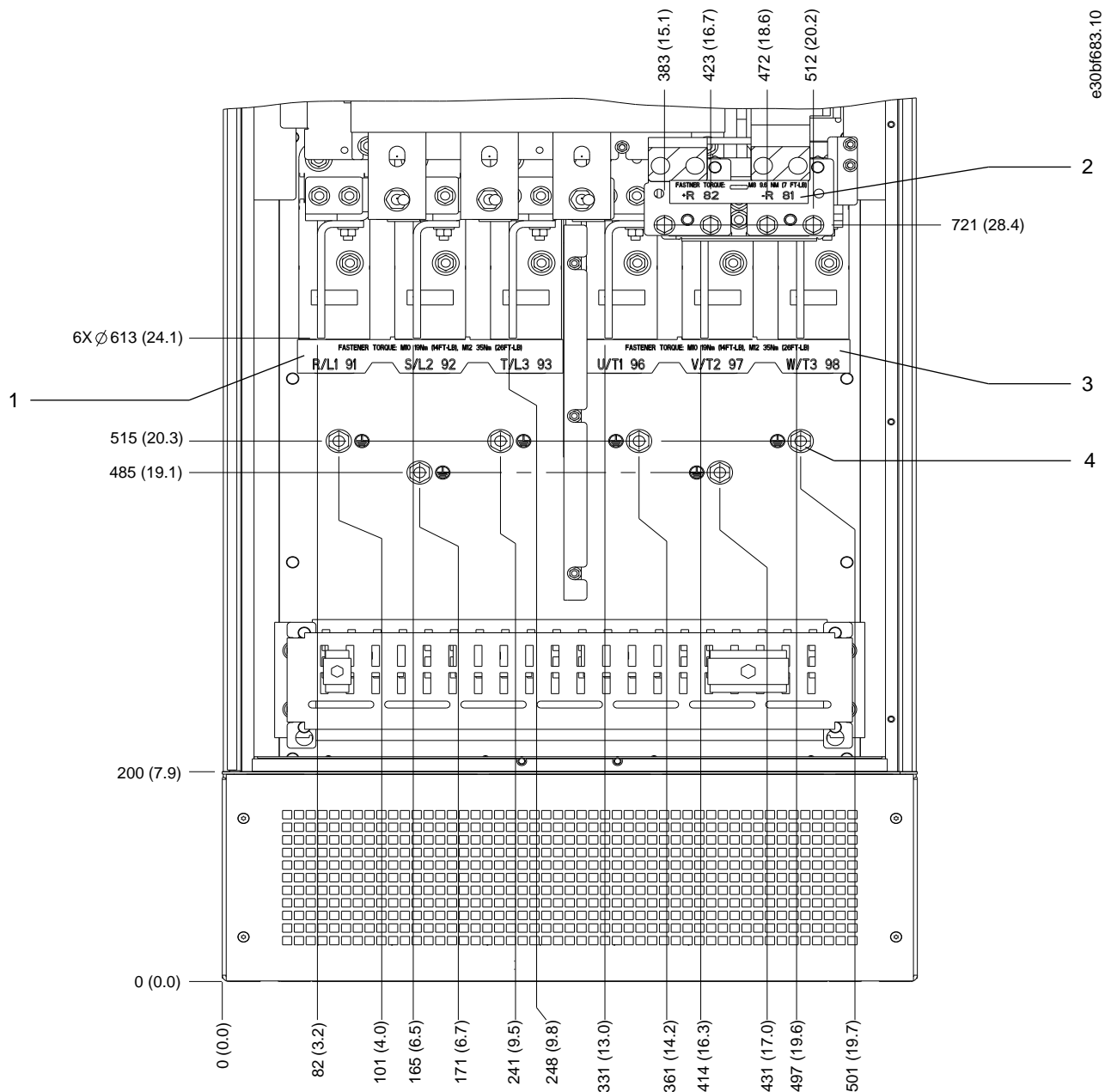
Abbildung 21: E1h-Klemmenabmessungen (Frontansicht)
