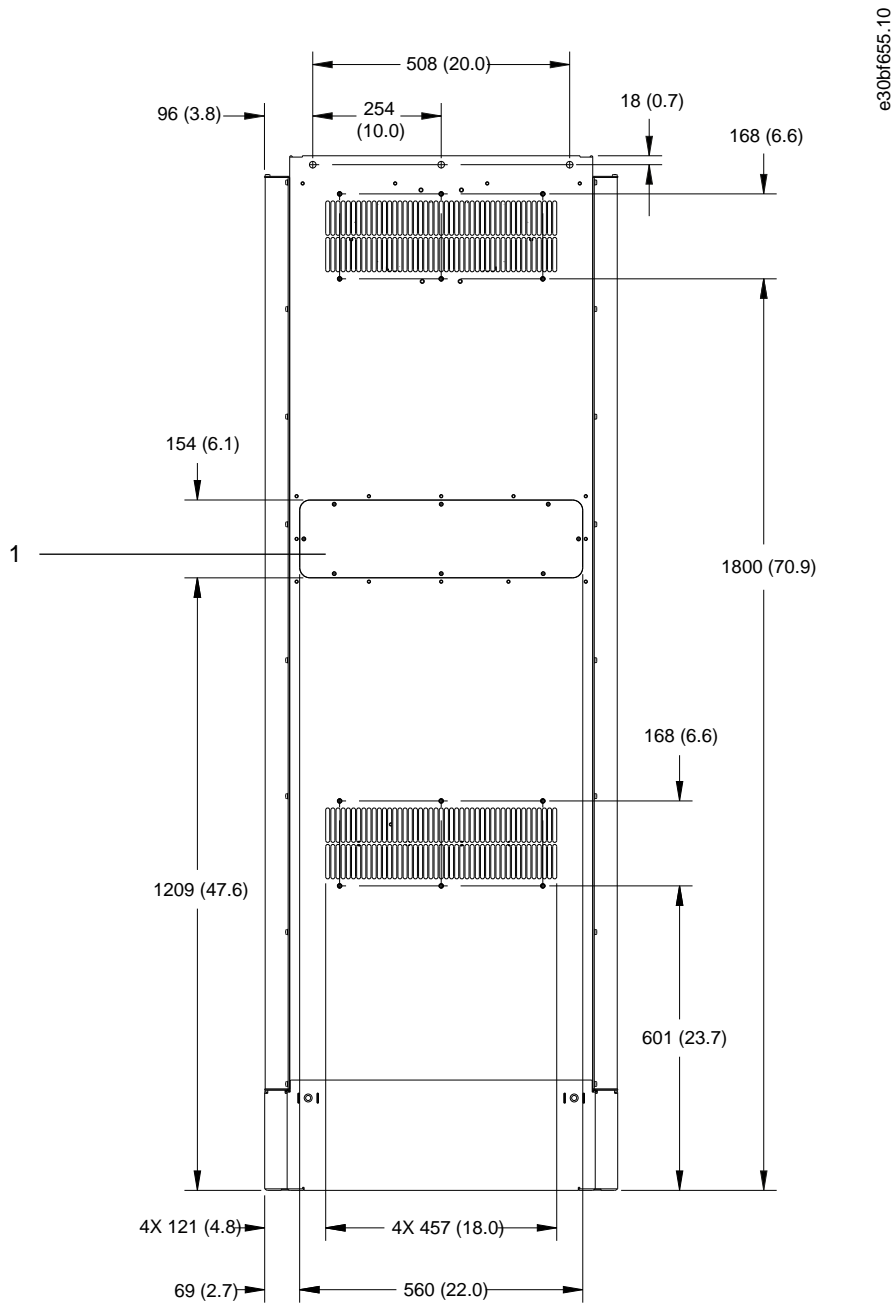
Illustration 58: Vue arrière du boîtier E2h
