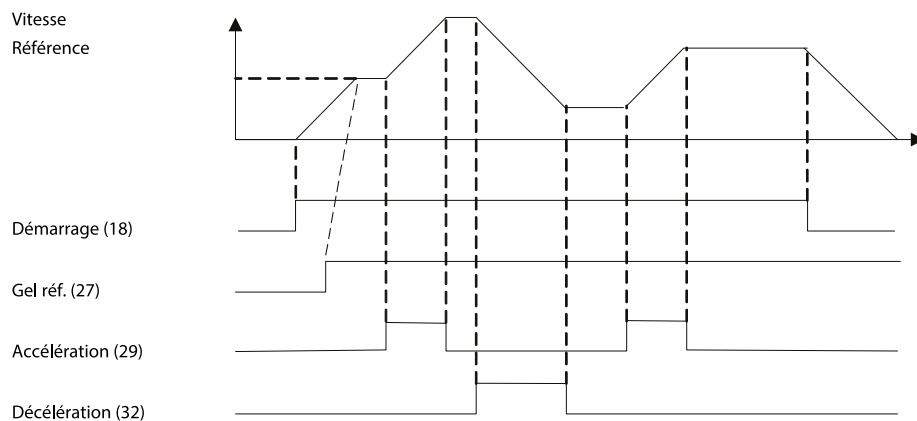
Illustration 39: Accélération/décélération
