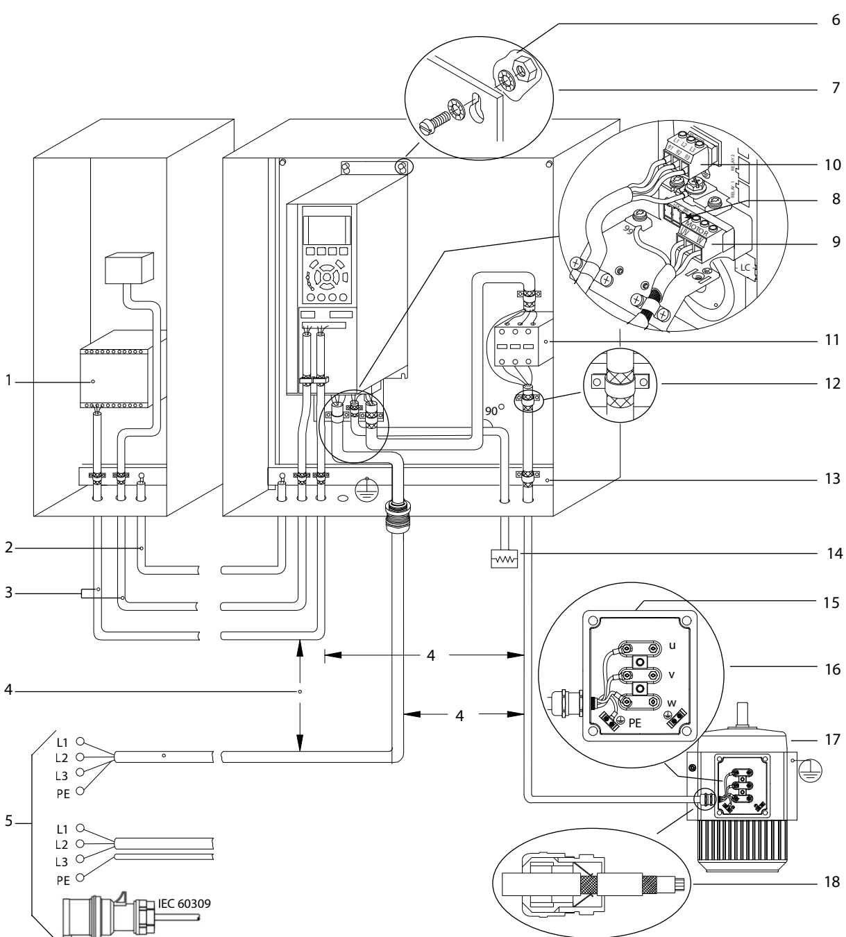
Illustration 16: Exemple d'installation conforme aux exigences CEM
