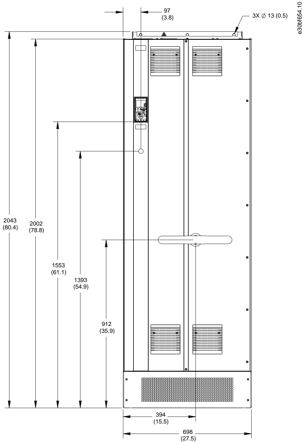
Illustration 56: Vue de face du boîtier E2h
