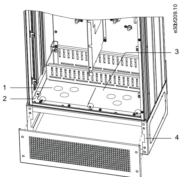
Illustration 12: Installation de la plaque d'entrée des câbles
