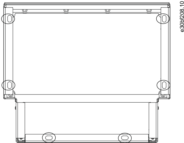
Illustration 9: Points de fixation du socle au sol (entourés)
