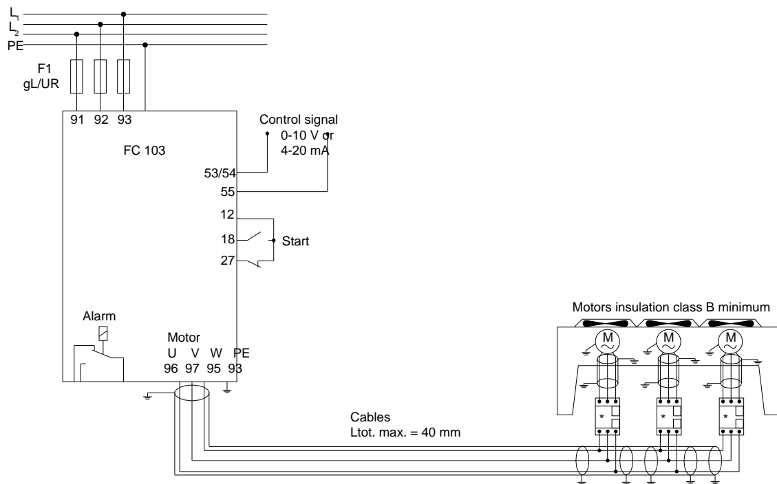
Illustration 43: Commande de vitesse utilisant la référence analogique (boucle ouverte) – Ventilateur ou pompe unique/ventilateurs ou pompes multiples en parallèle
