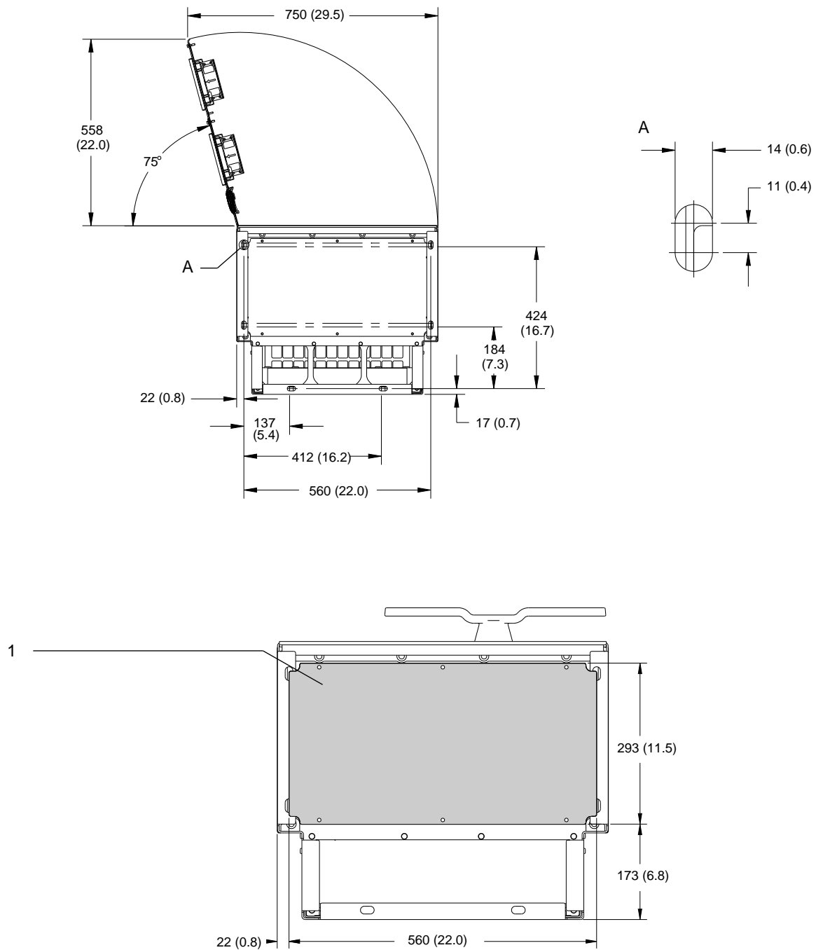
Illustration 55: Espace pour la porte et dimensions de la plaque d'entrée des câbles pour E1h
