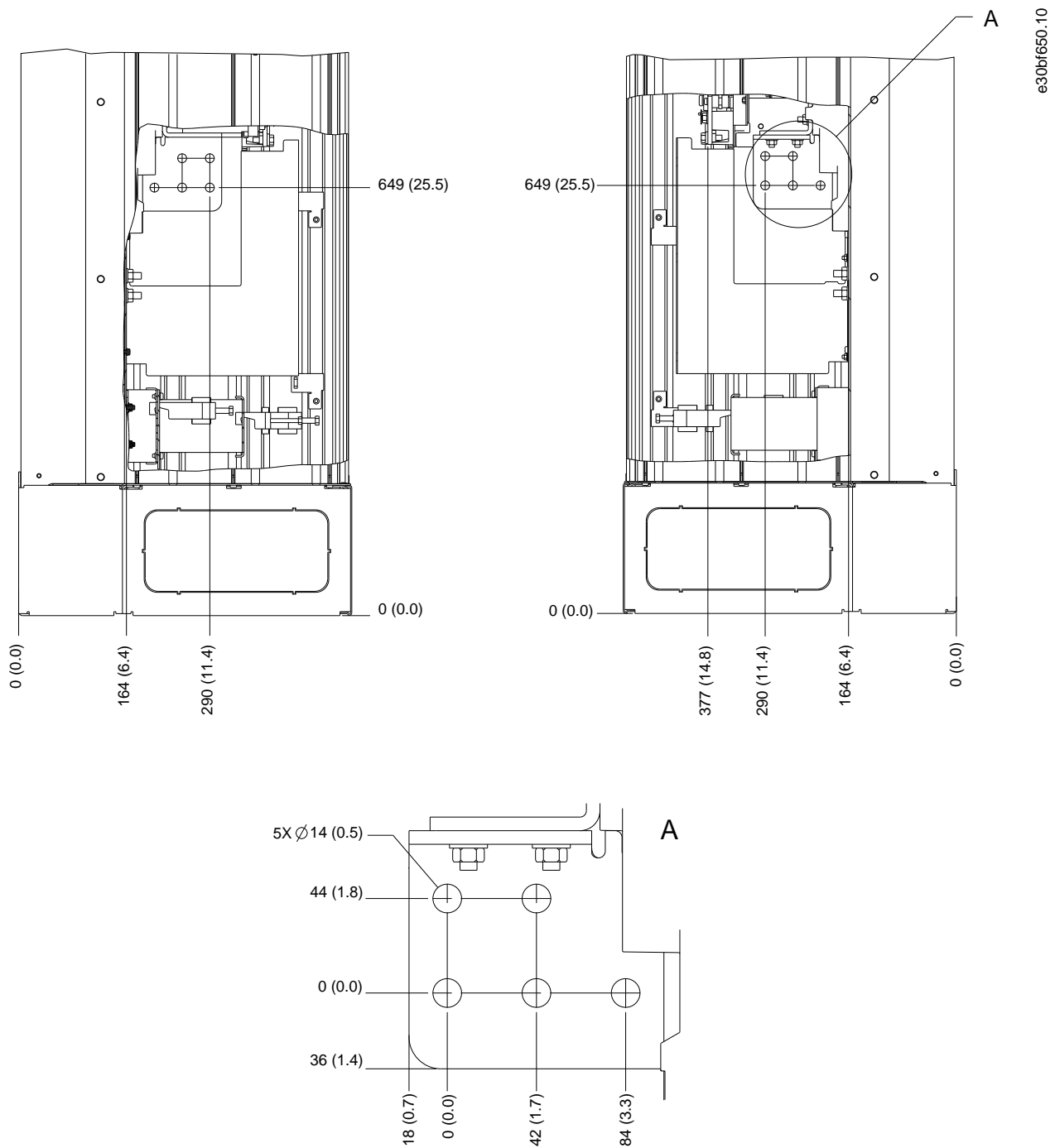
Illustration 22: Dimensions des bornes E1h (vues latérales)
