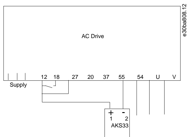
Illustration 46: Connexion du FC 103 et de l'AKS33 pour applications en boucle fermée
