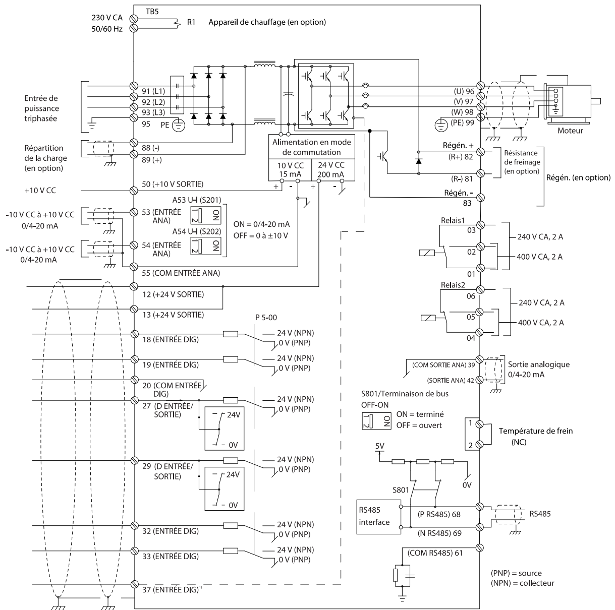
Illustration 17: Schéma de câblage de base
