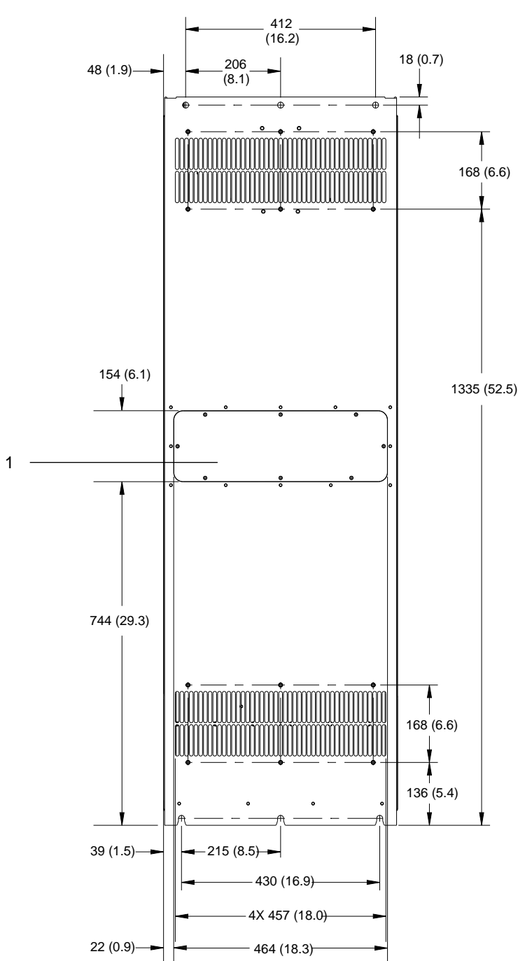
Illustration 62: Vue arrière du boîtier E3h
