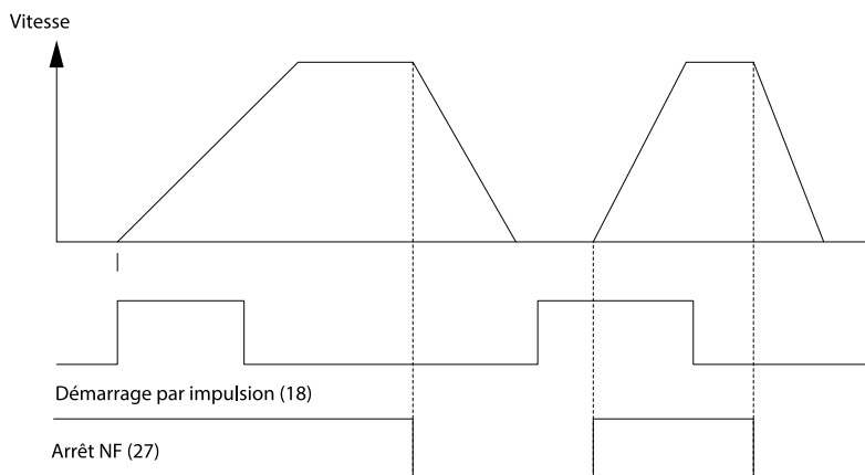
Illustration 41: Démarrage par impulsion/arrêt
