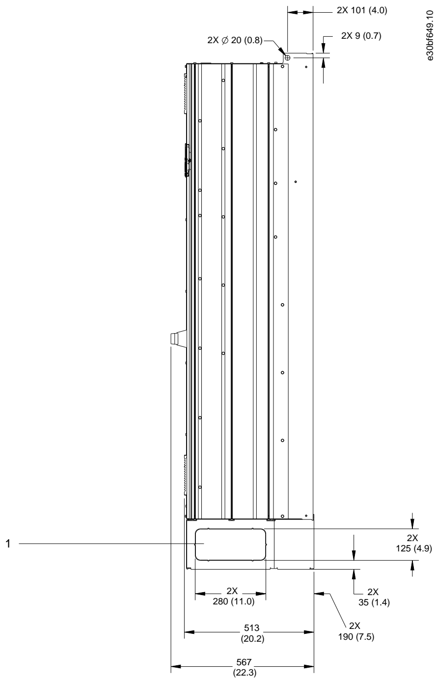
Illustration 53: Vue latérale du boîtier E1h
