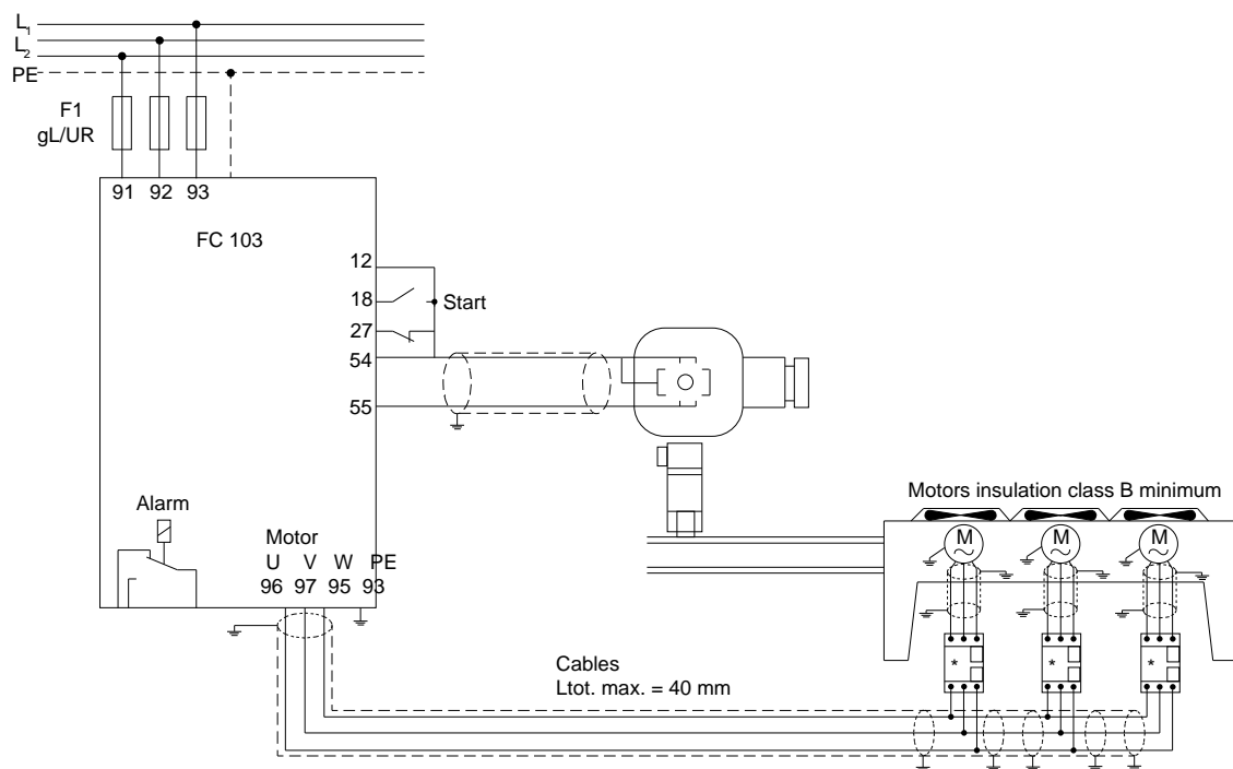
Illustration 44: Contrôle de pression en boucle fermée – Système autonome – Ventilateur ou pompe unique/ventilateurs ou pompes multiples en parallèle
