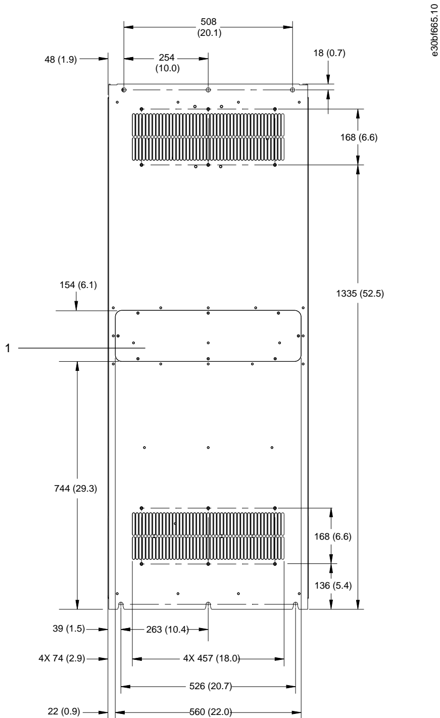
Illustration 66: Vue arrière du boîtier E4h
