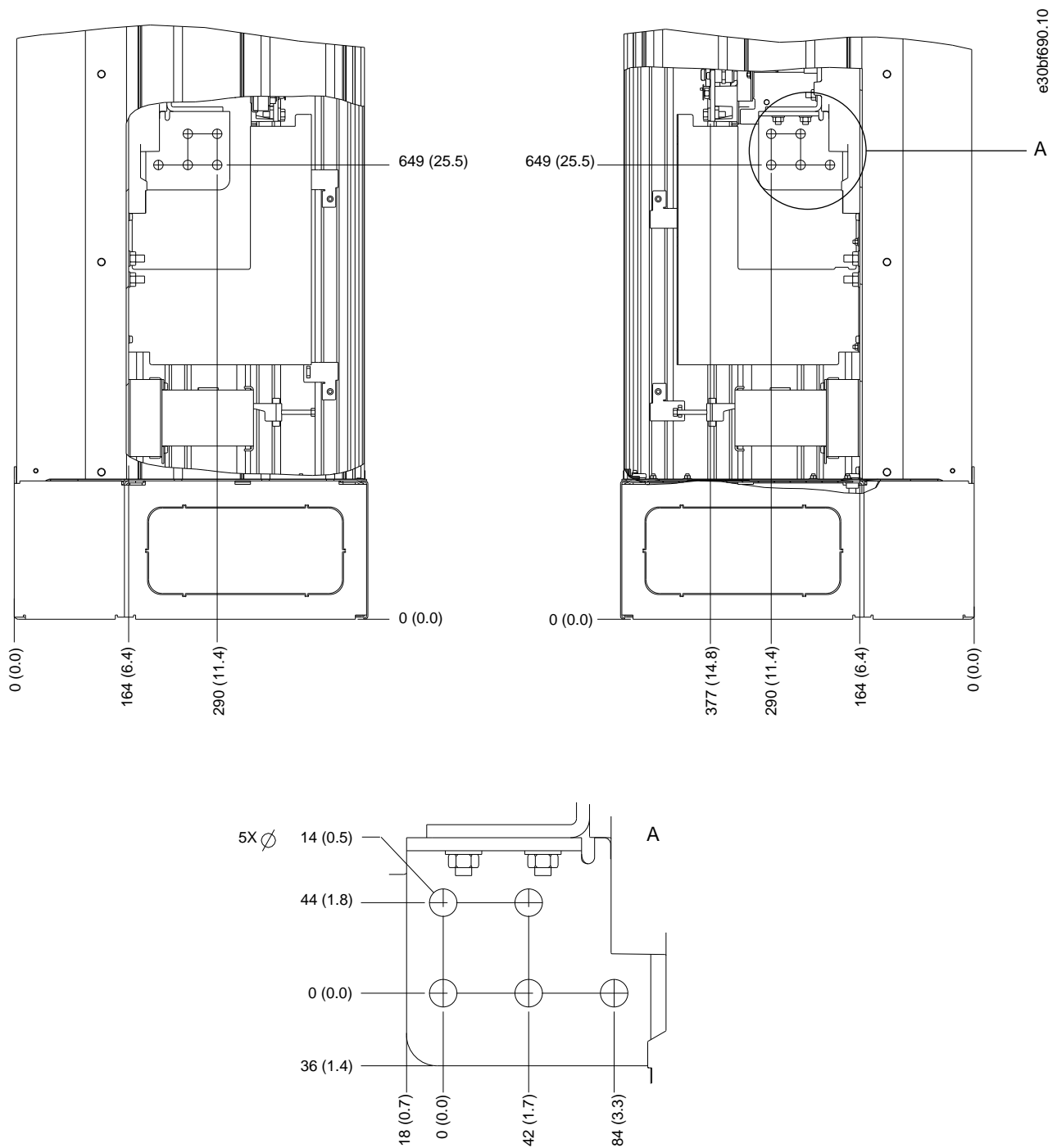
Illustration 24: Dimensions des bornes E2h (vues latérales)
