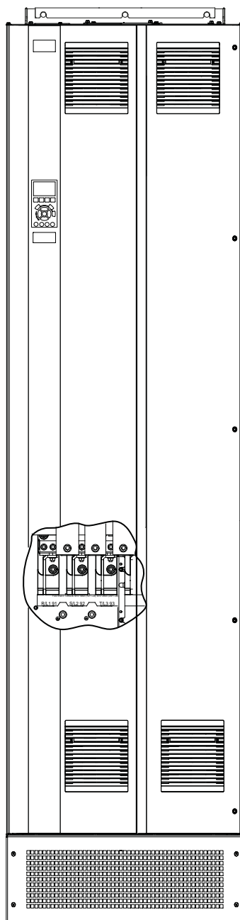
Illustration 19: Bornes réseau CA (E1h illustré).
