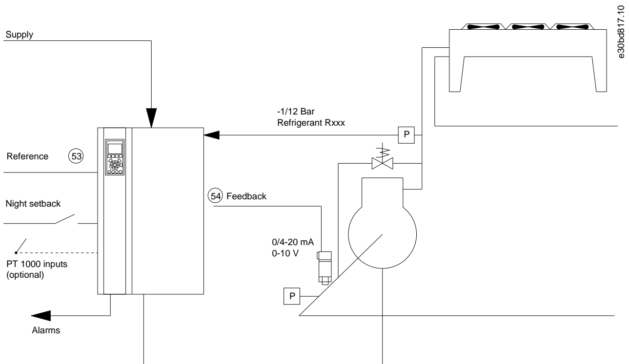
Illustration 42: Configuration standard du compresseur avec commande interne
