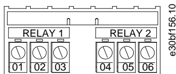
Illustration 34: Bornes des relais 1 et 2
