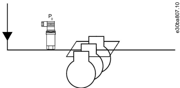
Illustration 45: Transmetteur de pression P 0
