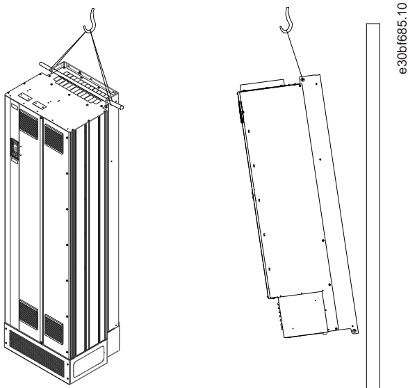
Illustration 8: Méthode de levage recommandée
