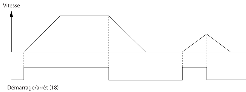
Illustration 40: Ordre de démarrage/arrêt avec Safe Torque Off
