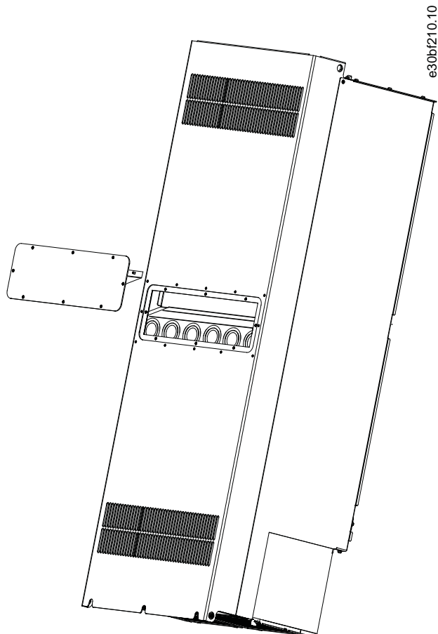
Illustration 47: Panneau d'accès au radiateur retiré de l'arrière du variateur
