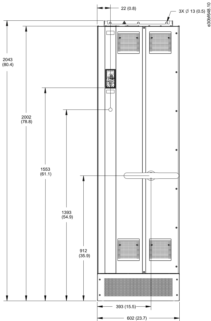
Illustration 52: Vue de face du boîtier E1h
