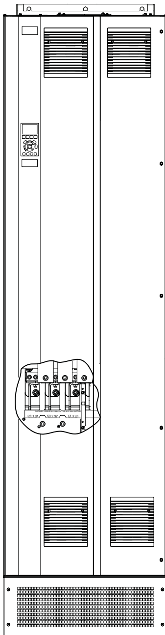
Ilustración 19: Terminales de red de CA (se muestra el alojamiento E1h).
