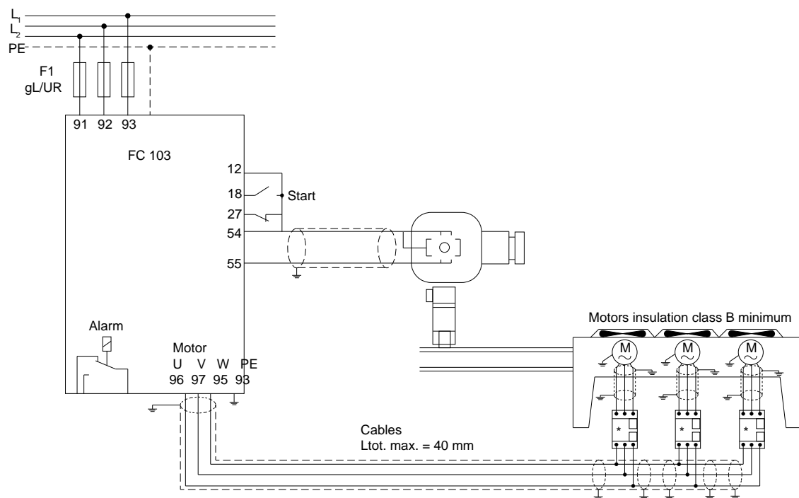
Ilustración 44: Control de presión de lazo cerrado. Sistema independiente. Bomba o ventilador único, o varios ventiladores o bombas en paralelo
