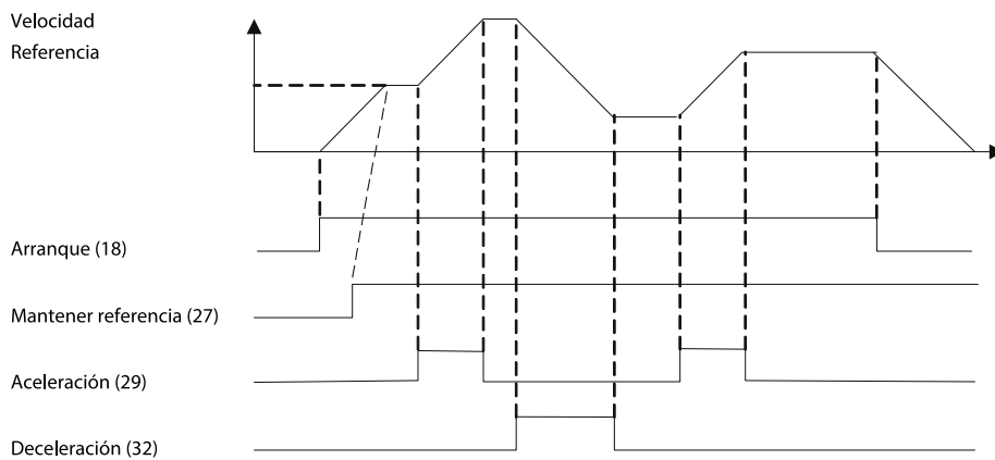
Ilustración 39: Aceleración/deceleración
