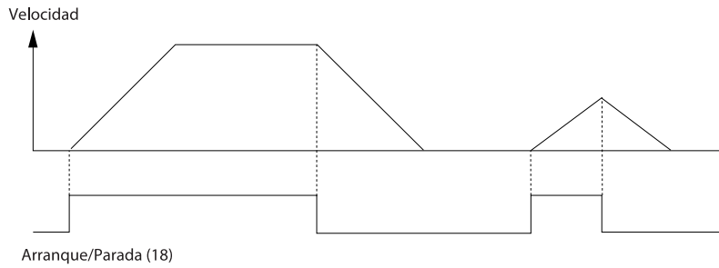
Ilustración 40: Orden de arranque/parada con Safe Torque Off
