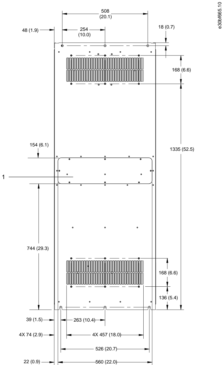
Ilustración 66: Vista posterior del alojamiento E4h
