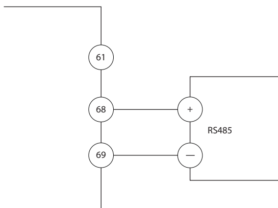
Ilustración 37: Diagrama de cableado de comunicación serie
