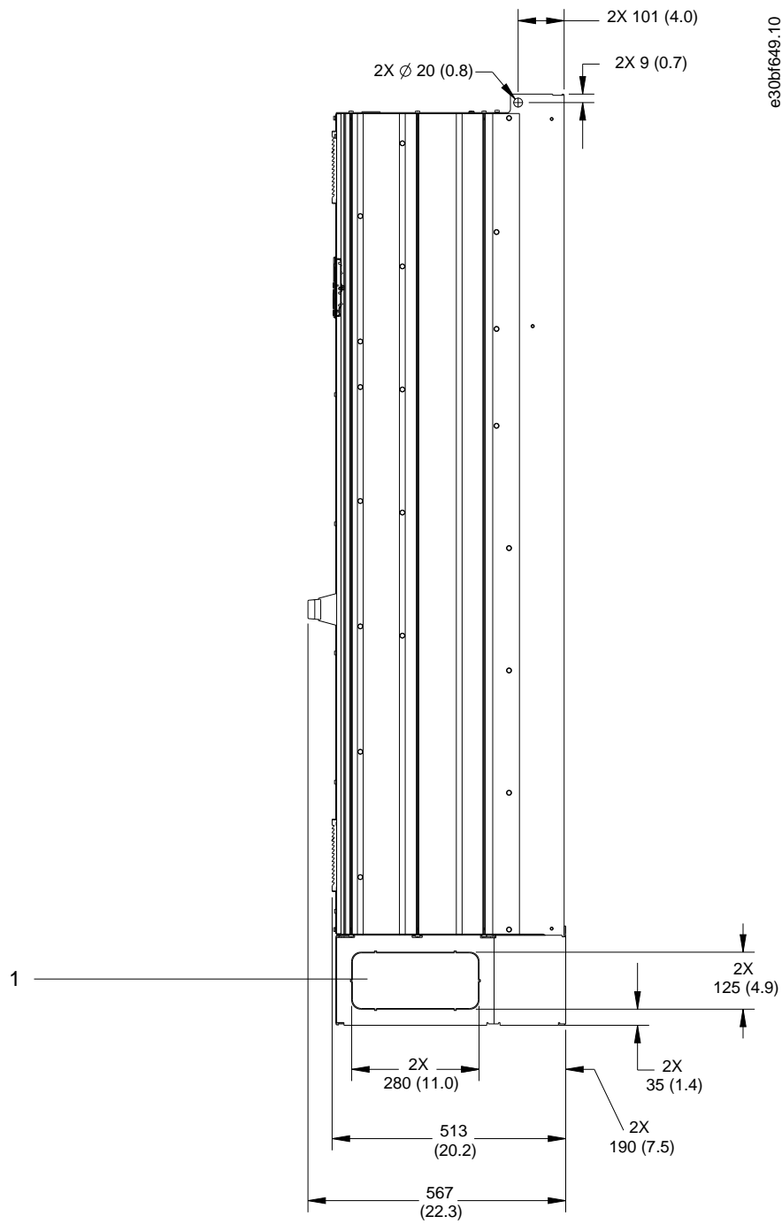
Ilustración 53: Vista lateral del alojamiento E1h
