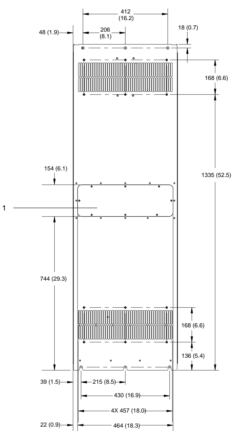
Ilustración 62: Vista posterior del alojamiento E3h
