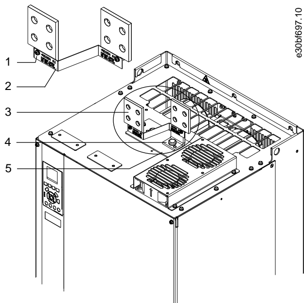
Illustrazione 15: Morsetti Regen/condivisione del carico
