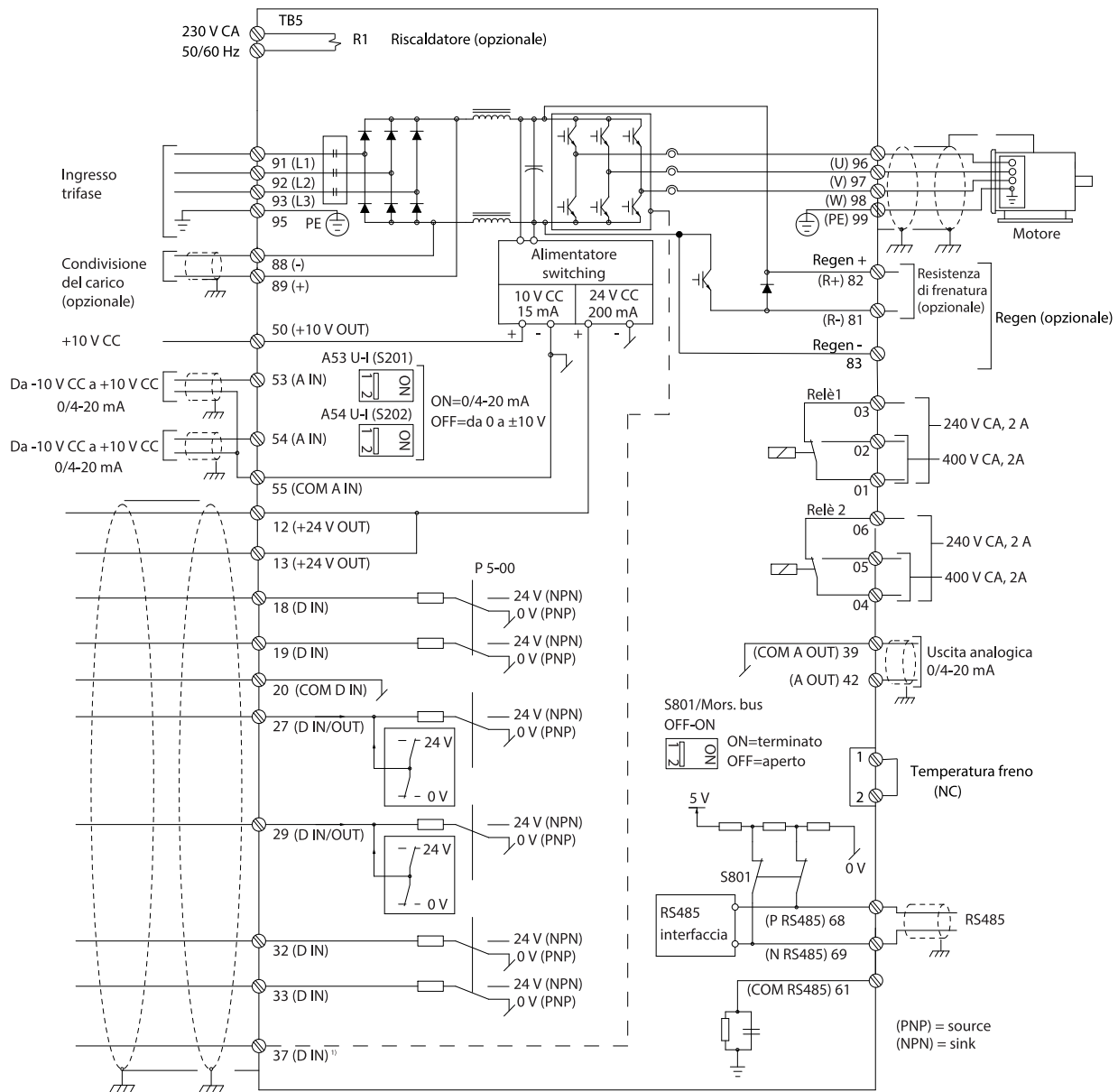
Illustrazione 17: Schema di cablaggio di base
