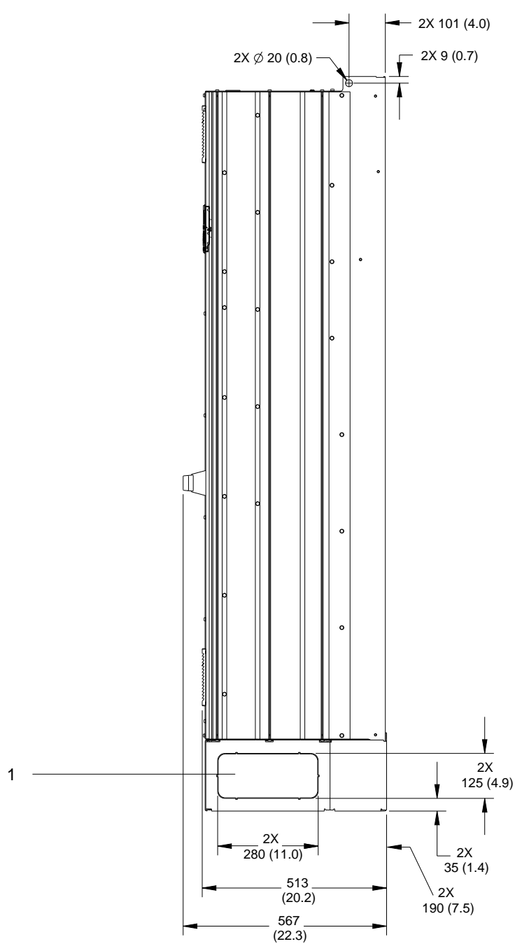
Illustrazione 57: Vista laterale dell'unità E2h
