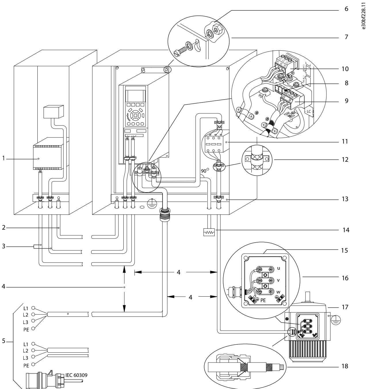
Illustrazione 16: Esempio di installazione EMC corretta
