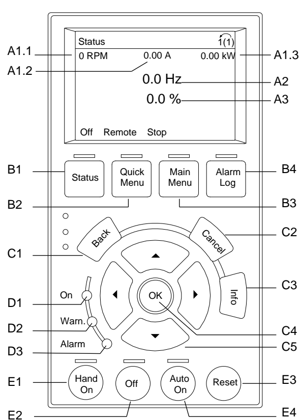
Illustrazione 5: Pannello di Controllo Locale (LCP) grafico
