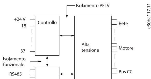
Illustrazione 51: Isolamento PELV
