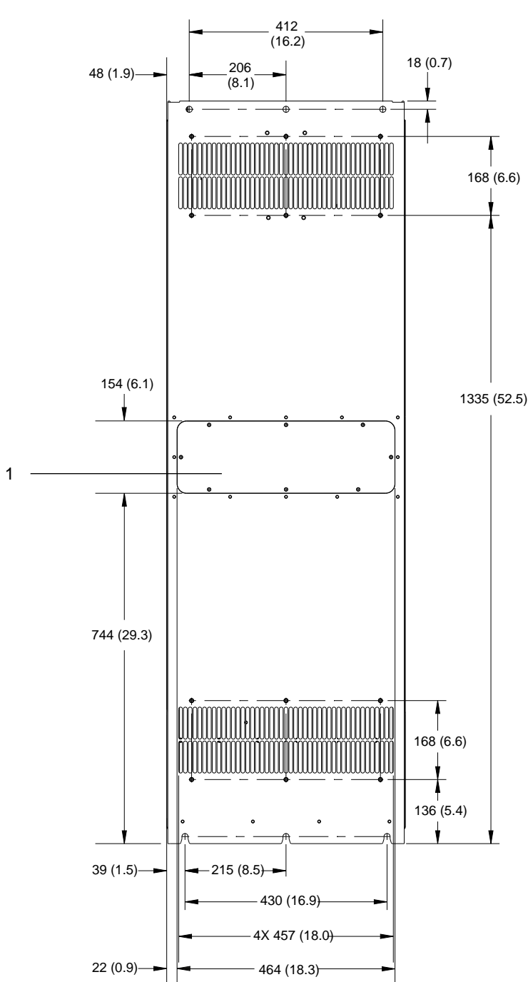
Ilustração 62: Vista traseira do E3h
