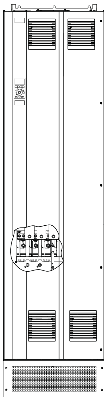
Ilustração 19: Terminais de rede elétrica CA (E1h mostrado).
