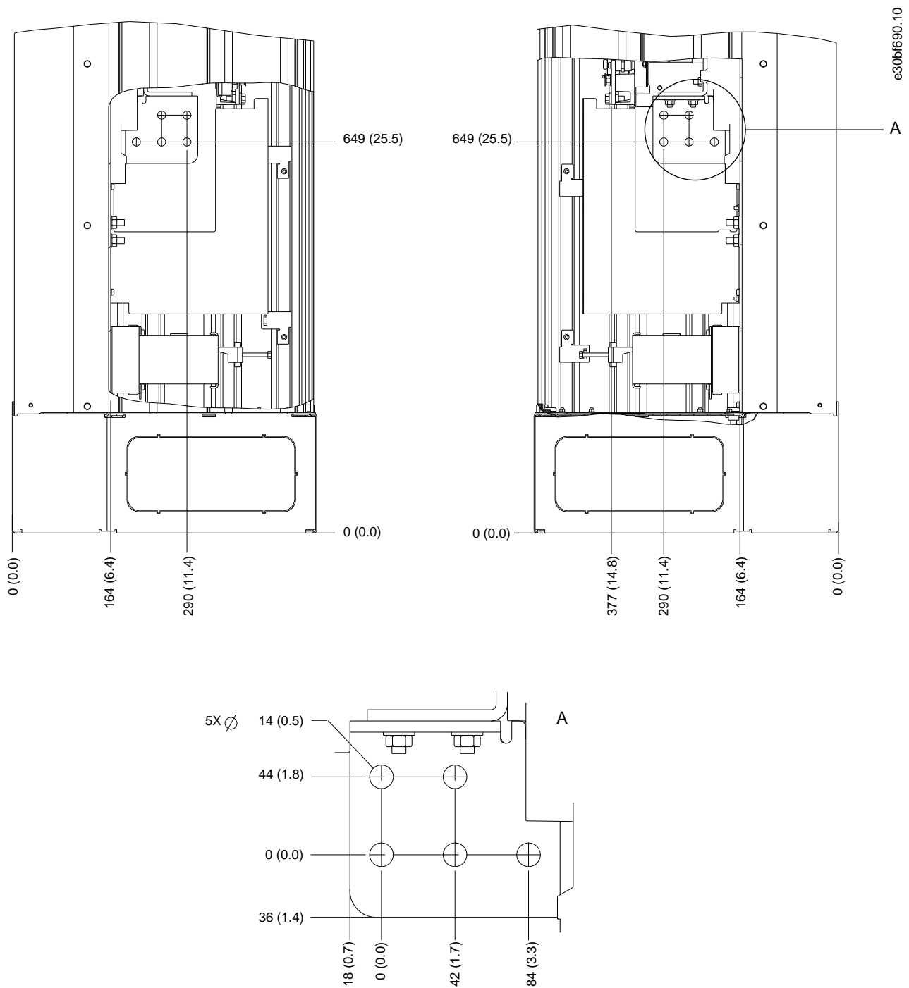
Ilustração 24: Dimensões dos terminais do E2h (vistas laterais)
