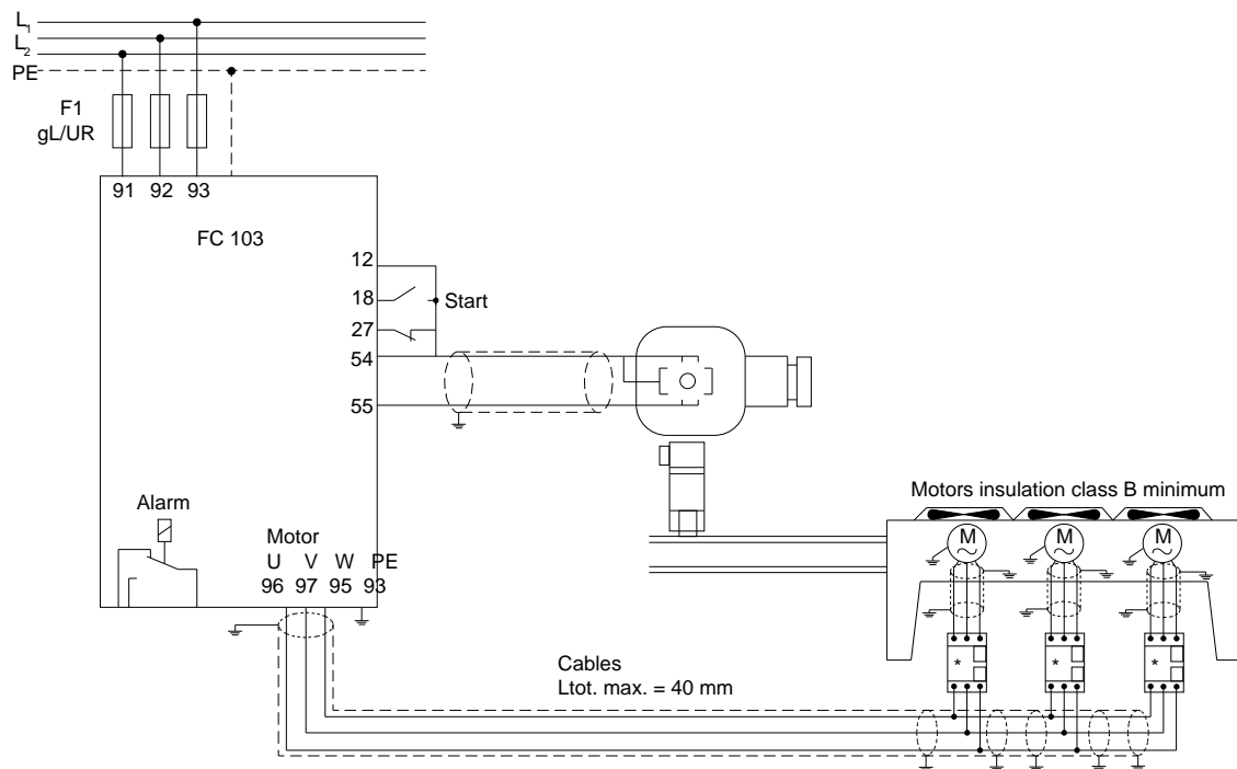
Рисунок 44: Регулирование давления в замкнутом контуре — изолированная система — одиночный вентилятор или насос/ несколько вентиляторов или насосов, подключенных параллельно
