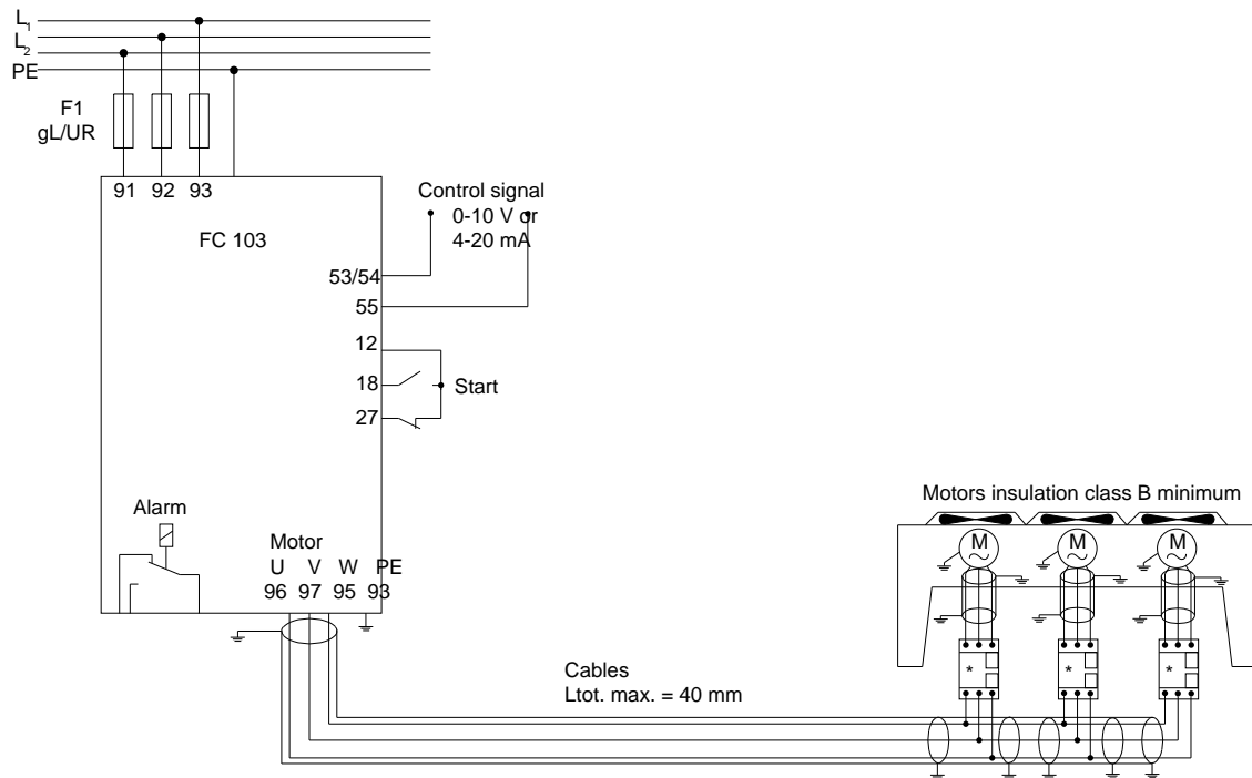
Рисунок 43: Регулирование скорости с использованием аналогового задания (разомкнутый контур) — один вентилятор или насос/ несколько вентиляторов или насосов, подключенных параллельно
