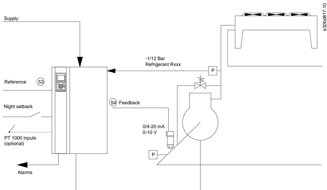
Рисунок 42: Стандартная конфигурация компрессора с внутренним управлением
