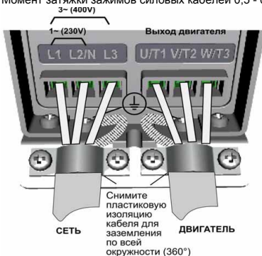
Рисунок 3: Подключение силовых кабелей преобразователя Vacon 10, MI1
