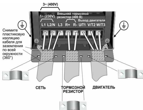
Рисунок 4: Подключение силовых кабелей преобразователя Vacon 10, MI2-MI3
