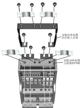
图 2: 附加 PE 板和 API 电缆支架
