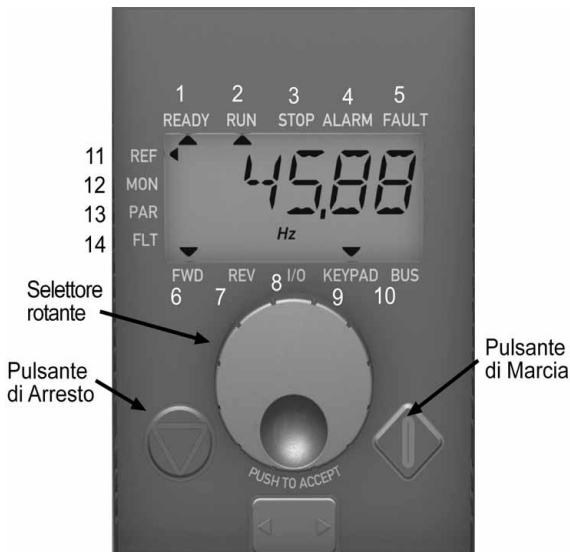
Figura 7.1: Pannello di controllo Vacon10
