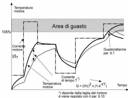
Figura 9.9: Calcolo dell'immagine termica del motore.
