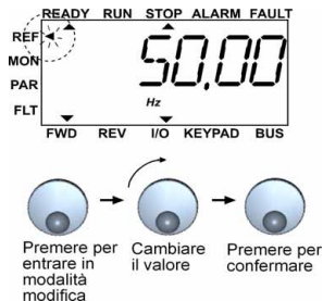
Figura 7.3: Menù Riferimento da Pannello
