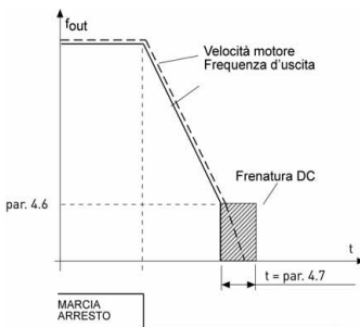
Figura 9.6: Tempo di frenatura DC con la funzione di Arresto = Rampa.
