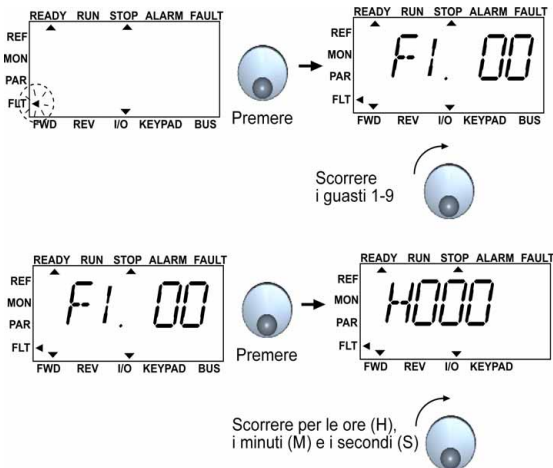
Figura 7.6: Menù Memoria Guasti
