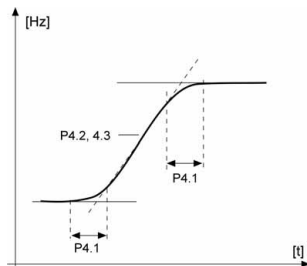
Figura 9.3: Accelerazione/decelerazione a S.
