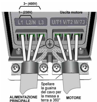
Figura 3.4: Vacon 10 collegamenti di potenza, MI1
