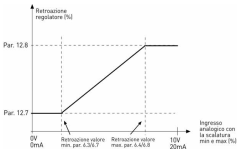
Figura 9.11: Valori minimo e massimo retroazione
