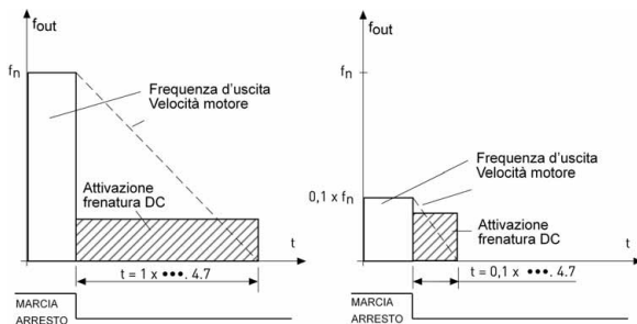
Figura 9.5: Tempo di frenatura DC con la funzione di Arresto = Arresto per inerzia.
