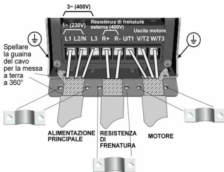
Figura 3.5: Vacon 10 collegamenti di potenza, MI2 - MI3
