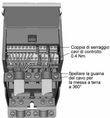
Figura 3.8: Installare i cavi di controllo. Si veda il capitolo 6.2
