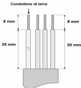
Figura 3.9: Spelatura dei cavi
