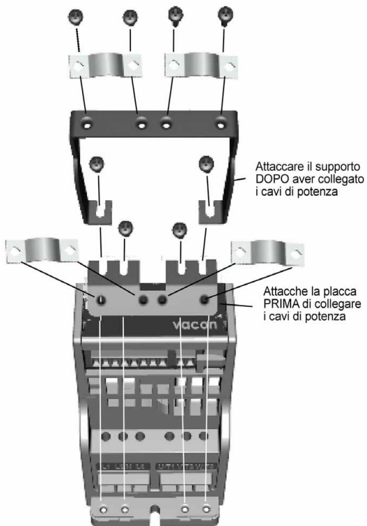
Figura 3.6: Connessione della placca di messa a terra e del supporto cavi.
