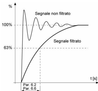
Figura 9.7: Filtraggio dei segnali AI1 e AI2
