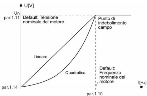
Figura 9.1: Variazione lineare e quadratica della tensione del motore.
