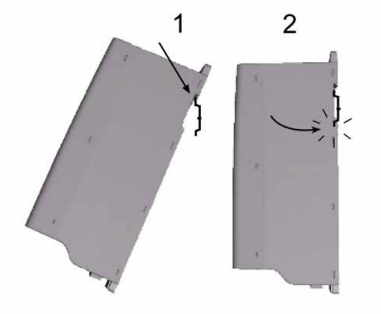
Figura 3.2: Montaggio su guida DIN
