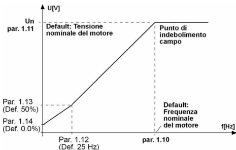
Figura 9.2: Curva V/f programmabile
