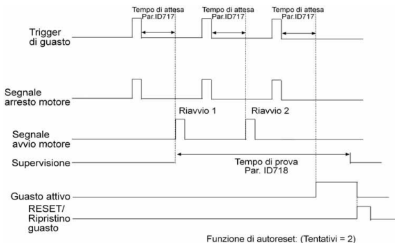
Figura 9.10: Riavviamento automatico.
