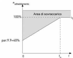
Figura 9.8: Capacità di raffreddamento del motore
