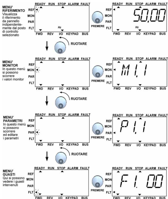
Figura 7.2: Il Menù Principale di Vacon 10
