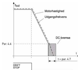
Figur 9.6: DC-bremsetid, når stoptilstand = rampe
