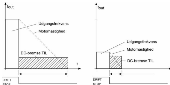
Figur 9.5: DC-bremsetid, når stoptilstand = friløb
