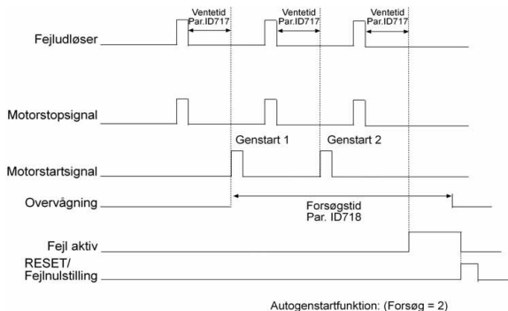
Figur 9.10: Automatisk genstart
