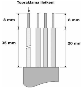
Şekil 3.9: Kabloları soyma
