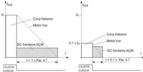
Şekil 9.5: Durdurma modu = Serbest duruş olduğunda DC frenleme süresi
