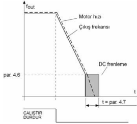
Şekil 9.6: Duruş modunda DC frenleme = rampalı
