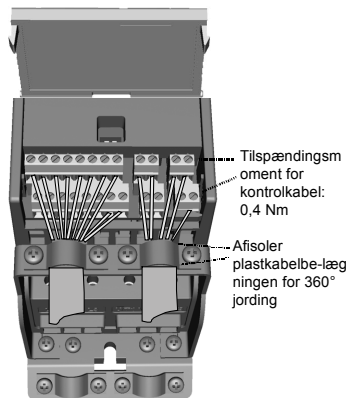
Figur 2.7: Monter net- og motorkablerne, MI1-MI3
