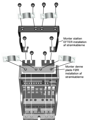
Figur 2.3: Fastgørelse af PE-pladen og API-kabelstøtten, MI1-MI3
