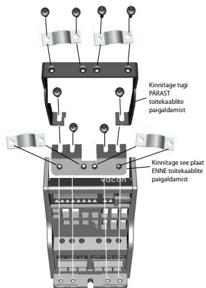
Joonis 2.3: PE-plaadi ja API kaablite kinnitamine, MI1 kuni MI3
