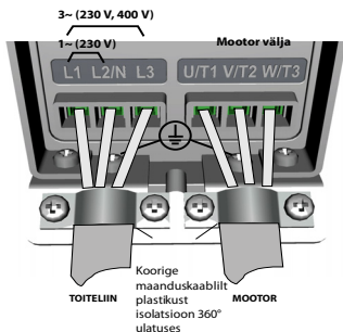
Joonis 2.4: Vacon 10 toiteühendused, MI1
