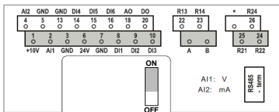
Joonis 3.1: Vacon 10 I/O
