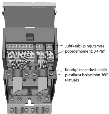
Joonis 2.7: Paigaldage juhtkaablid, MI1 kuni MI3
