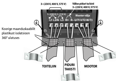
Joonis 2.5: Vacon 10 toiteühendused, MI2 ja MI3
