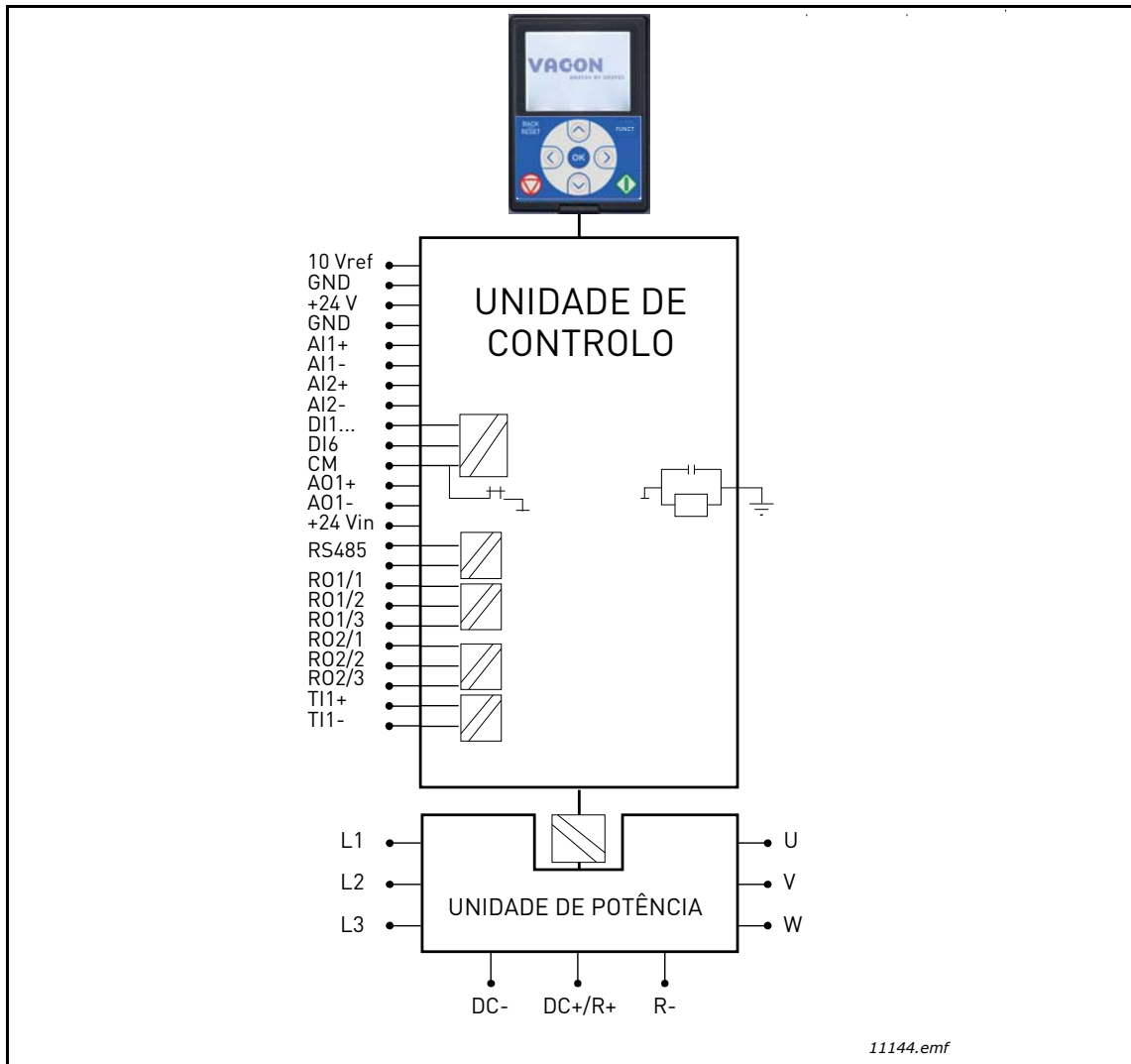
Figura 60. Barreiras galvânicas de isolamento
