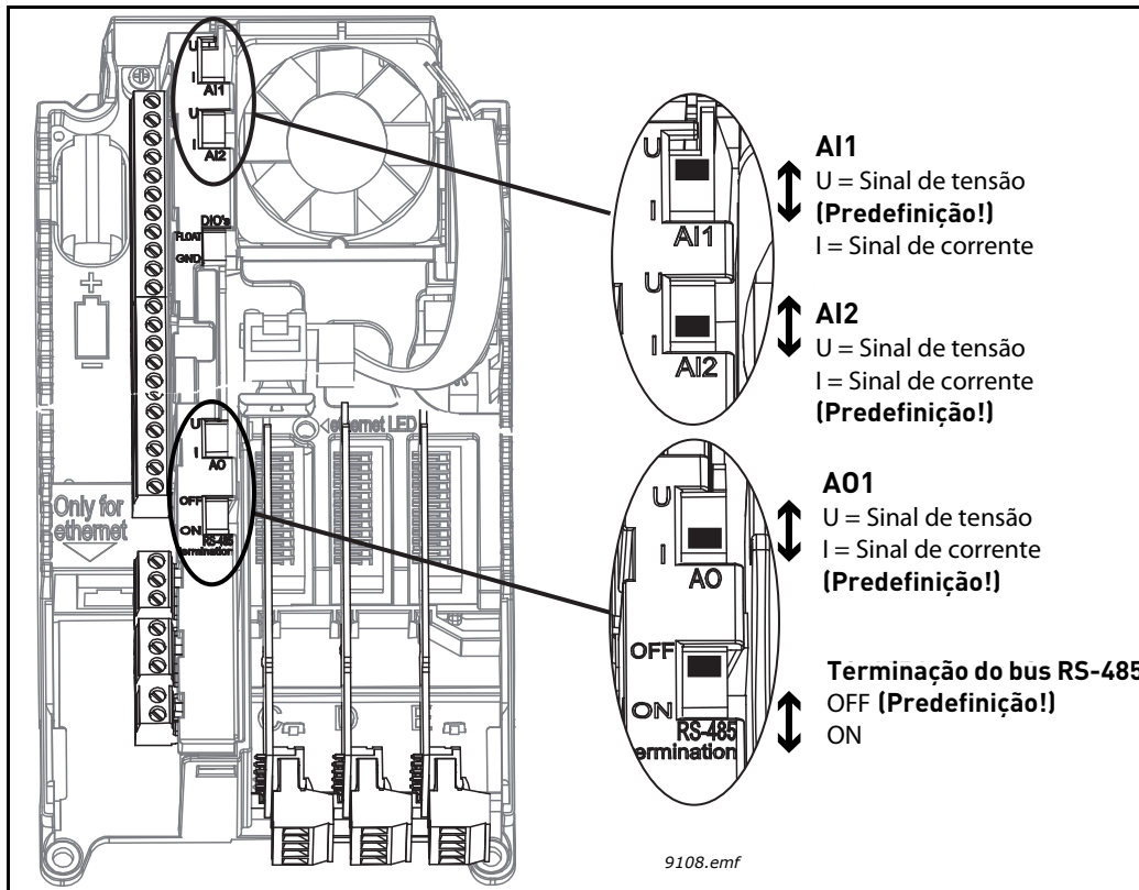
Figura 53. Interruptores DIP
