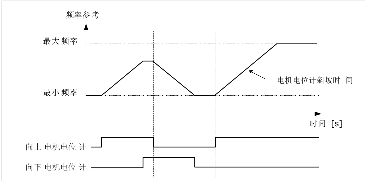
图 37: 电机电位计参数
