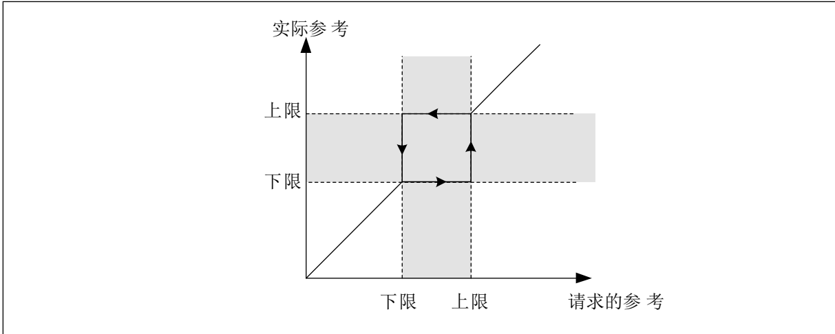
图 53: 禁止的频率
