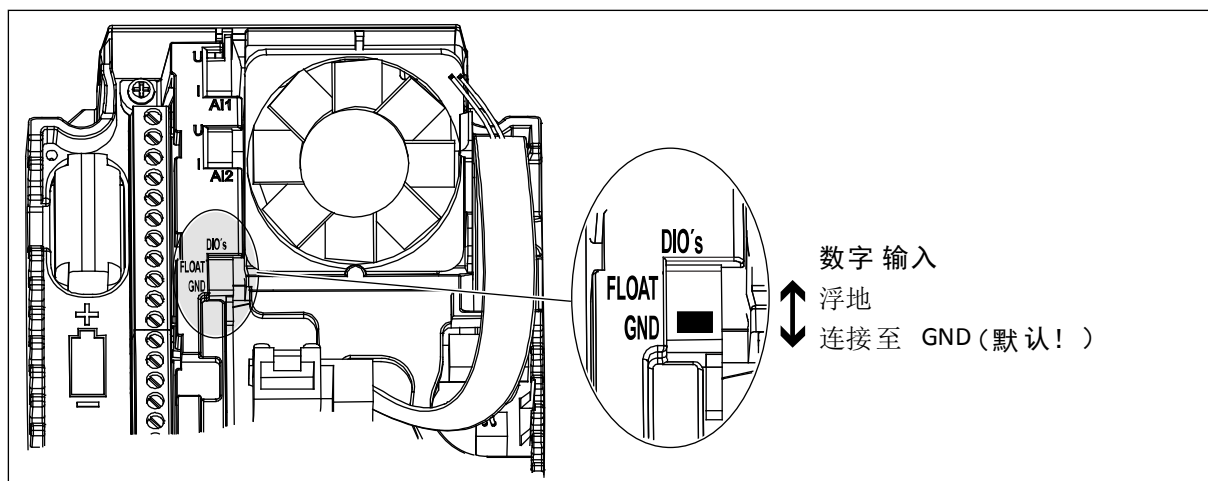
图 15: DIP 开关
