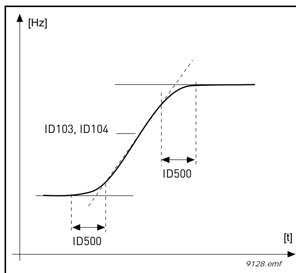
Figura 46. Accelerare/decelerare (în formă de S)
