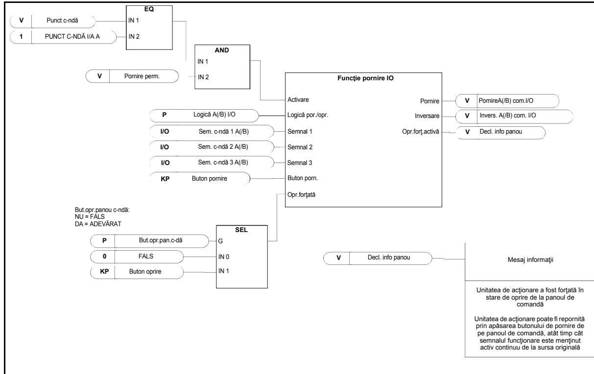
Figura 37. Logică de pornire/oprire I/O A, schemă bloc
