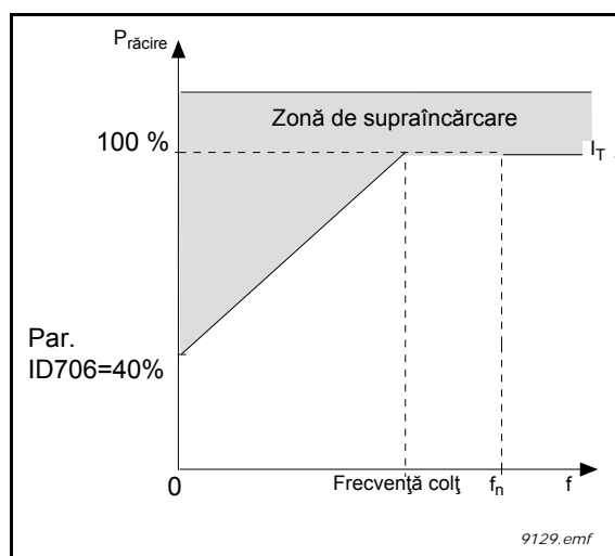
Figura 56. Curba curentului termic I_T al motorului
