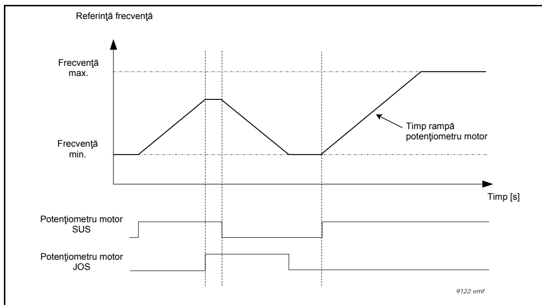
Figura 44. Parametri potențiomtru motor
