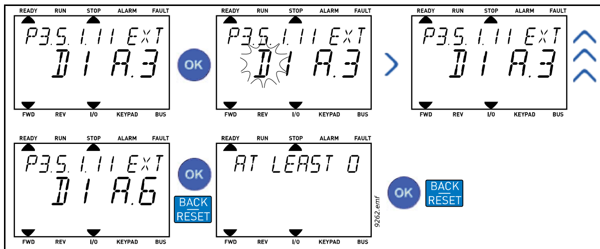
Figura 20. Programarea intrărilor digitale cu panoul de comandă text
