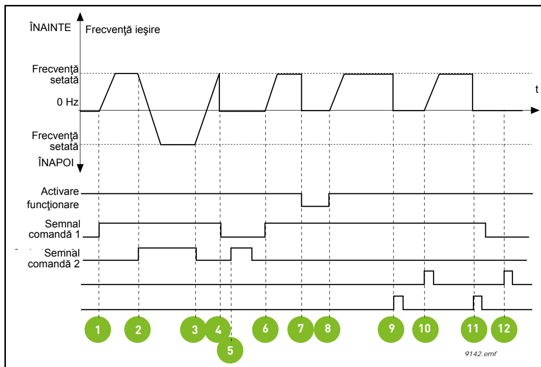
Figura 41. Logică pornire/oprire I/O A = 3
