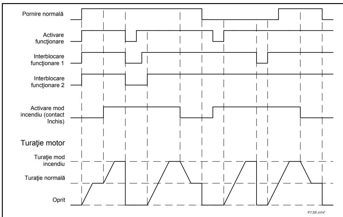
Figura 78. Funcționarea modului incendiu
