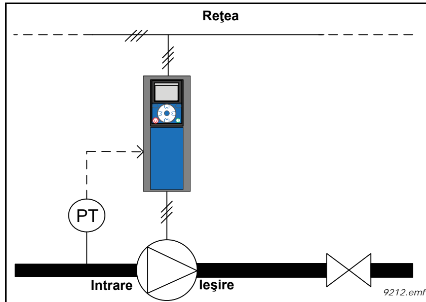
Figura 30. Loc de amplasare a senzorului de presiune
