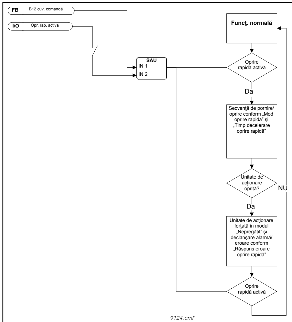
Figura 62. Logica de oprire rapidă
