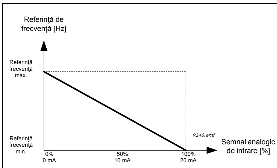
Figura 52. Inversiune semnal AI, selectare „1”
