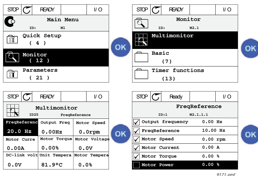
Figura 16. Pagina de supraveghere multiplă
