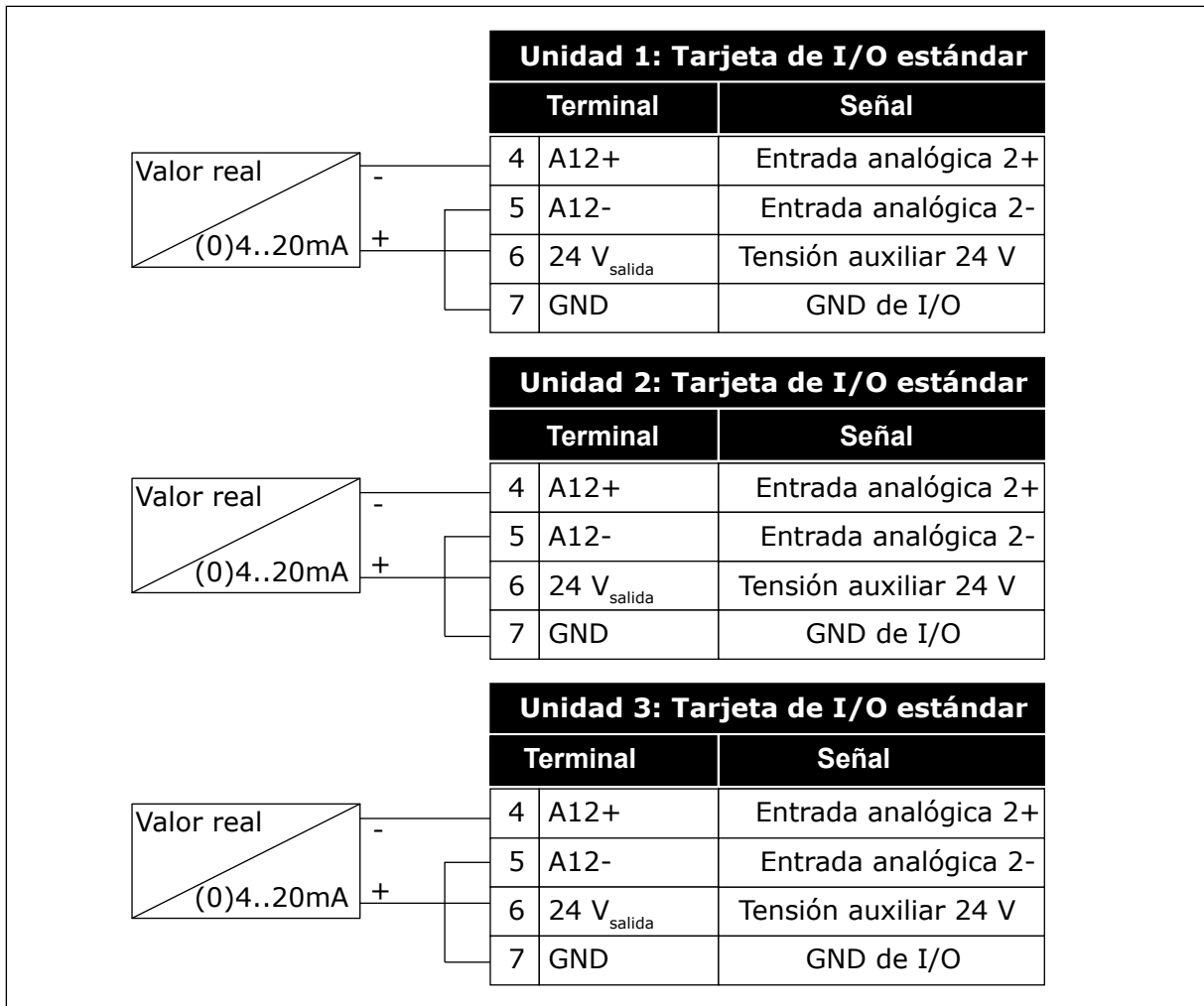
Imag. 94: Cableado de los sensores de valor actual para cada convertidor
