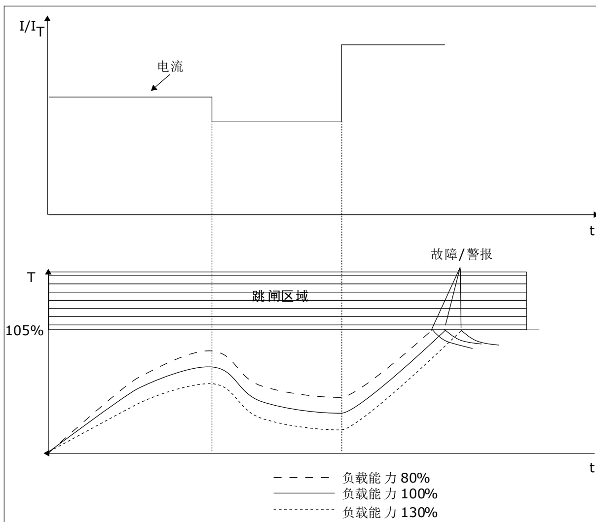
图 66: 电机温度的计算
