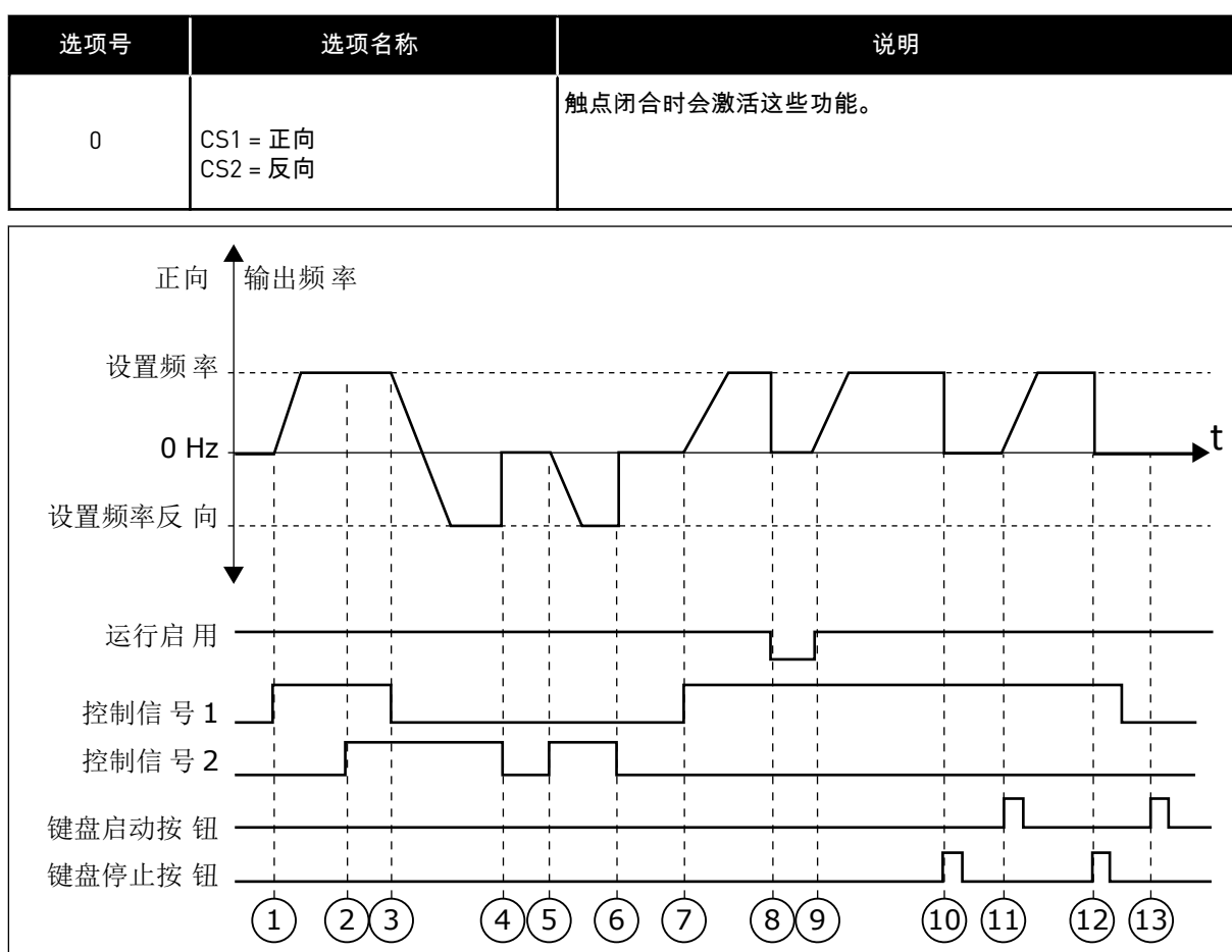
图 42: I/O A 启动/停止逻辑 = 0
