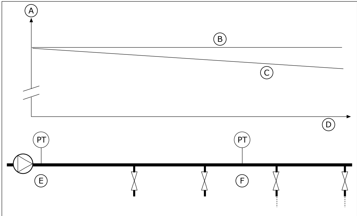
图 84: 压力传感器的位置
