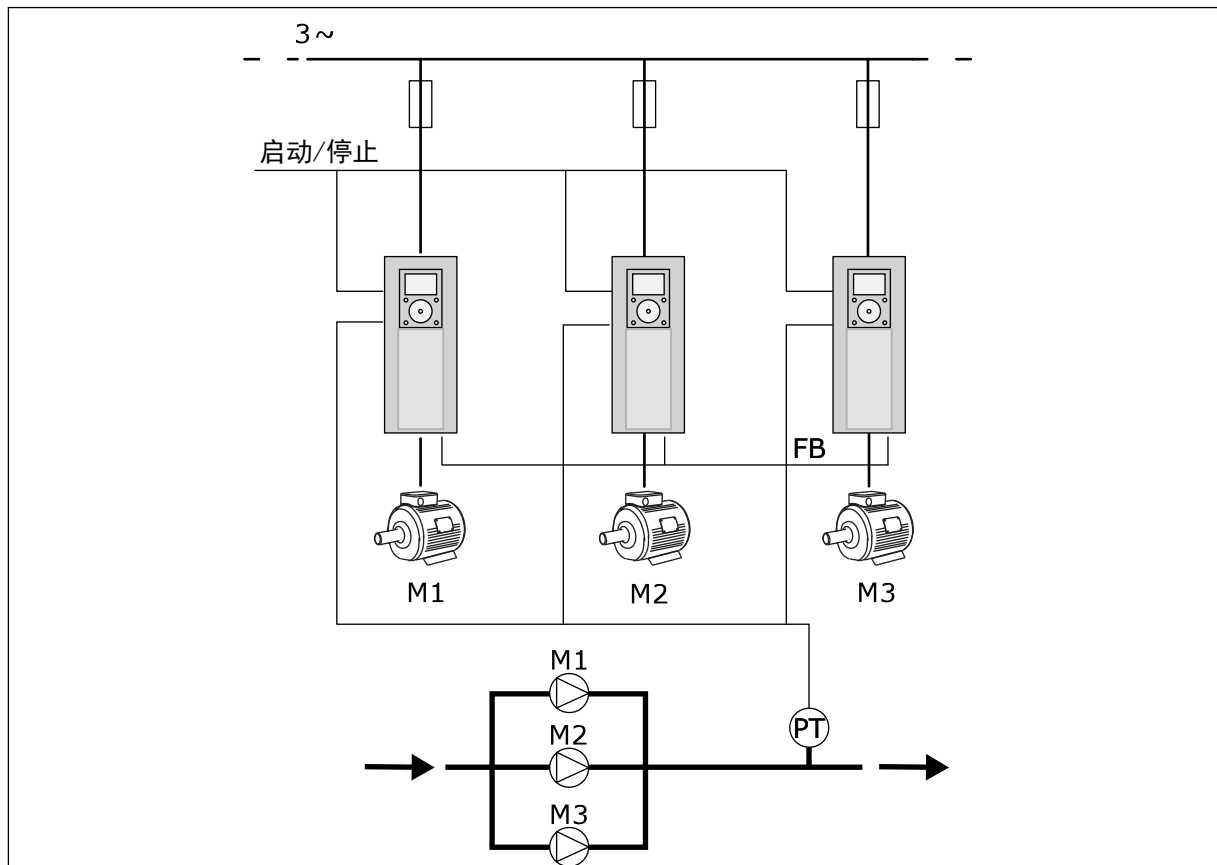
图 13: 多泵（多变频器）配置
