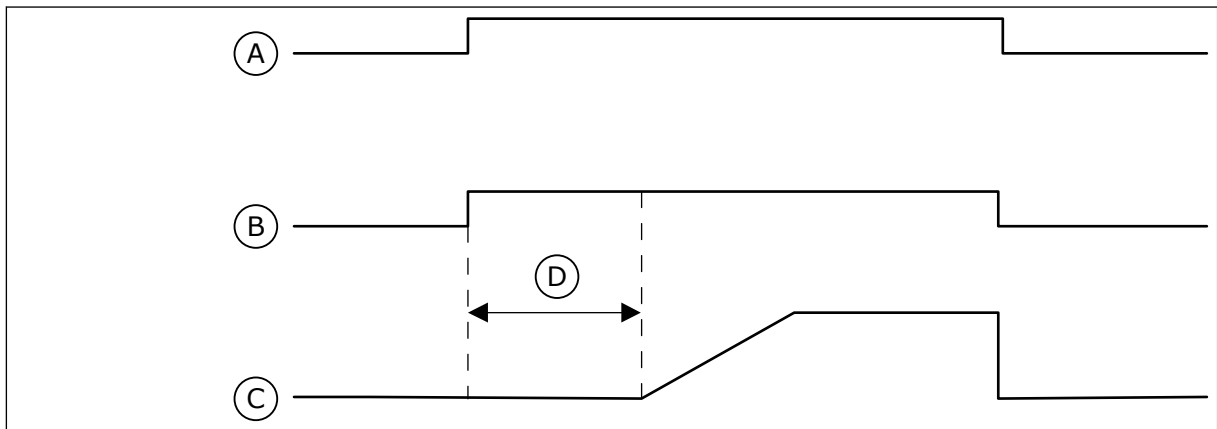
图 106: 注给泵功能
