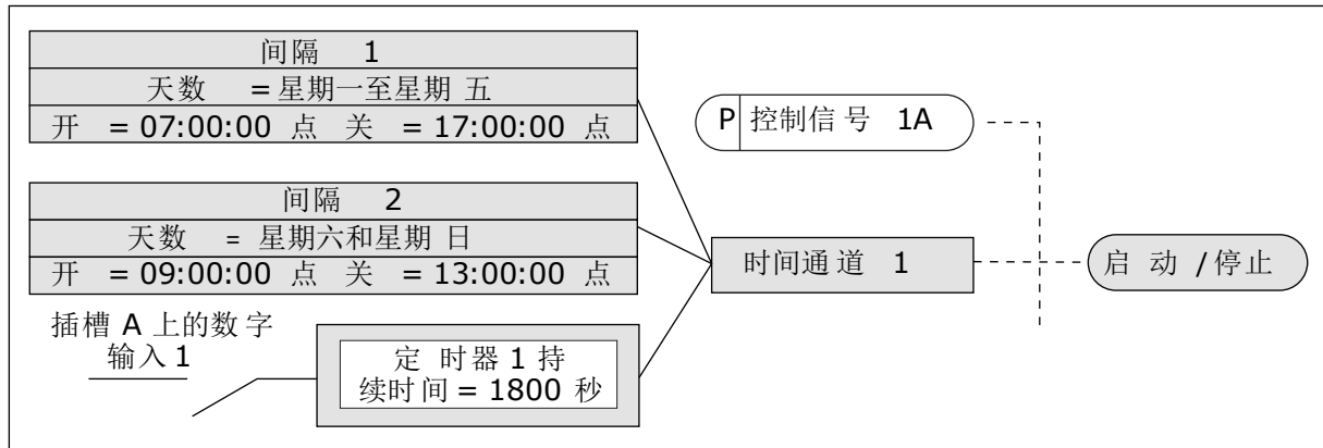
图 78: 时间通道 1 ( 而非数字输入 ) 用作启动命令的控制信号
