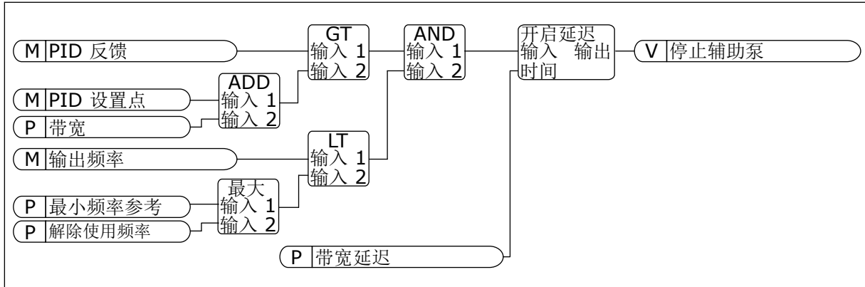
图 102: 降级频率
