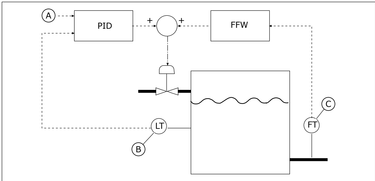
图 80: 前馈控制
