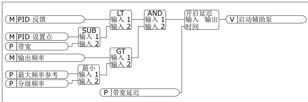
图 101: 分级频率
