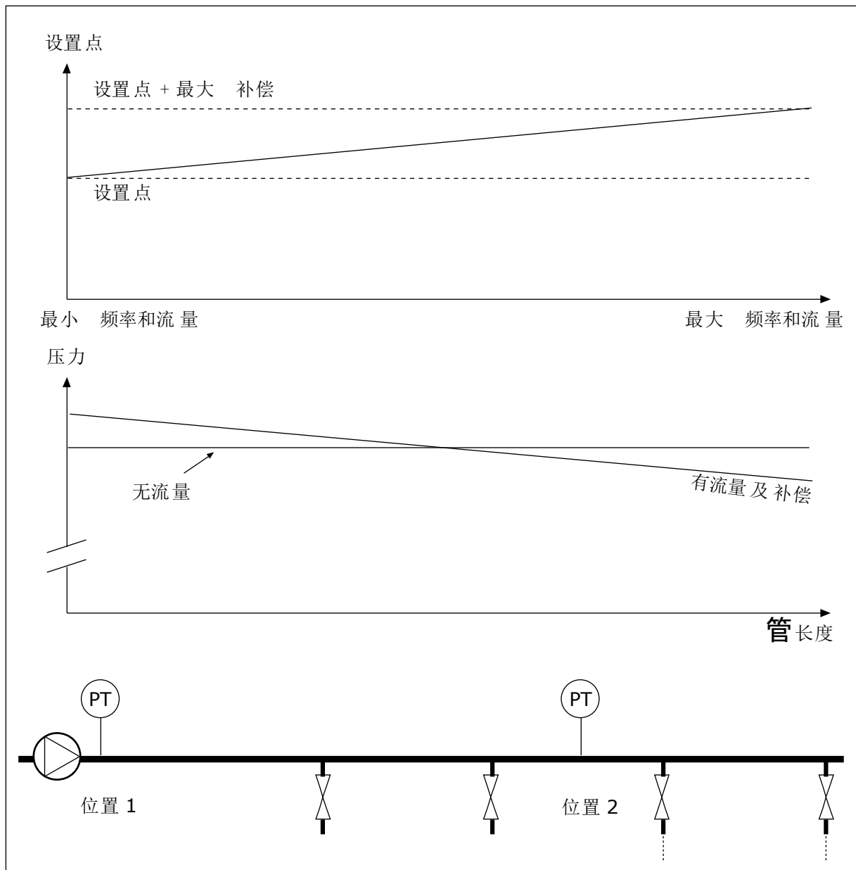
图 85: 压力损失补偿的启用设置点 1
