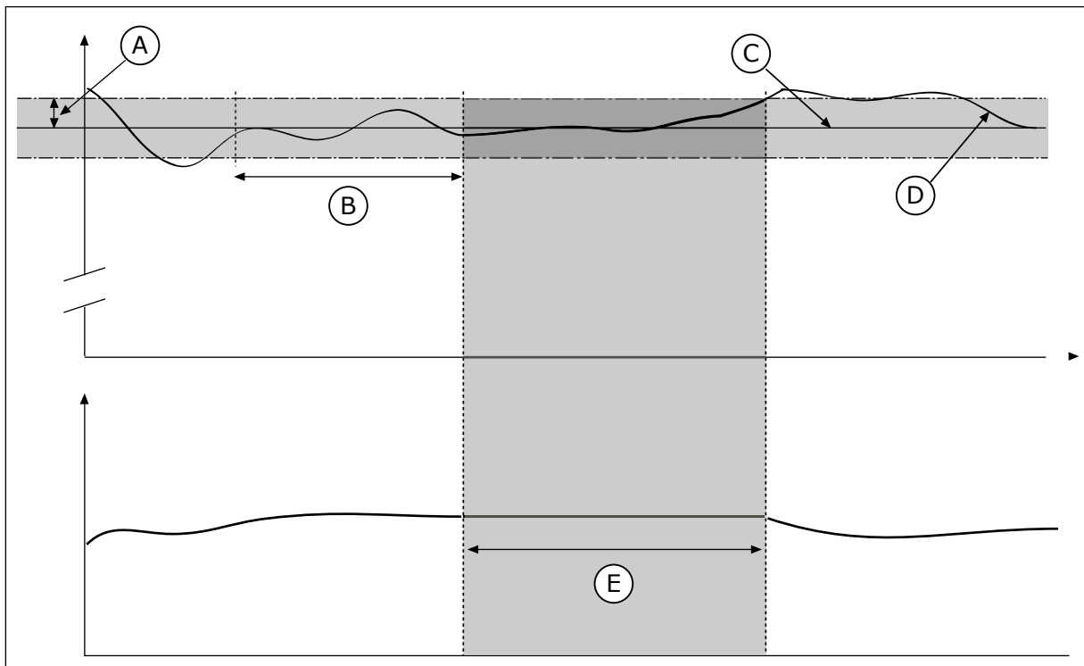
图 79: 死区功能
