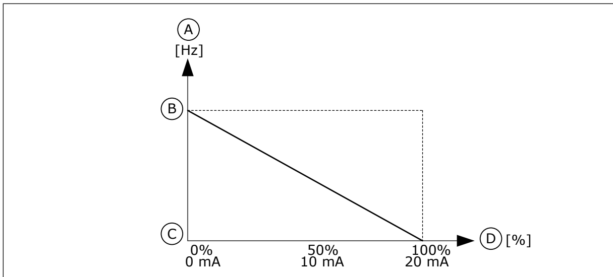
图 61: A11 信号反演, 选项 1
