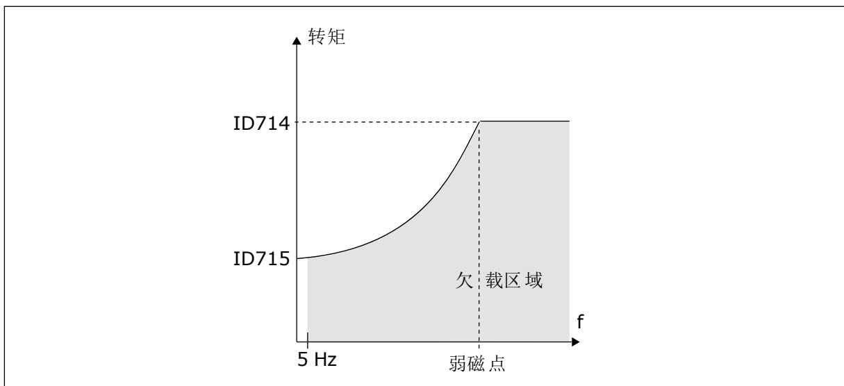
图 69: 设置最小负载
