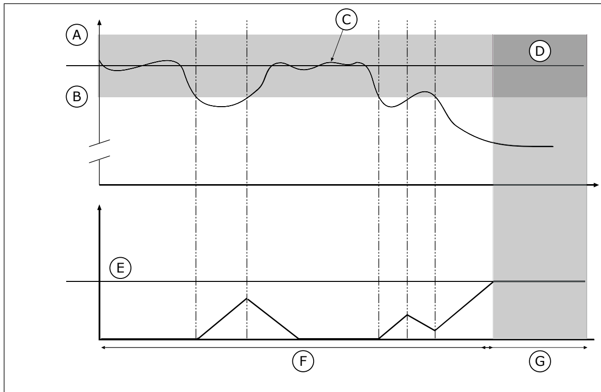
图 83: 反馈监控功能
