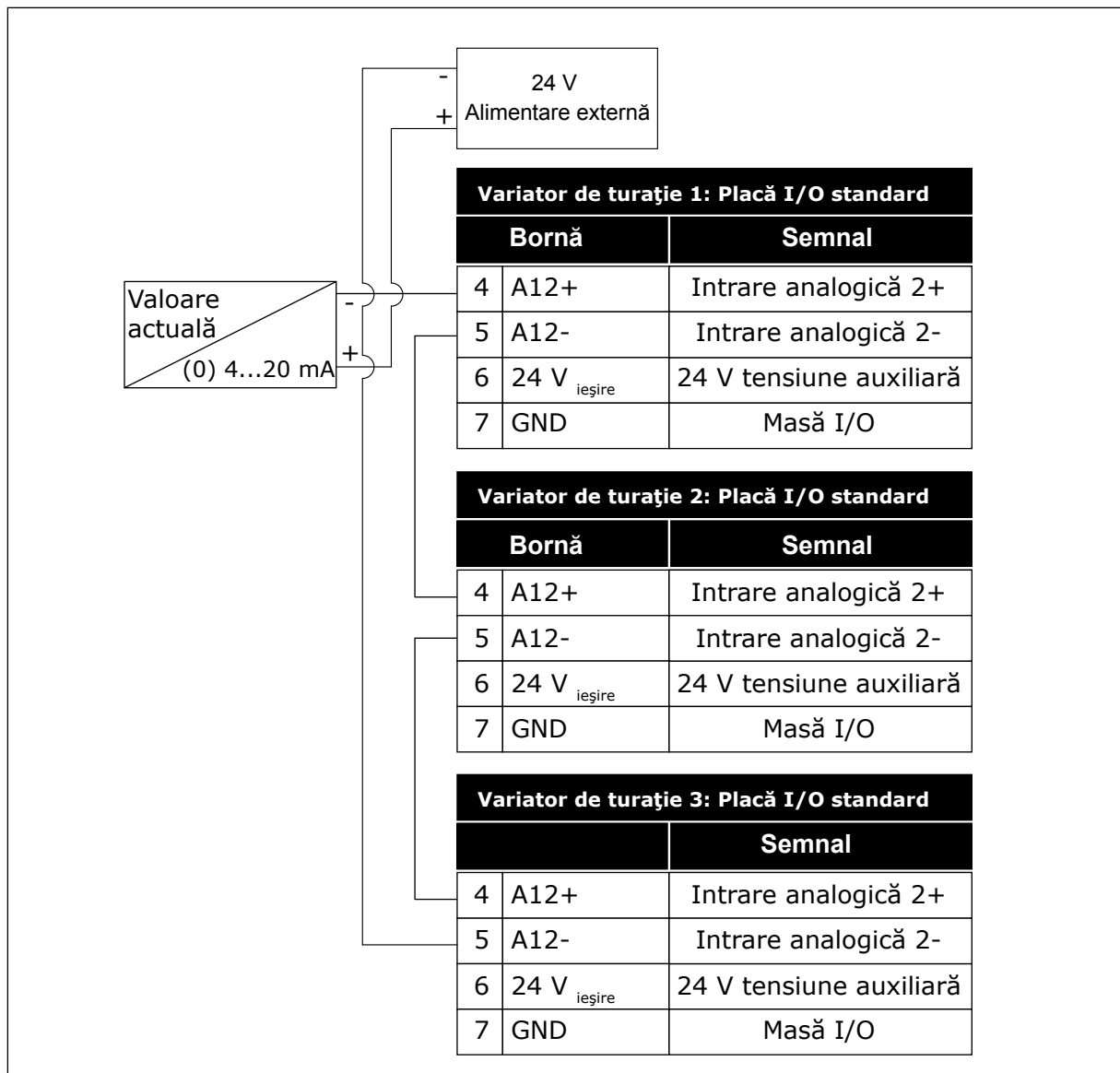
Fig. 96: Cablarea aceluiași senzor pentru toate variatoarele de turație (alimentat de la o sursă externă de 24 V)
