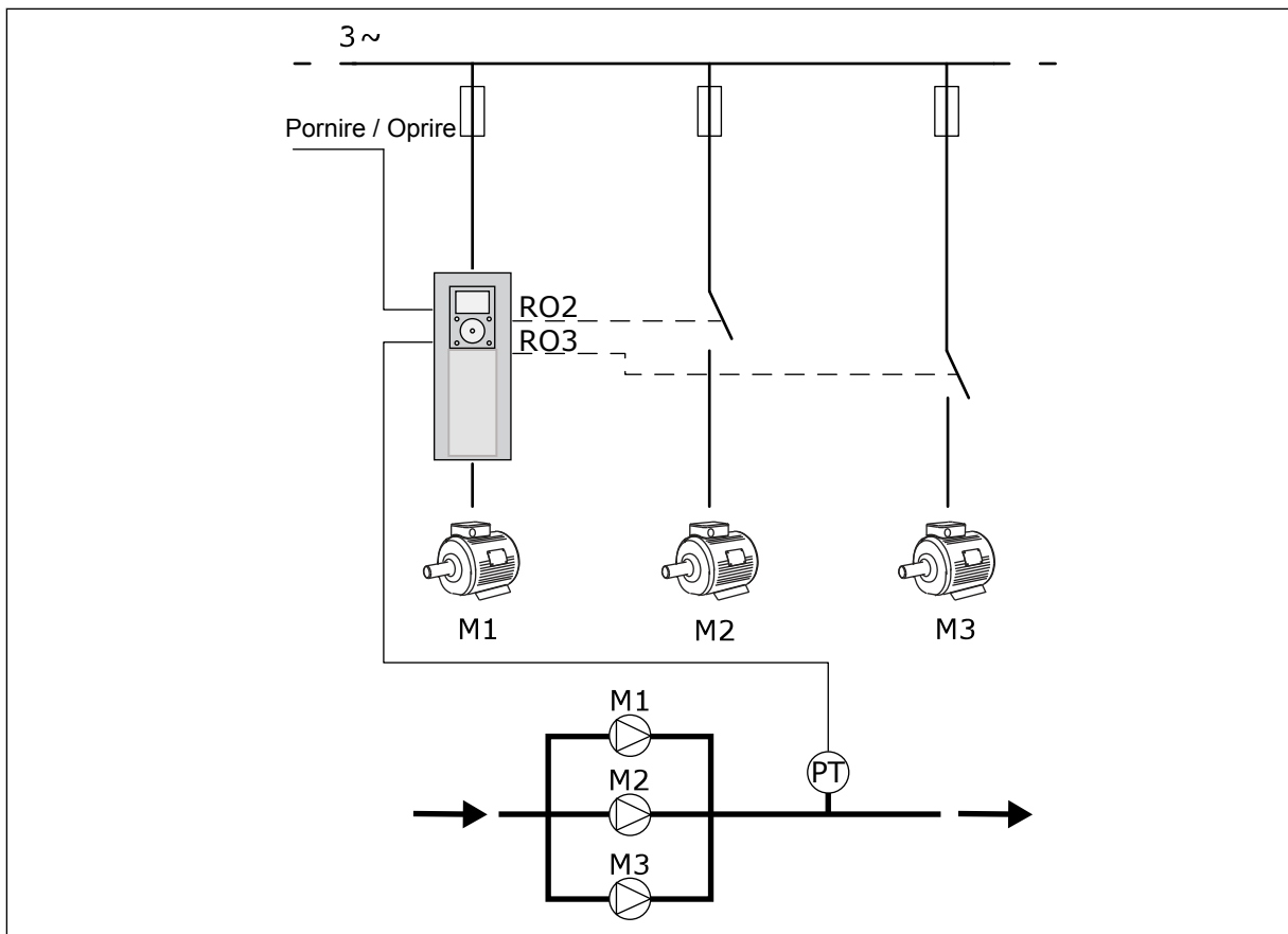
Fig. 8: Configurarea Pompe multiple (acționare simplă)
