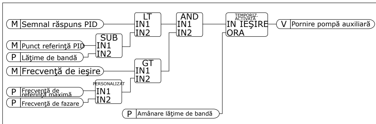
Fig. 101: Switching Frequency (Frecvență de fazare)
