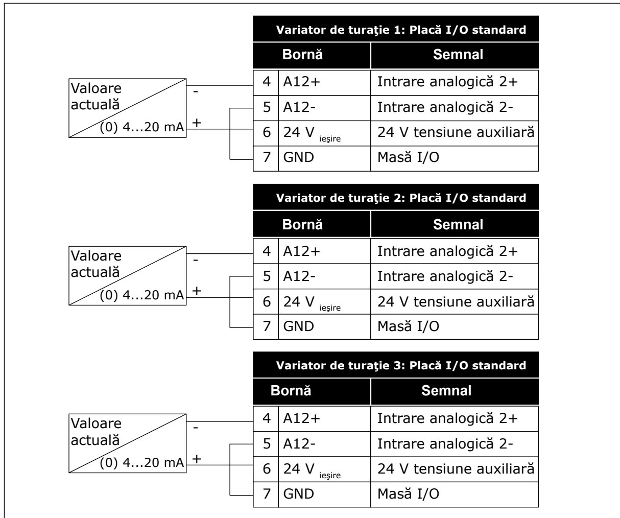
Fig. 94: Cablarea senzorilor de feedback pentru fiecare variator de turație
