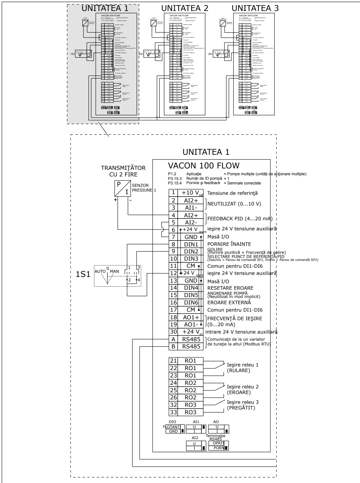
Fig. 18: Diagramă de cablaj electric a sistemului Pompe multiple (acțiune multiplă), exemplul 1A
