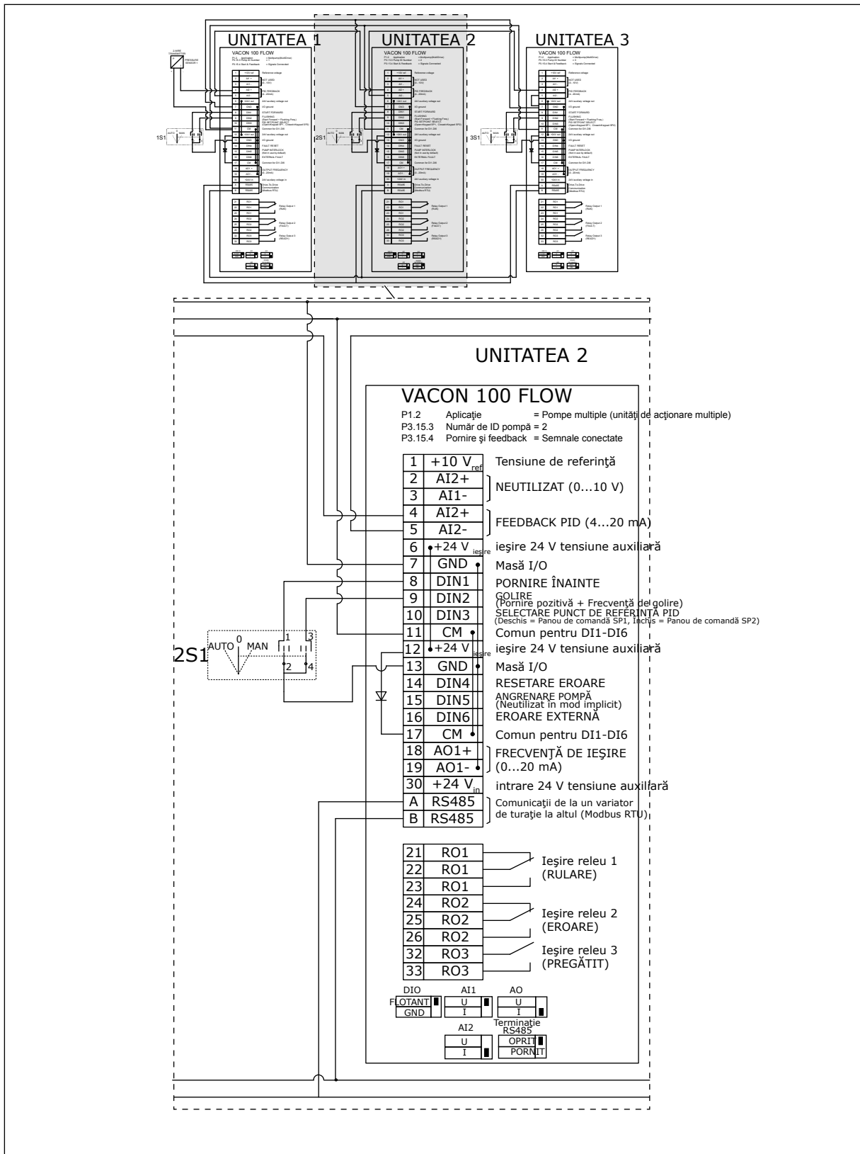
Fig. 22: Diagramă de cablaj electric a sistemului Pompe multiple (acțiune multiplă), exemplul 2B
