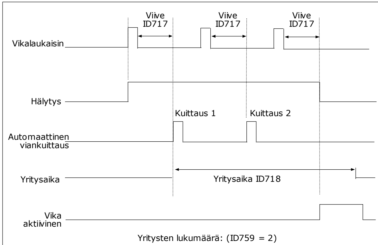
Kuva 72: Automaattinen viankuittaustoiminto
