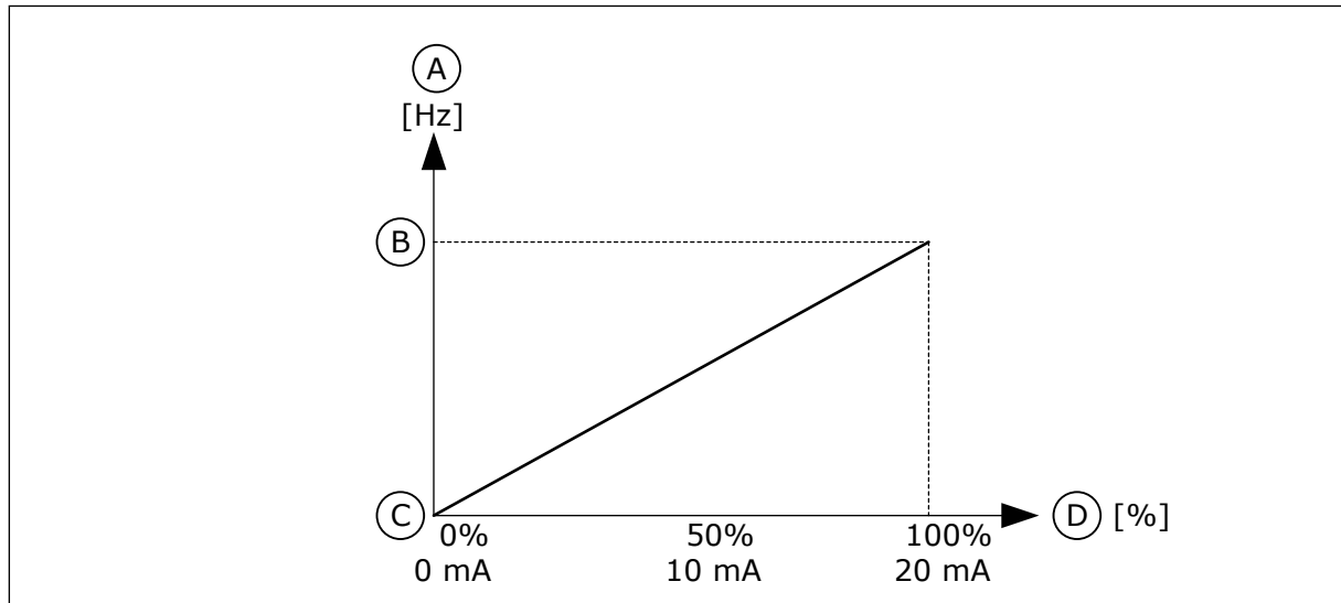
Kuva 57: Analogiatulon signaalialue, valinta 0
