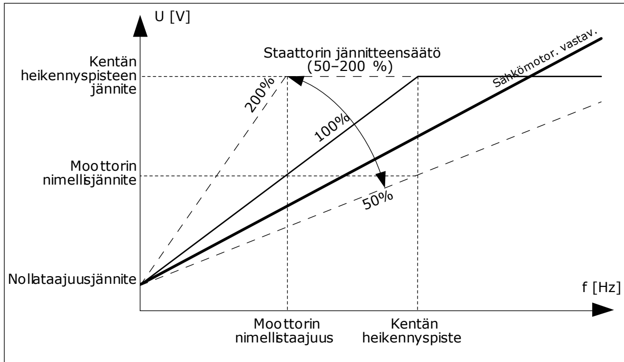
Kuva 37: Staattorin jännitteen säätö
