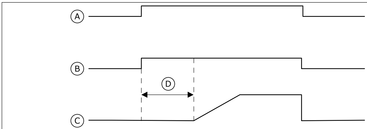
Kuva 106: Siemenvesipumpputoiminto
