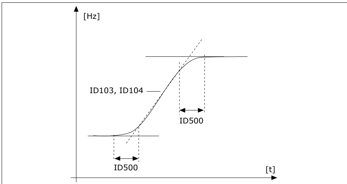
Kuva 49: Kiihdytys-/hidastuskäyrä (S-muoto)
