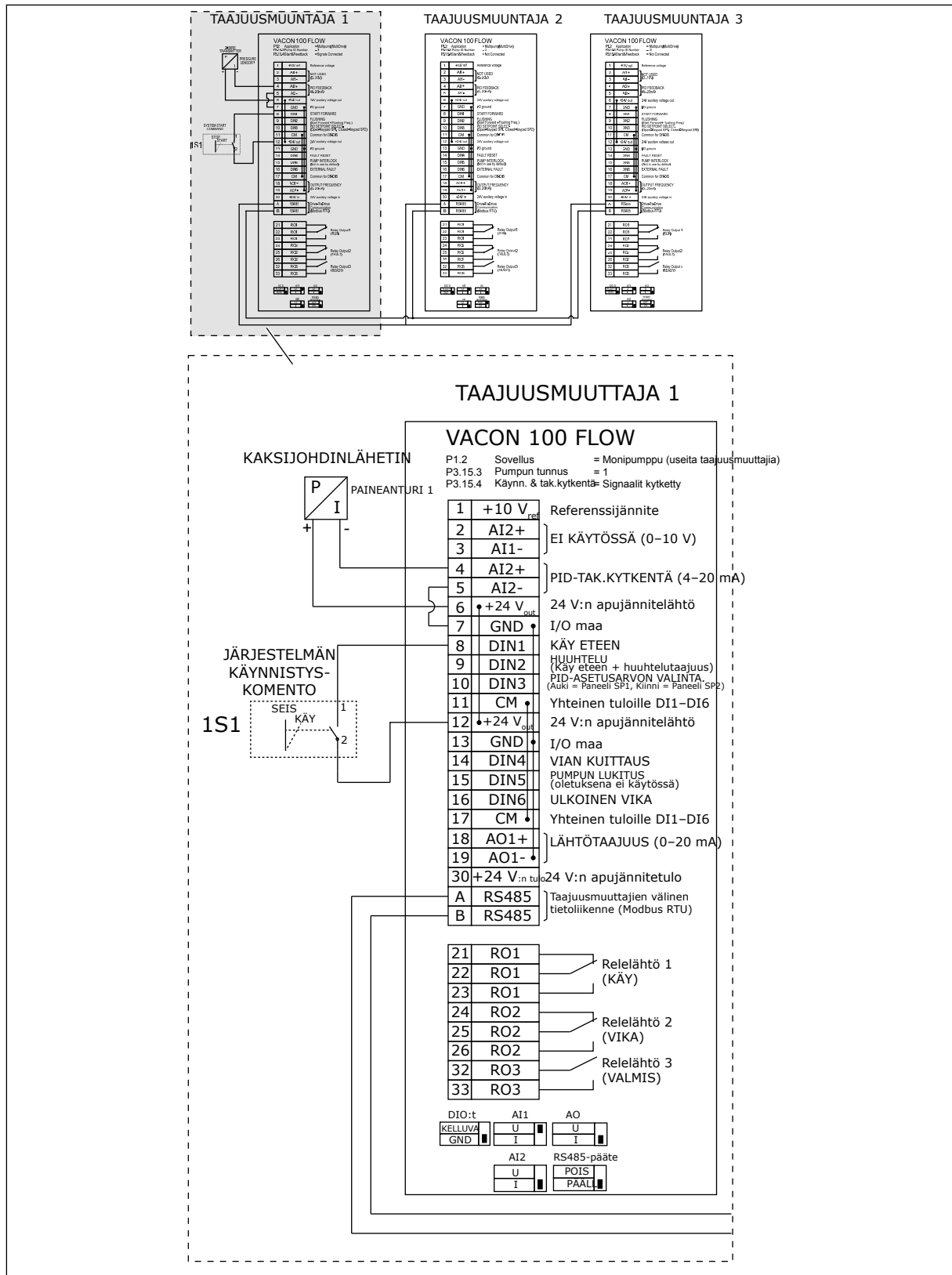
Kuva 30: Usean taaajuusmuuttajan monipumppujärjestelmän kytkentäkaavio, esimerkki 5A
