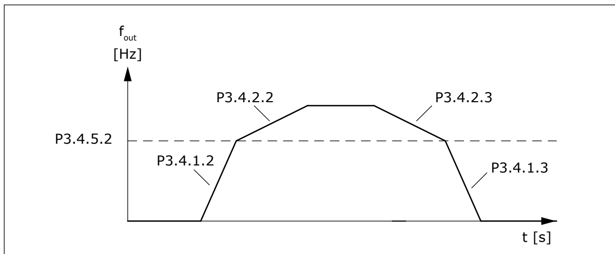
Kuva 50: Rampin 2 aktivointi, kun lähtötaajuus ylittää kynnyсарvon. (P3.4.5.2 = Kiihdyt. 2 taajuusraja, P3.4.1.2 = Kiiht.aika 1, P3.4.2.2 = Kiiht.aika 2, P3.4.1.3 = Hid.aika 1, P3.4.2.3 = Hid.aika 2).
