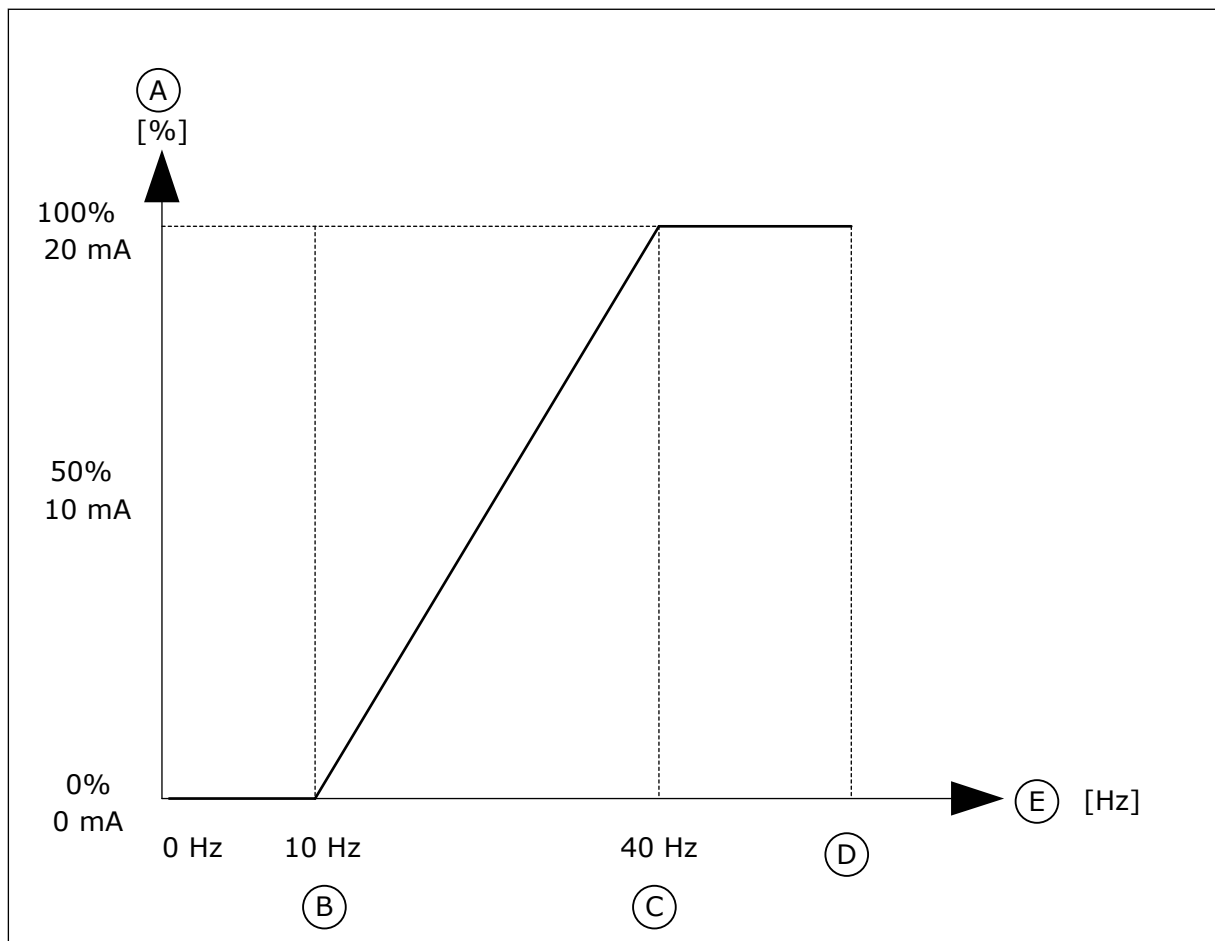
Kuva 62: A01-signaalin skaalaus
