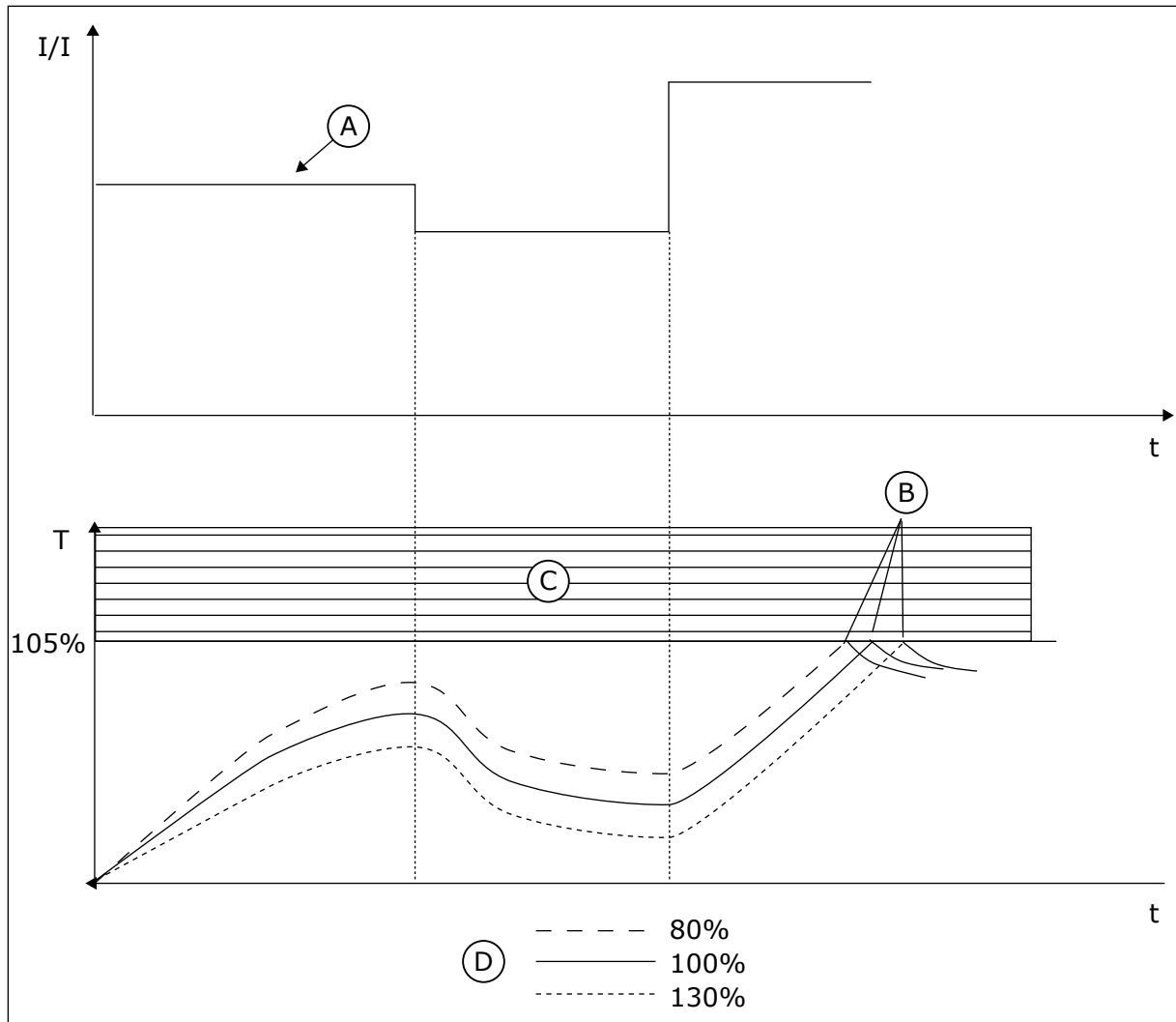
Pav. 67: Variklio temperatūros apskaičiavimas
