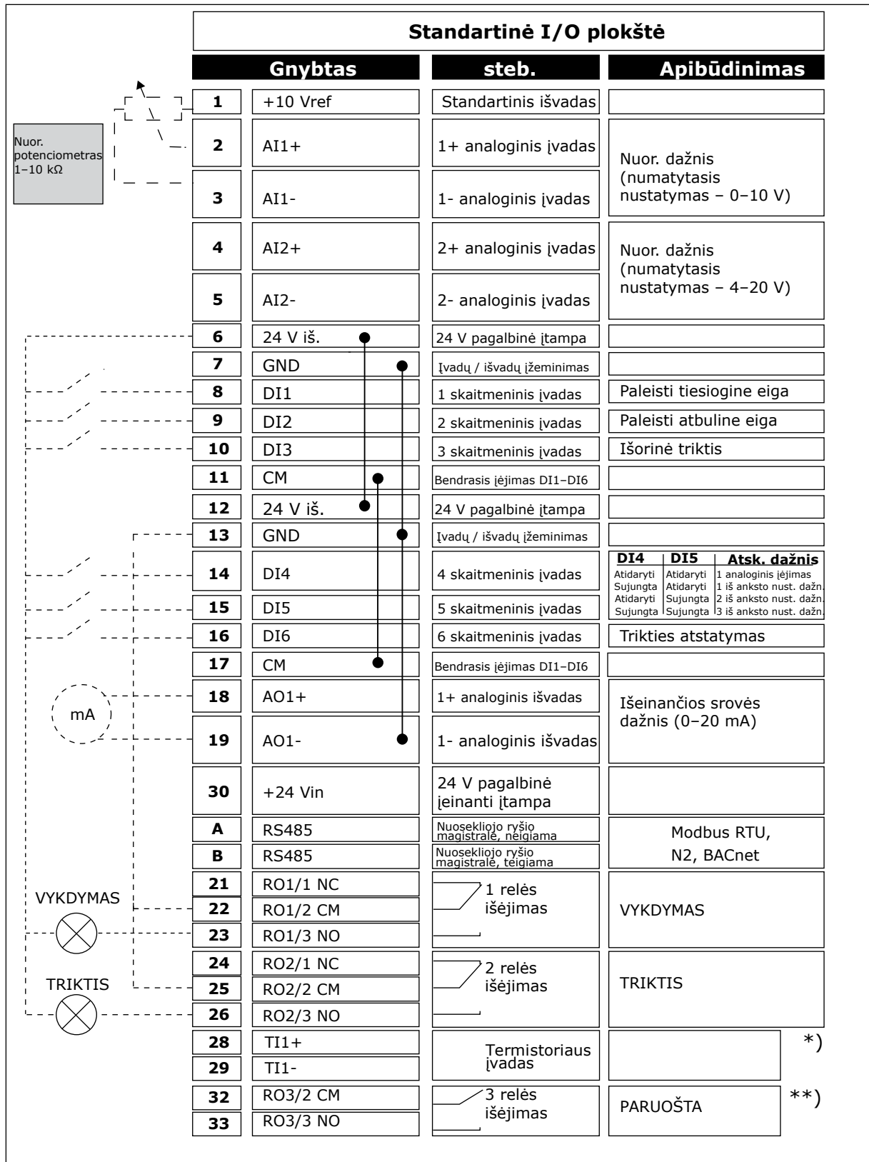
Pav. 4: Standartinės ir ŠVOK (angl. HVAC) programų numatytosios valdymo jungtys
