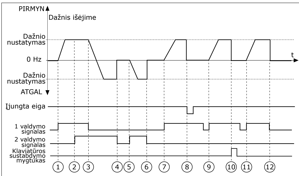
Pav. 44: Įvady / išvady A paleidimo / sustabdymo logika = 2
