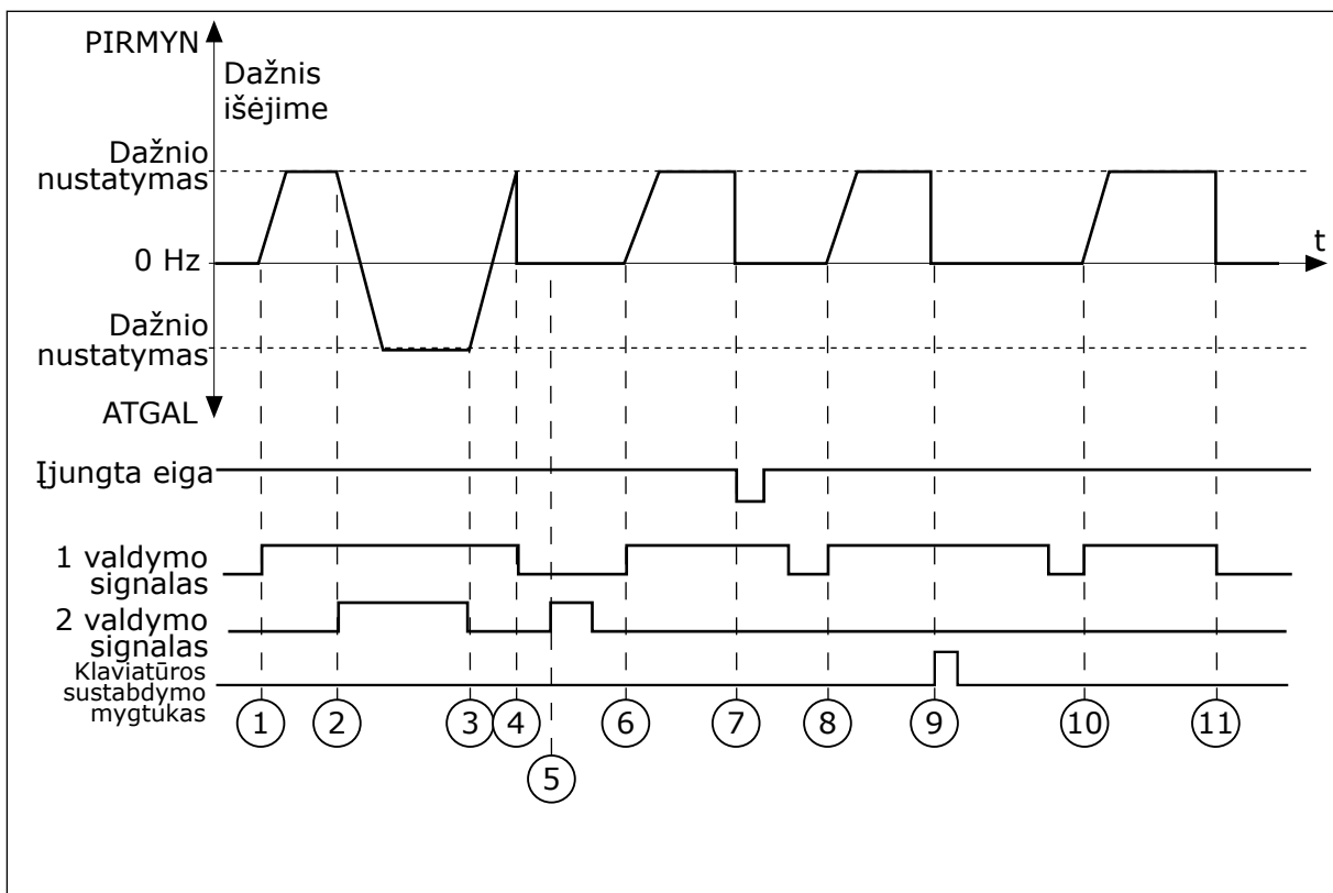
Pav. 46: Įvady / išvady A paleidimo / sustabdymo logika = 4
