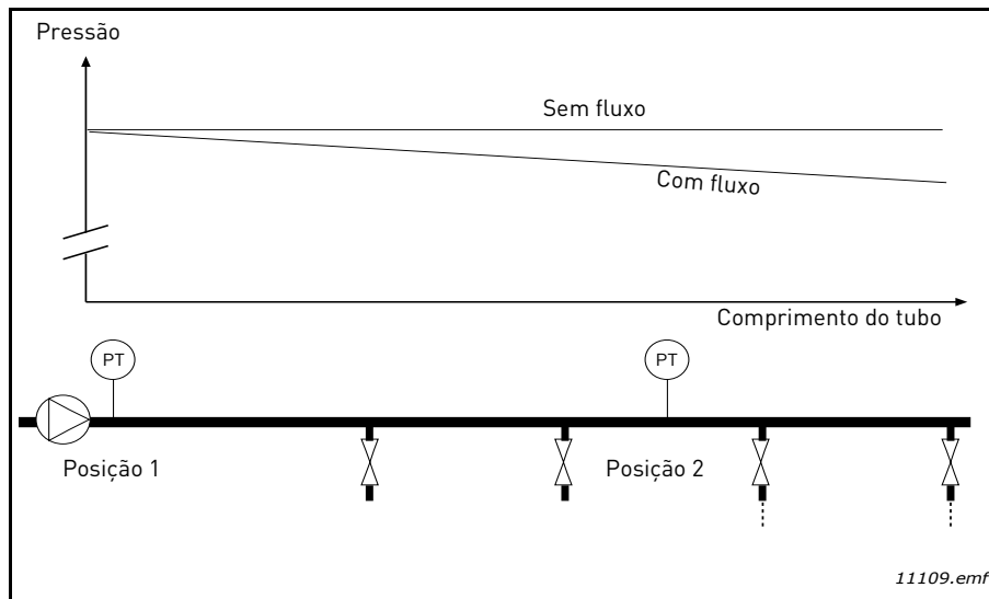
Figura 37. Posição do sensor de pressão
