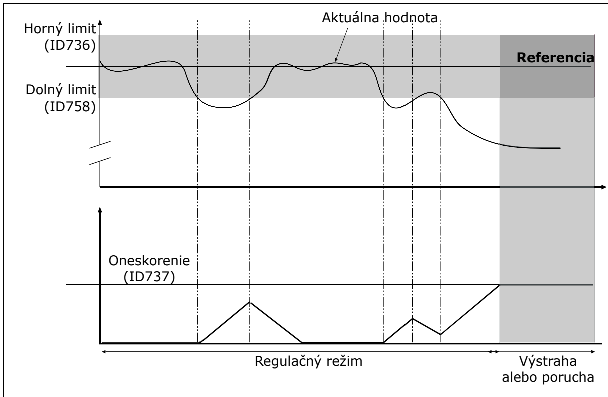
Obr. 41: Funkcia kontroly odozvy
