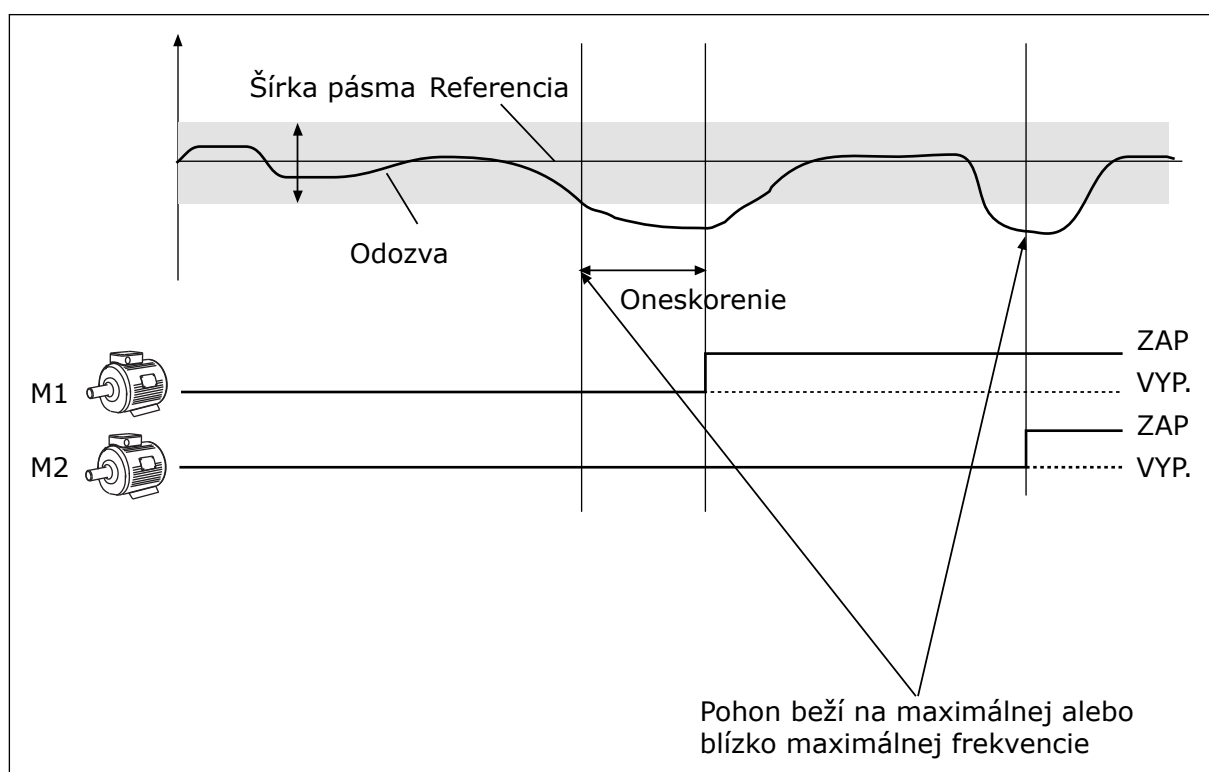
Obr. 44: Funkcia multi-čerpadla
