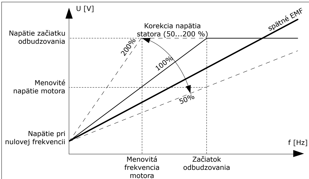
Obr. 14: Korekcia napätia statora
