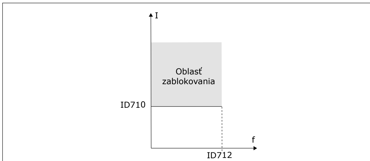
Obr. 30: Nastavenie vlastností zablokovania
