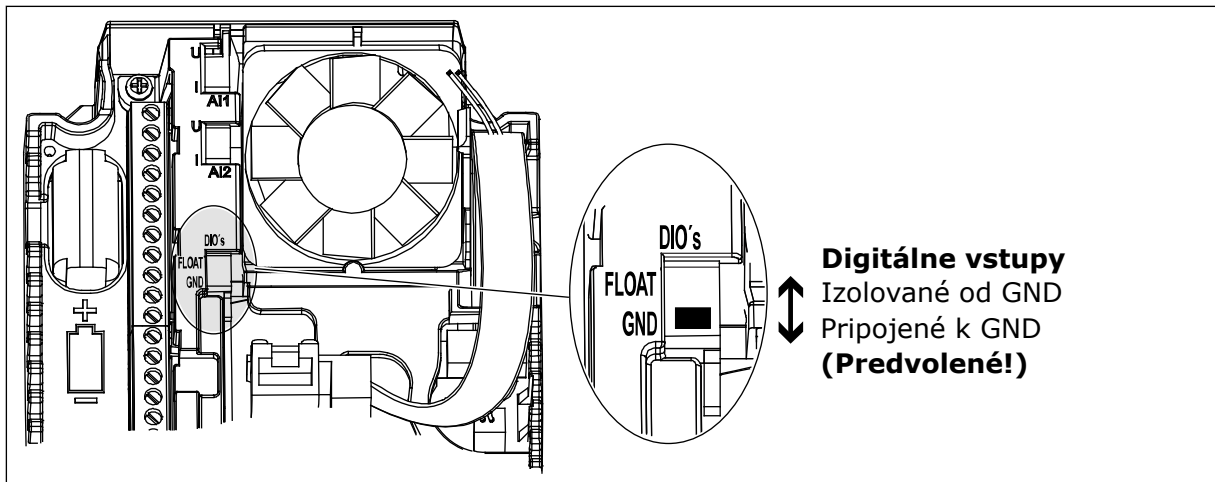
Obr. 7: Prepínač DIP
